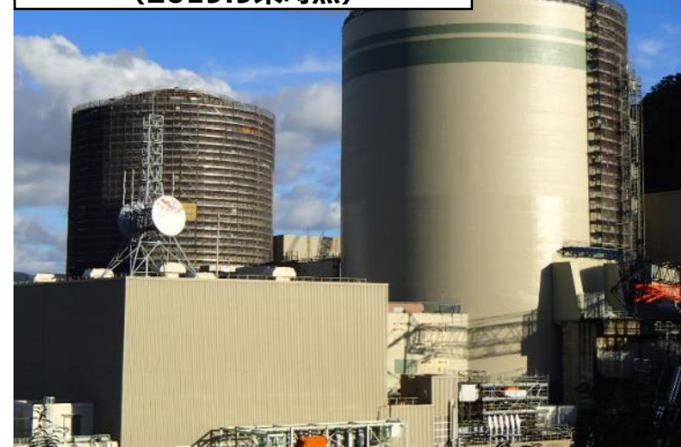
格納容器上部遮蔽設置工事の状況 (2019.9末時点)
