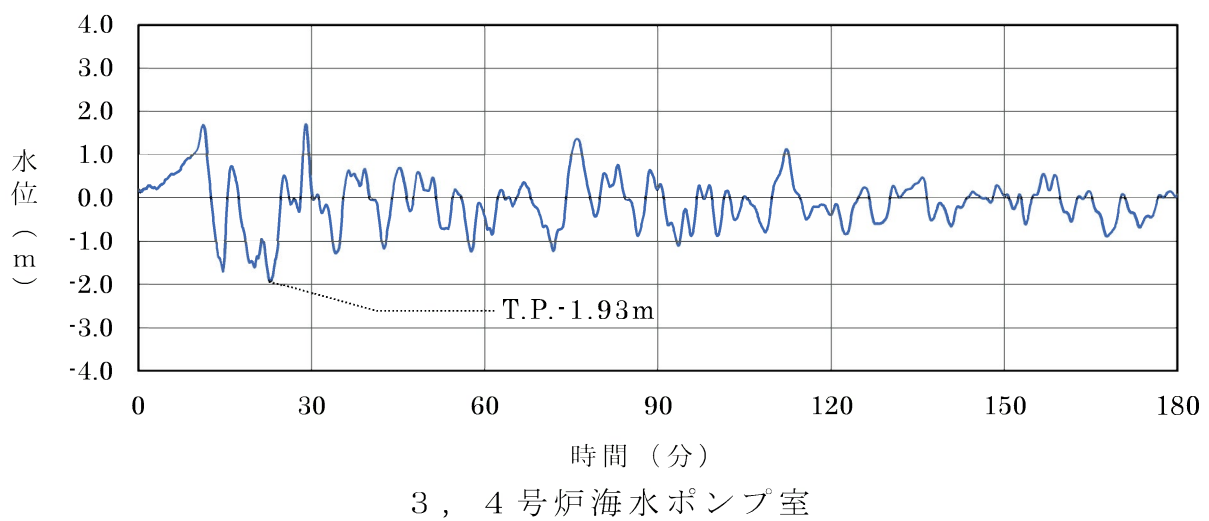
第 1.2.7.3.2 図(4) 基準津波 2 の時刻歴波形 (水位下降側)
