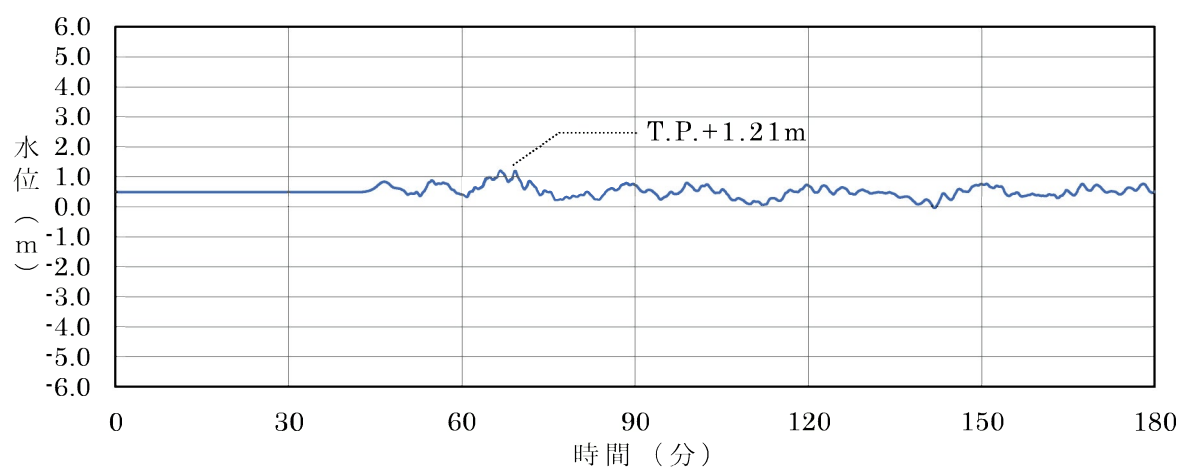
第 1.2.7.3.1 図(1) 基準津波 1 の時刻歴波形 (水位上昇側)
