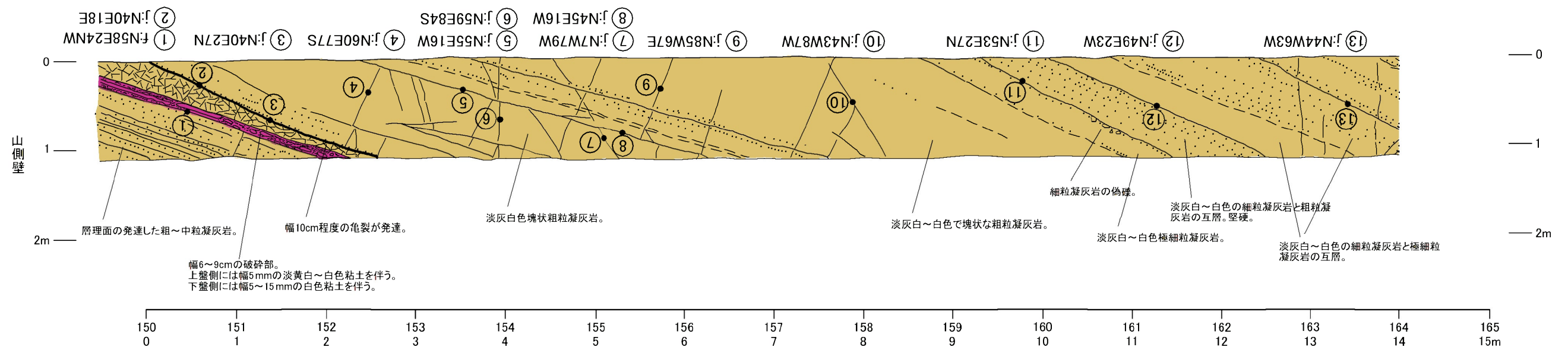
第1.2.3.4.5図(2) 水抜き坑の壁面観察(2)
