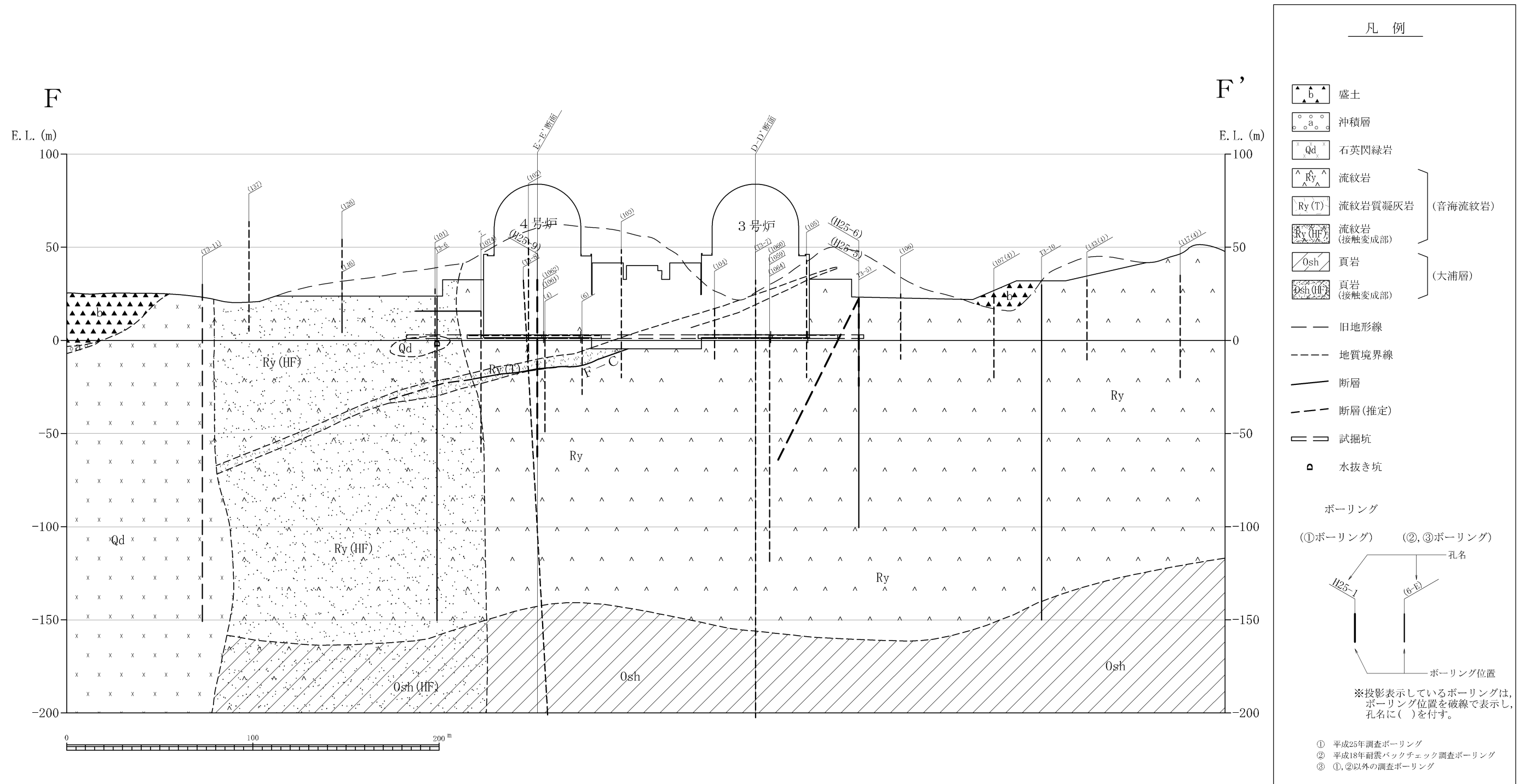
第1.2.3.3.4図(6) 地質鉛直断面図 (F - F' 断面図)
