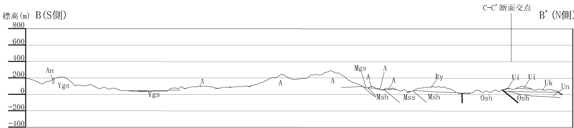
高浜 B-B' 断面
