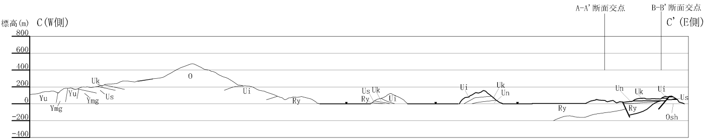
高浜 C-C' 断面
