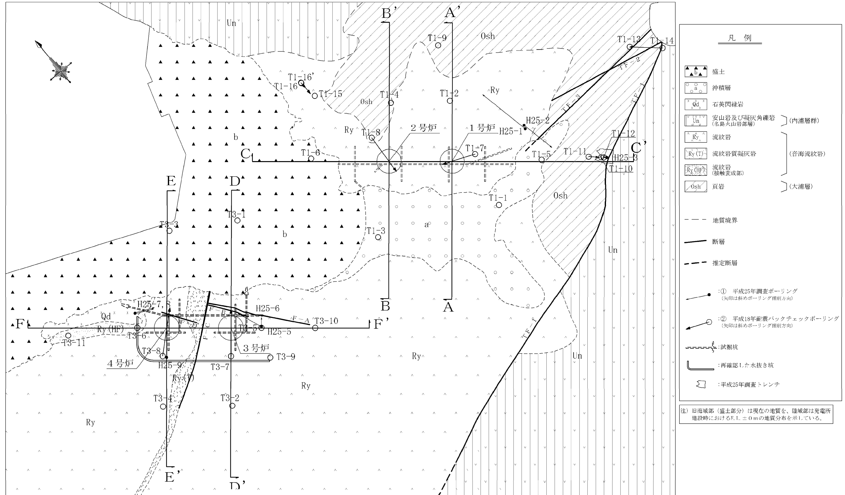
第1.2.3.3.3図 敷地の水平地質断面図 (E.L.±0m)
