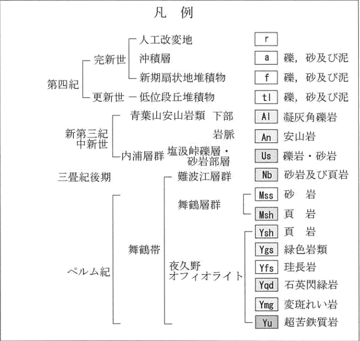
第1.2.3.1.11図 多門院リニアメント周辺の地質図
