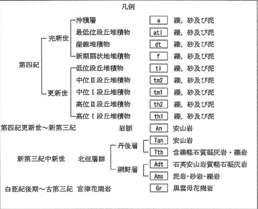
第1.2.3.1.10図 郷村断層周辺の地質図 1.2.3-72
