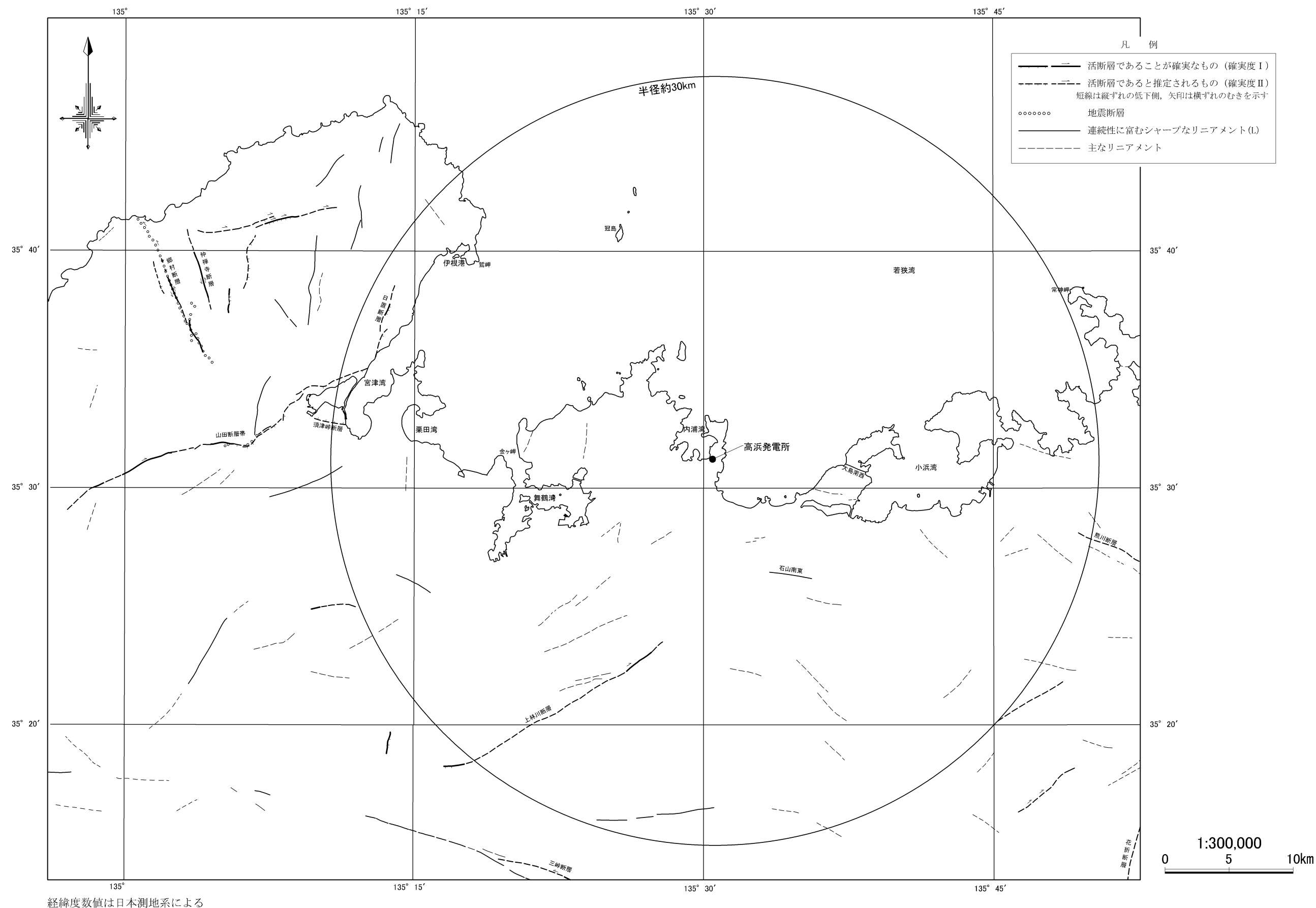
第1.2.3.1.4図 敷地周辺陸域の活断層分布図 「近畿の活断層」
