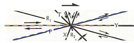
せん断センスを示す複合面構造(狩野・村田、1998 (25) )
