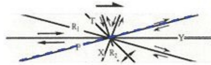
せん断センスを示す複合面構造 (狩野・村田、1998 (25) )
