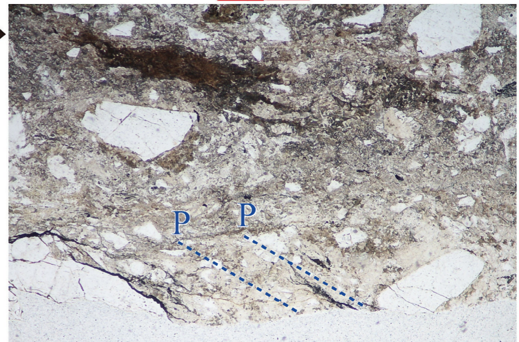
単ニコル
