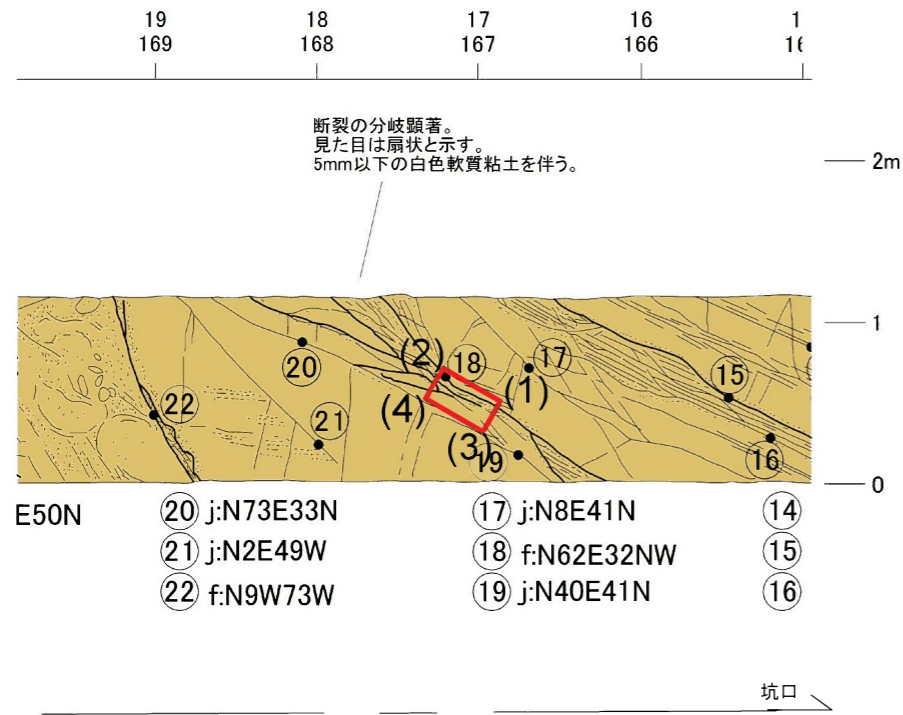
最新面の最大傾斜方向に切った鉛直断面
