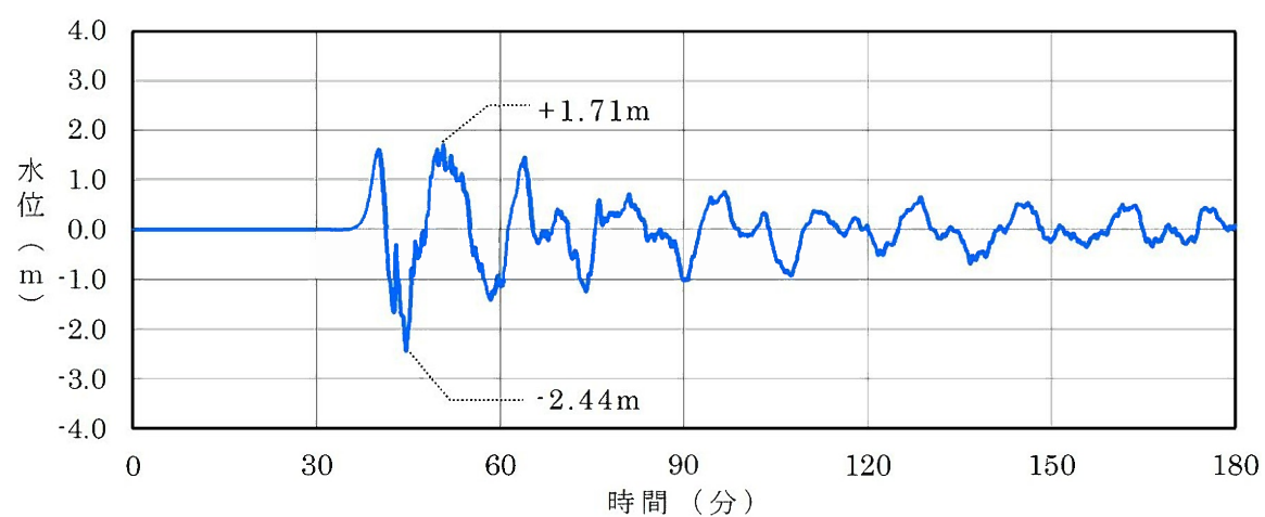
基準津波 1
