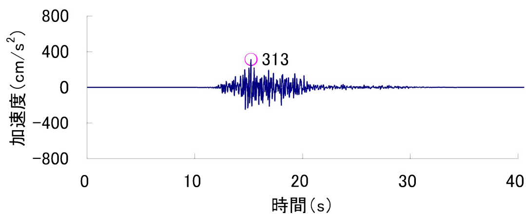
Ss-3 (UD 方向)
