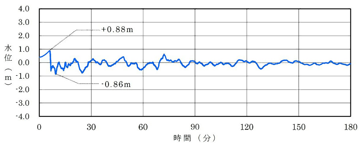
基準津波 2
