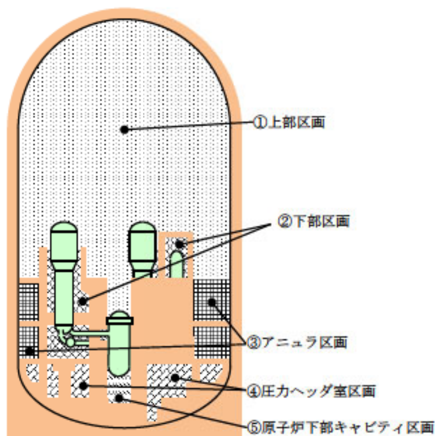
図 3.3-7 MAAP ノード分割図 (原子炉格納容器モデル：3ループプラントの例)
