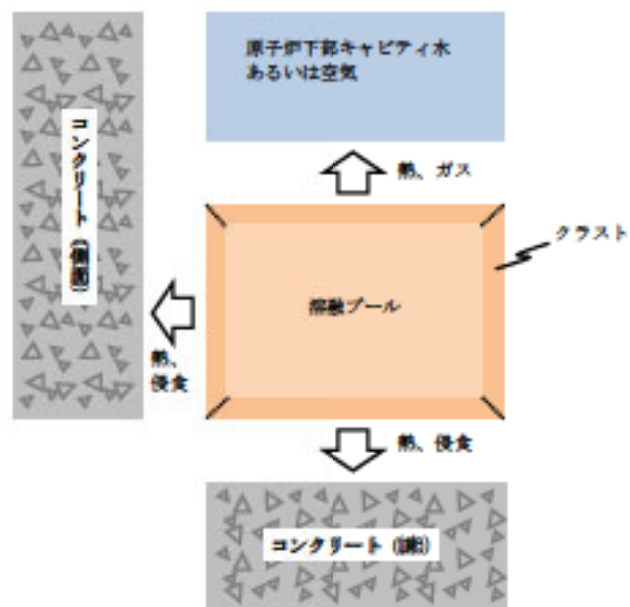
図 3.3-14 熔融炉心の伝熱の概念
