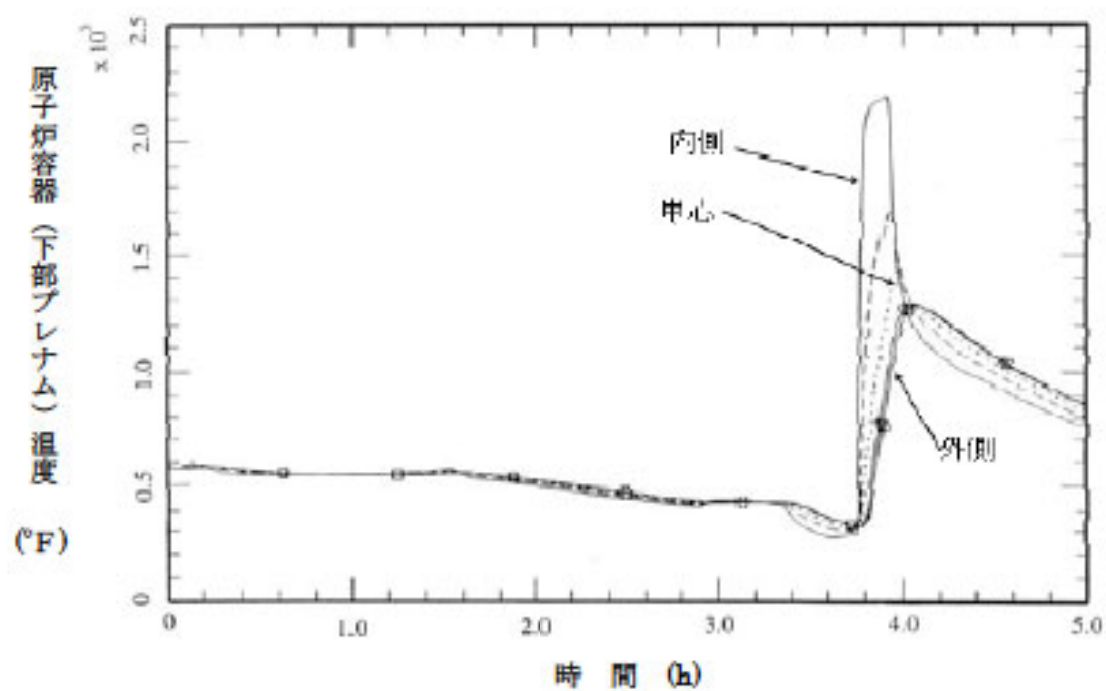
図 4.2-7 TMI 事故のベンチマーク解析結果：原子炉容器下部ヘッド壁温
