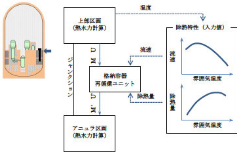
図 3.3-8 格納容器再循環ユニットモデル
