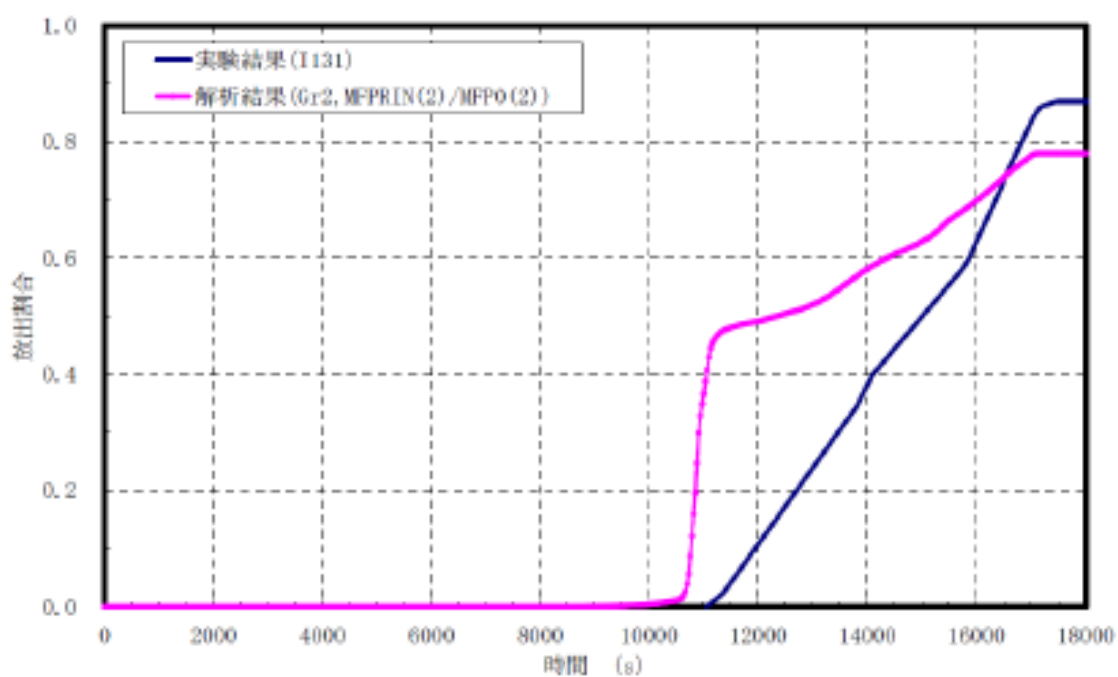
図 4.2-43 よう素放出割合の比較
