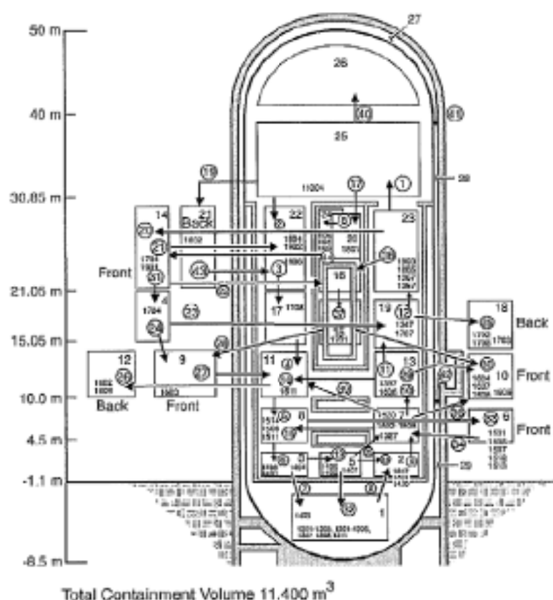
図 4.2-12 ノード分割図 1)
