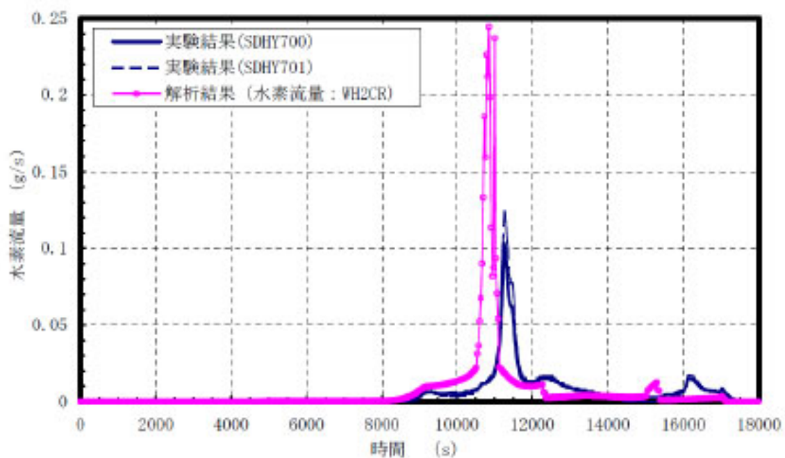
図 4.2-44 1次系での水素流量の比較
