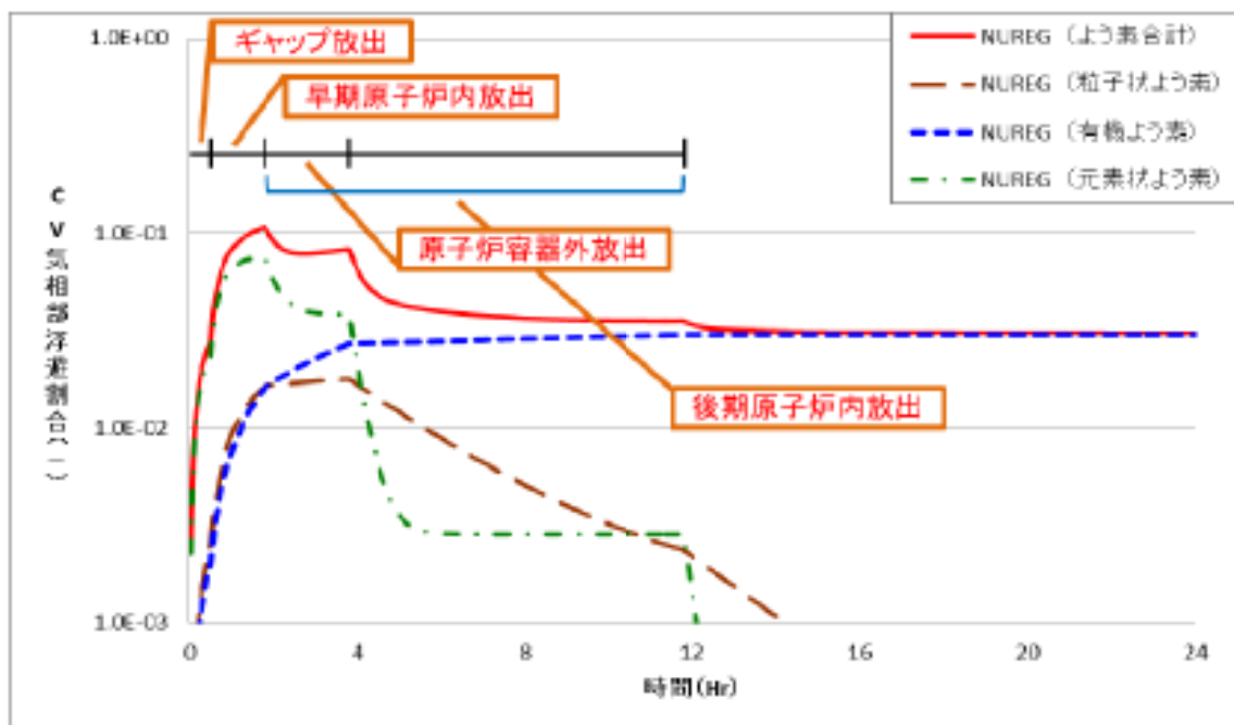
図 3.A-4 原子炉格納容器内気相部浮遊よう素量 (炉心内蓄積量に対する割合：NUREG-1465 ベース)
