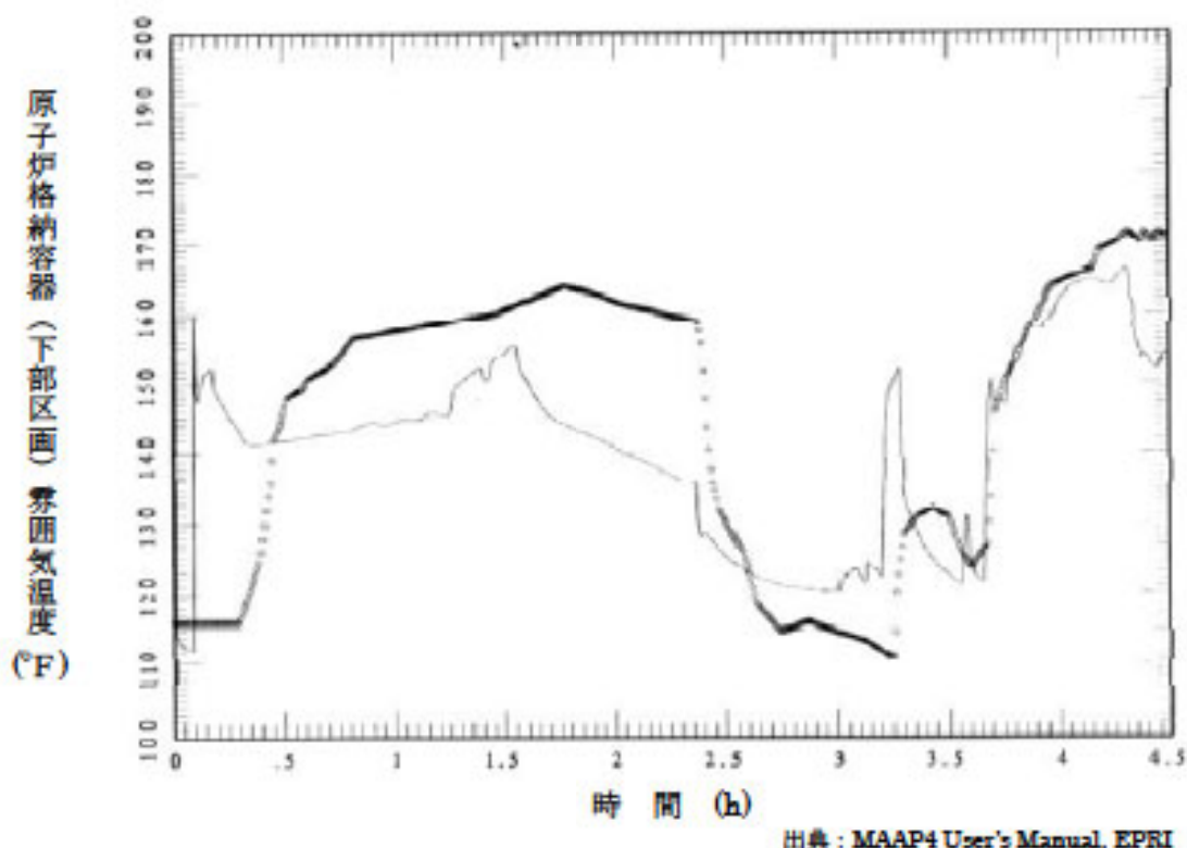
図 4.2-8 TMI 事故のベンチマーク解析結果：原子炉格納容器下部区画雰囲気気温度
