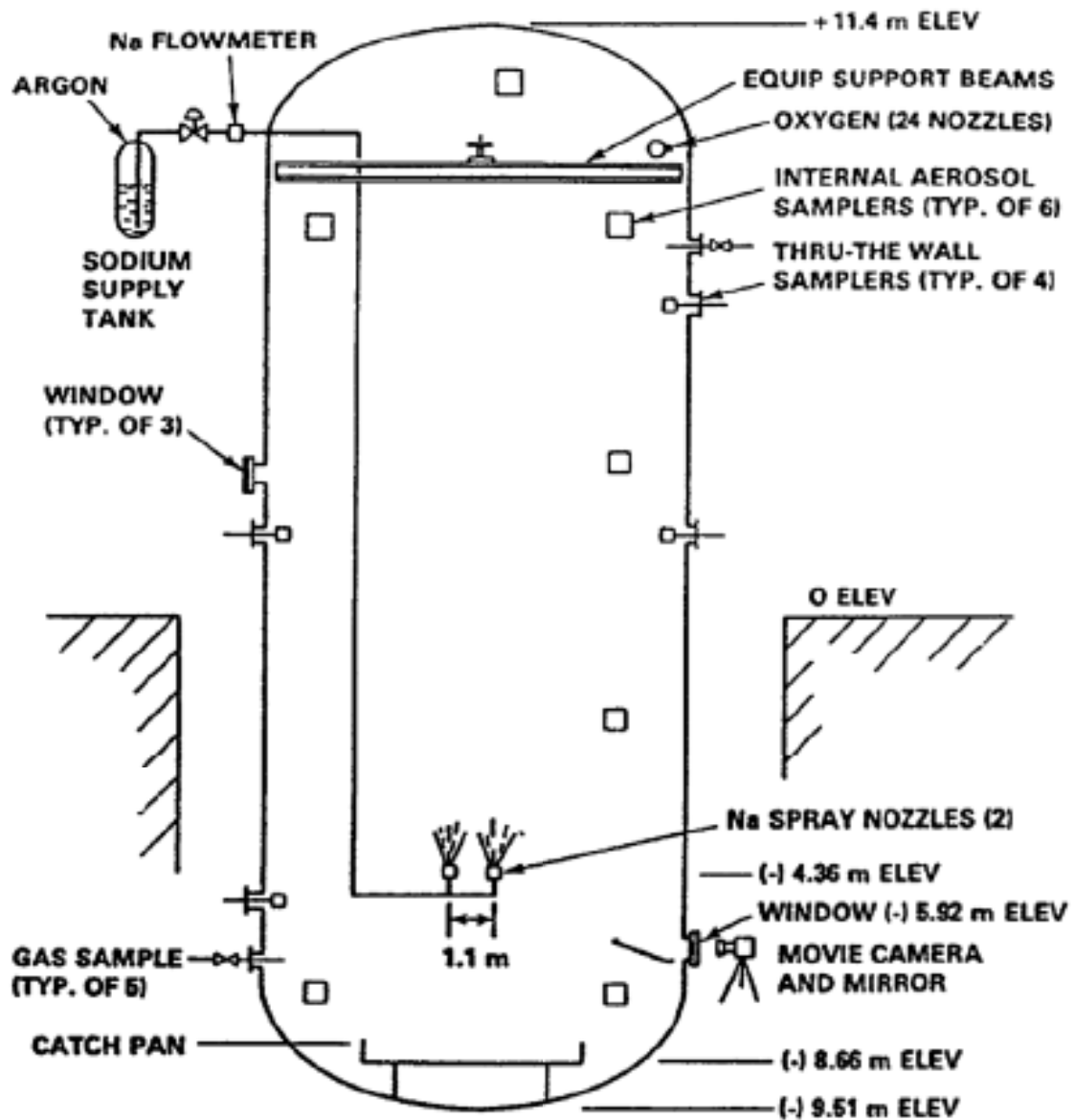
圖 4.2-48 ABCOVE-AB5 試驗裝置
