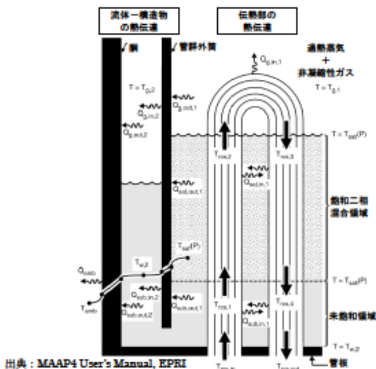
図 3.3-5 MAAP ノード分割図 (2次系モデル)
