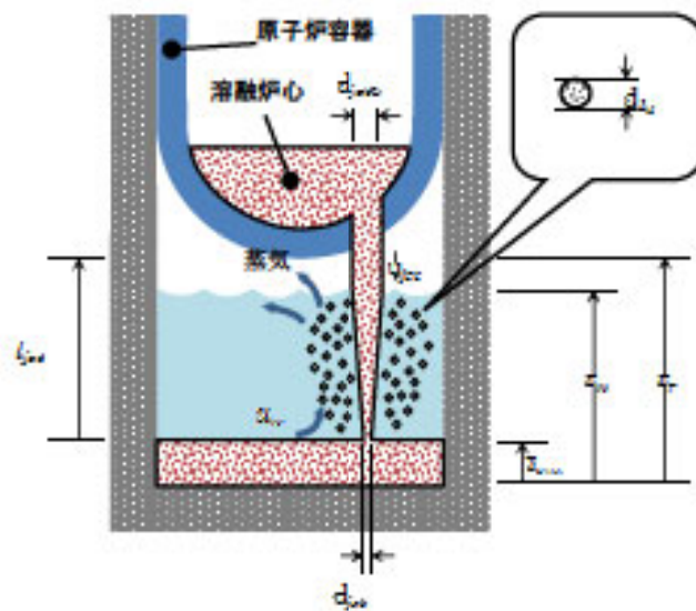
図 3.3-13 原子炉下部キャビティにおける熔融炉心挙動の概念
