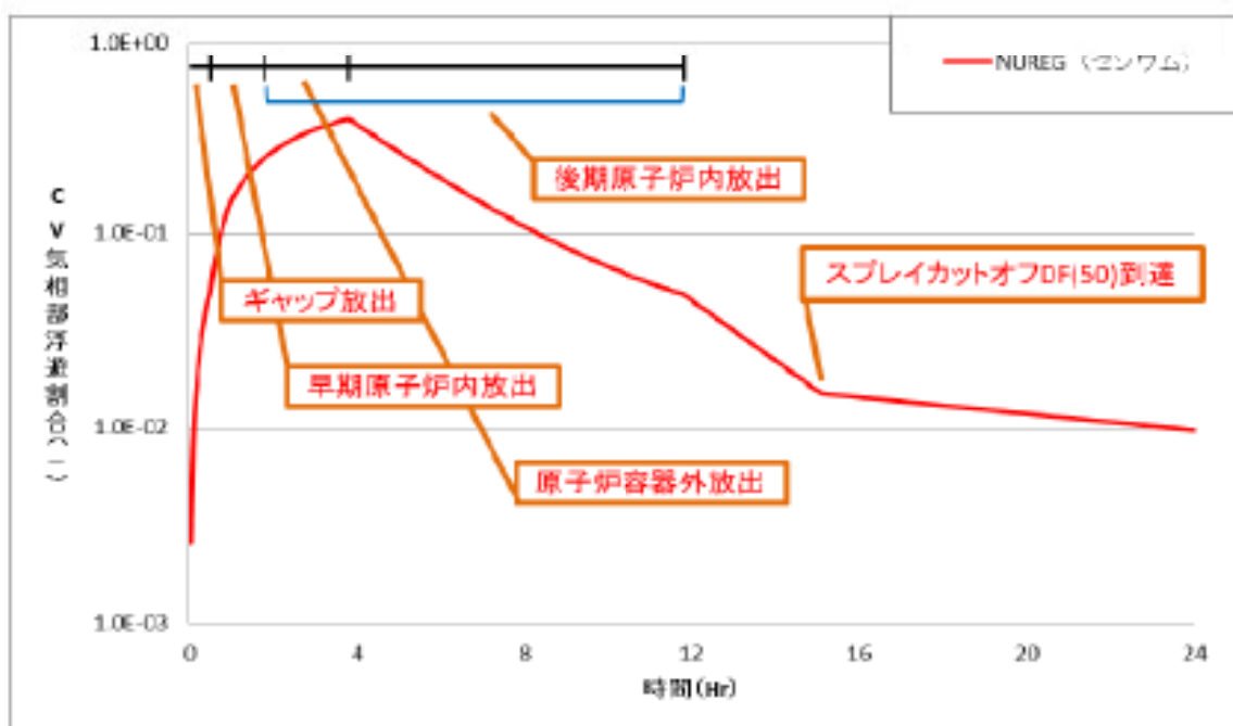
図 3.A-6 原子炉格納容器内気相部浮遊 Cs 量 (炉心内蓄積量に対する割合 : NUREG-1465 ベース)
