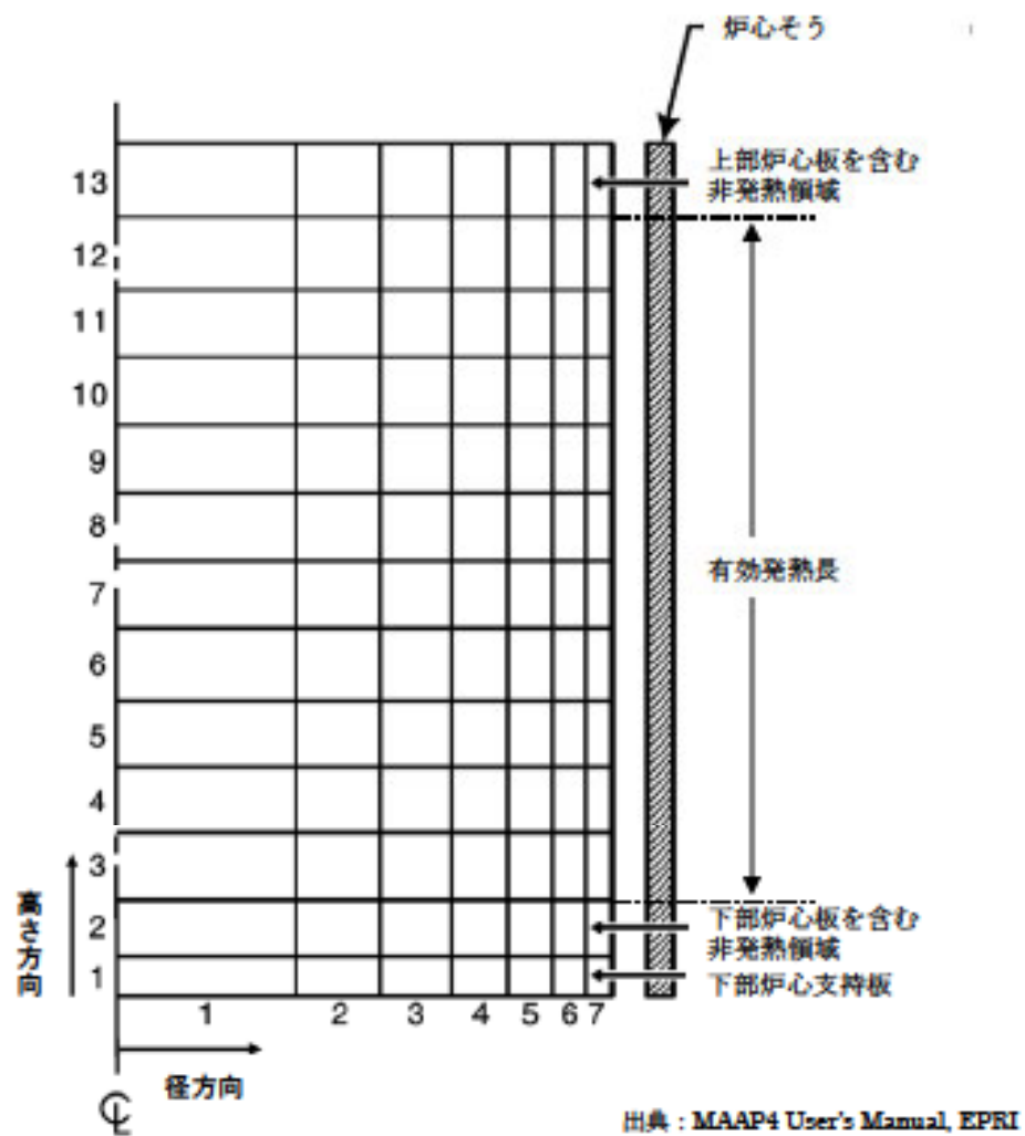
図 3.3-1 MAAP ノード分割例 (炉心モデル)
