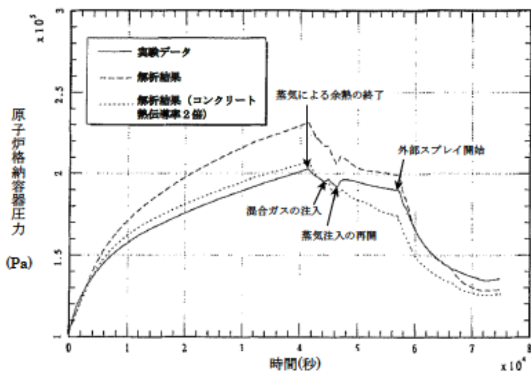
図 4.2-13 HDR 実験のベンチマーク解析結果：原子炉格納容器圧力 1)
