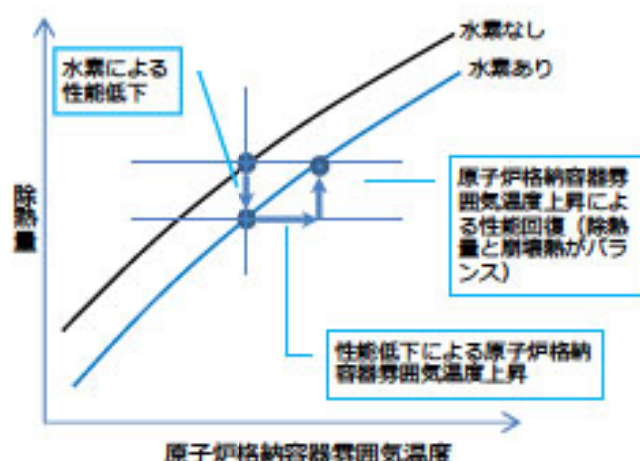
格納容器再循環ユニット除熱特性 概念図
