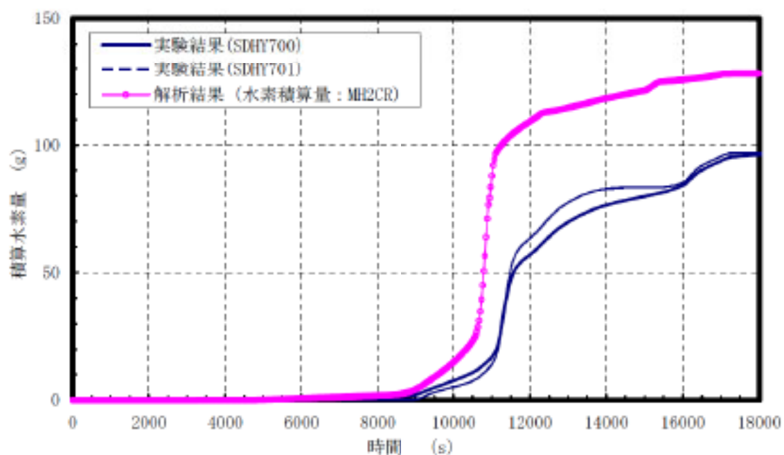
図 4.2-45 水素積算量
