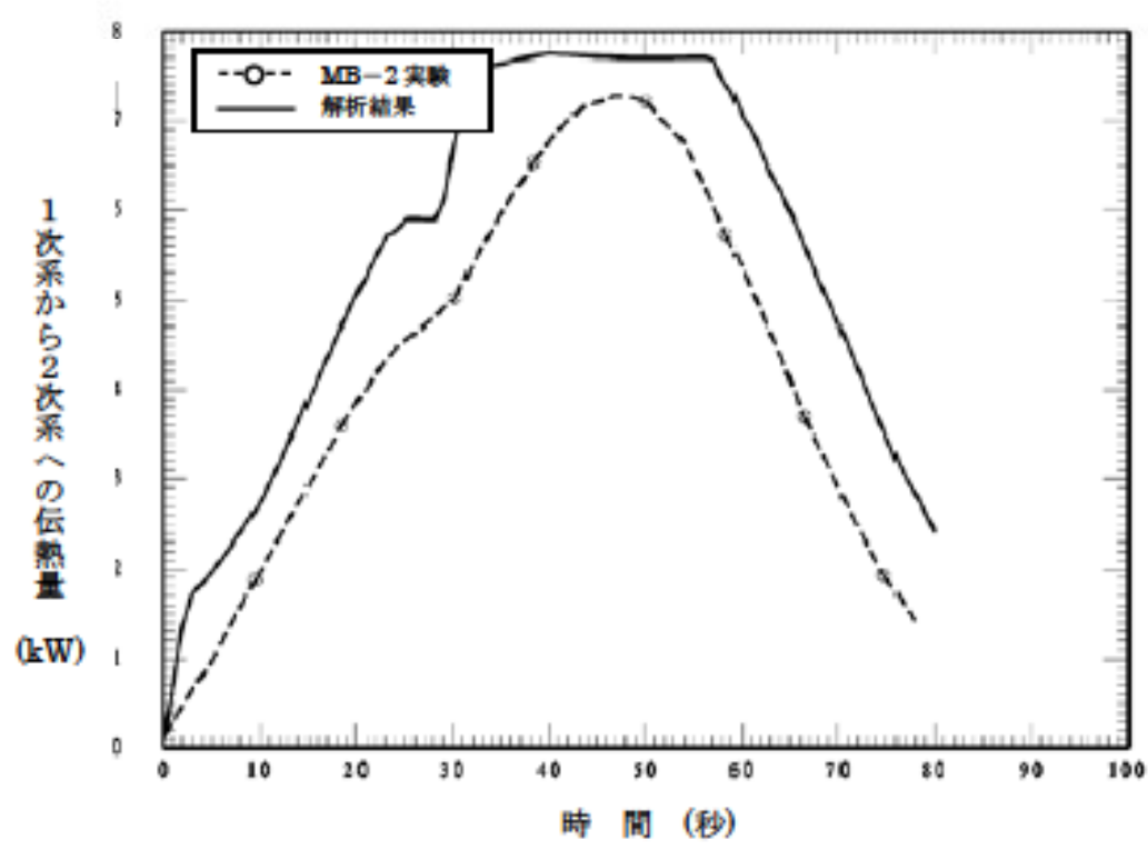
図 4.2-30 MB-2 実験ベンチマーク解析結果 (100%主蒸気管破断) (2/2)
