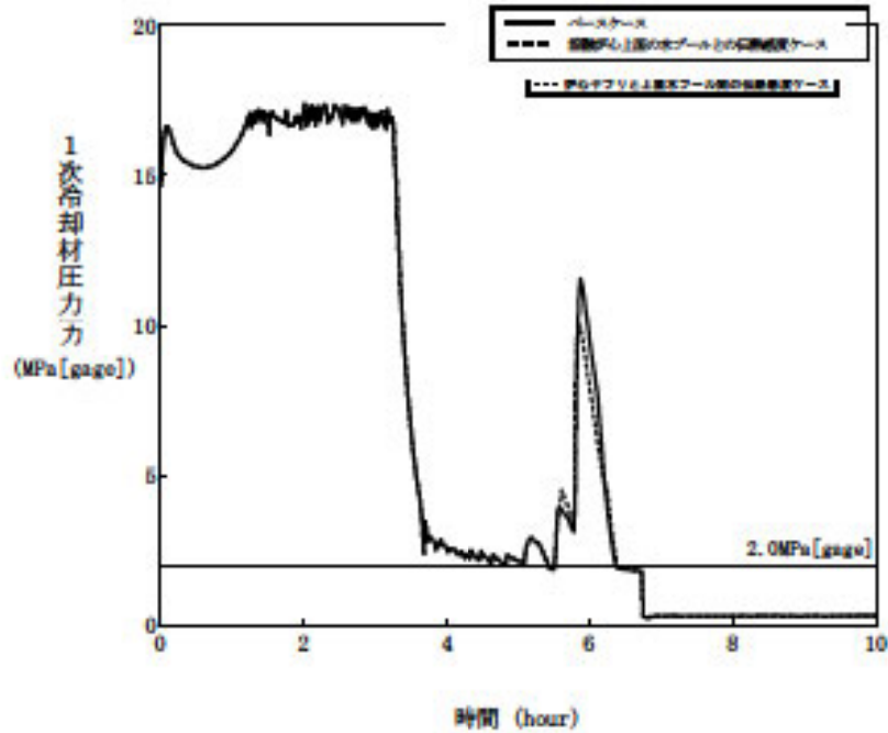
図 4.3-18 下部プレナムでの溶融炉心の熱伝達に関する感度解析結果 (溶融炉心上面の水プールとの伝熱)
