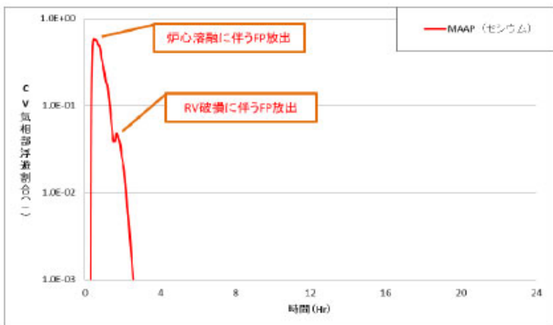
図 3.A-5 原子炉格納容器内気相部浮遊 Cs 量 (炉心内蓄積量に対する割合 : MAAP ベース (補正))
