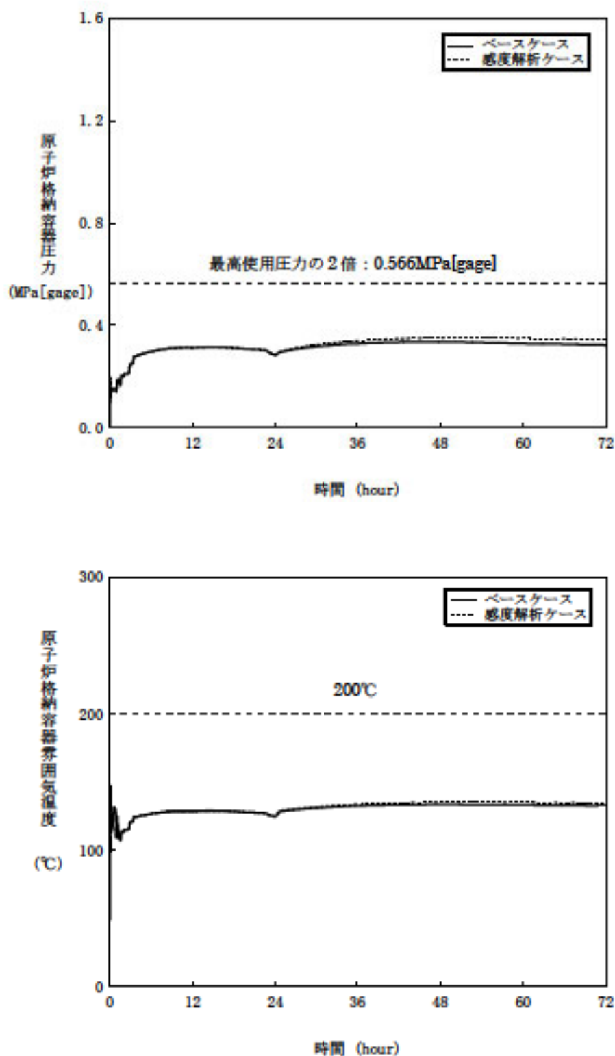
図 4.3-10 再循環ユニット自然対流冷却モデルに関する感度解析結果
