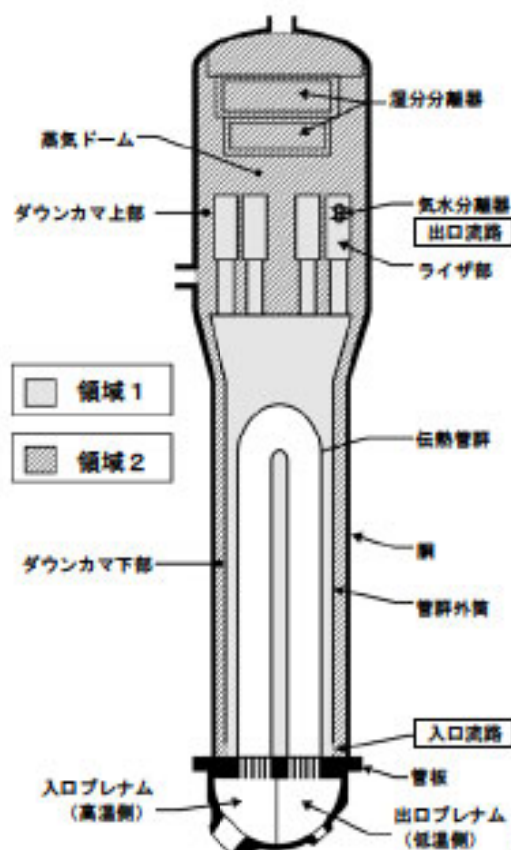
図 3.3-5 MAAP ノード分割図 (2次系モデル)
