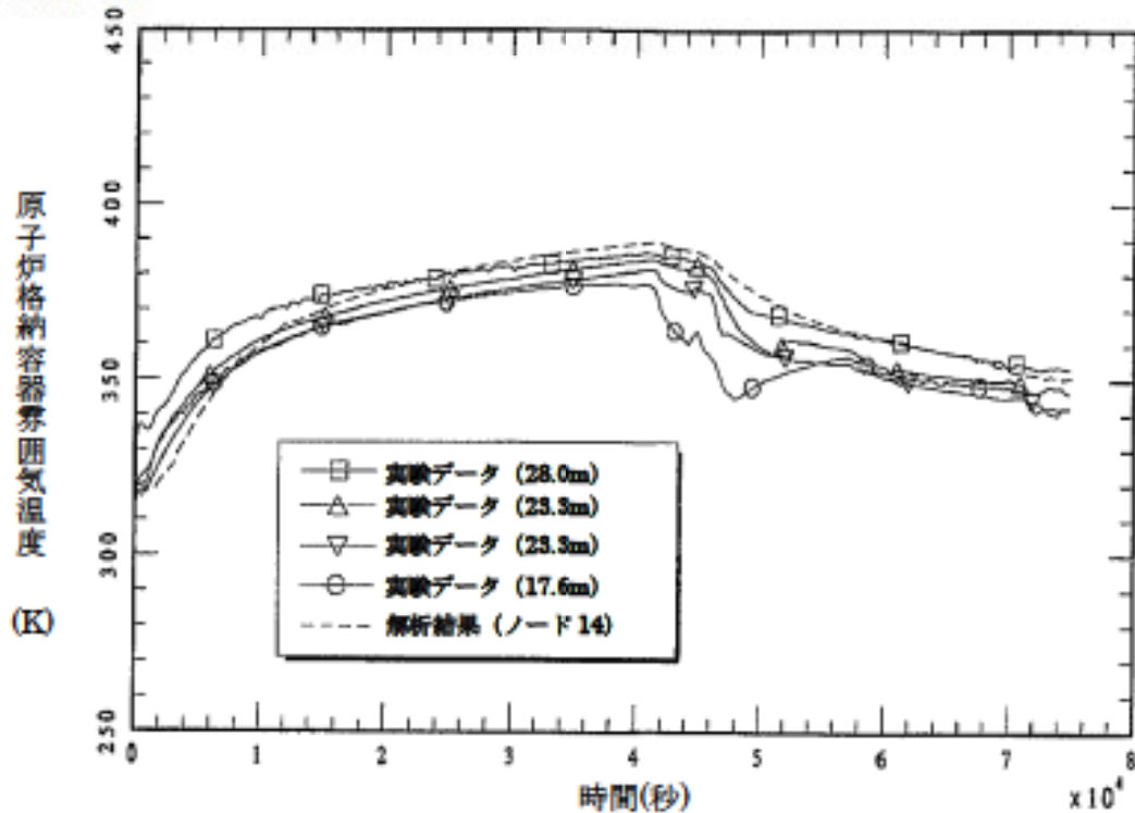
図 4.2-14 HDR 実験のベンチマーク解析結果：原子炉格納容器雰囲気温度 [K]
