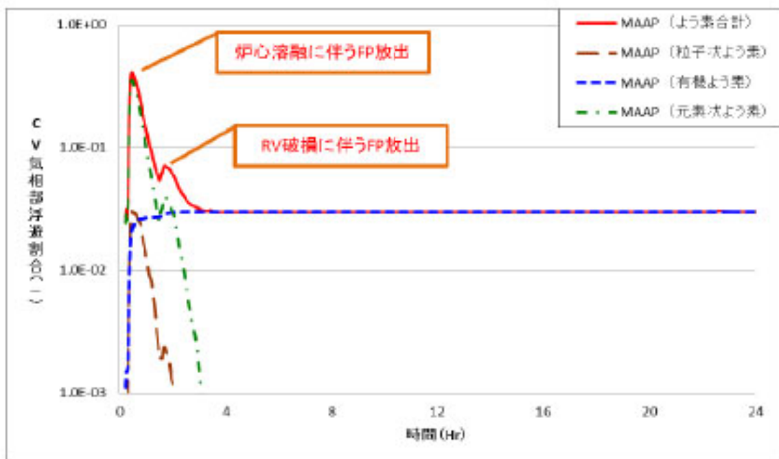
図 3.A-3 原子炉格納容器内気相部浮遊よう素量 (炉心内蓄積量に対する割合：MAAPベース (補正))
