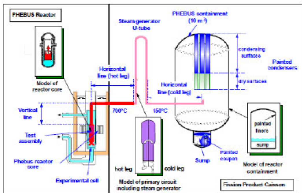
图 4.2-32 PHEBUS-FP 实验设备概要
