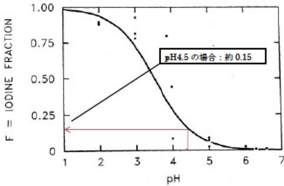
図 3.A-7 ヨウ化イオン(I - )とヨウ素(I 2 )の割合
