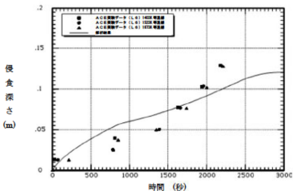
図 4.2-26 ACE 実験ベンチマーク解析結果 (ケース L6)
