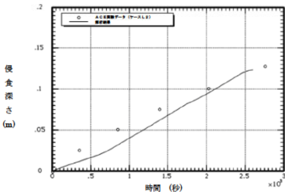
図 4.2-25 ACE 実験ベンチマーク解析結果 (ケース L2)
