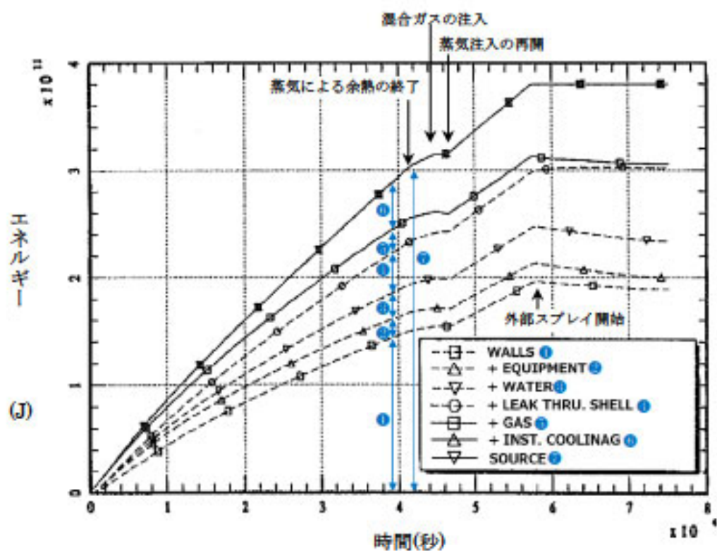
図 4.2-16 HDR 実験のベンチマーク解析結果：エネルギーバランス (MAAP) 1)
