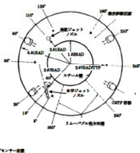
図 4.2-17 CSTF 実験装置の区画構成 (全体)
