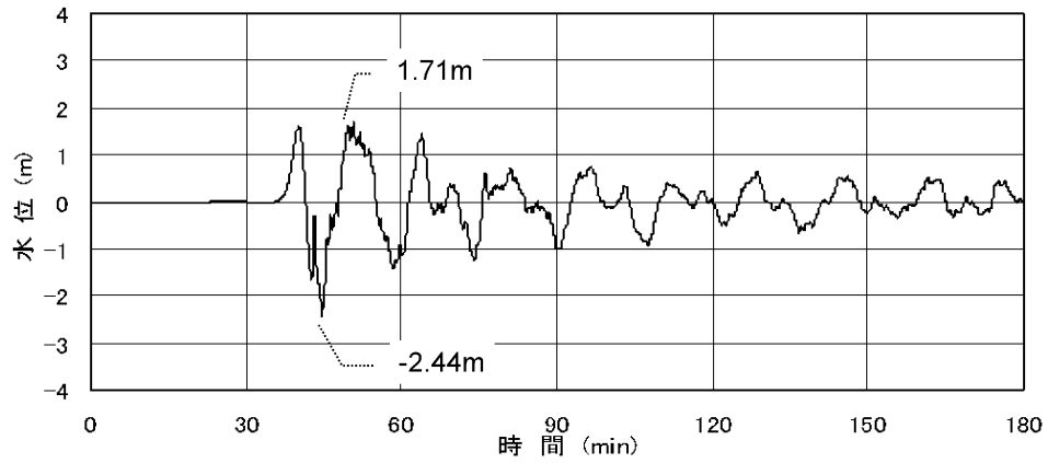
基準津波 1 若狭海丘列付近断層と隠岐トラフ海底地すべりを波源とする時刻歴波形
