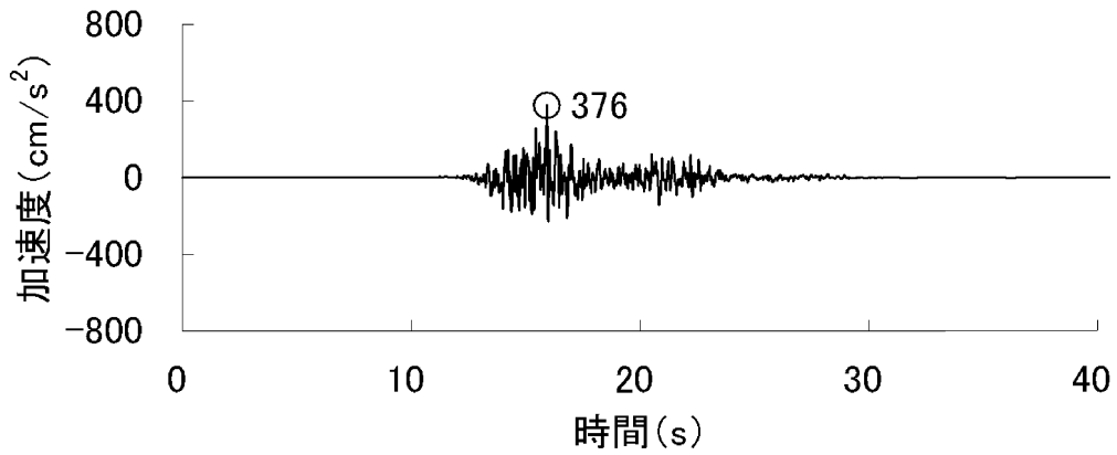
加速度 (水平方向 : Ss-2 H (NS))
