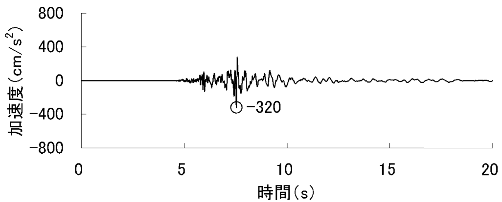
加速度（鉛直方向：Ss-7 V ）
