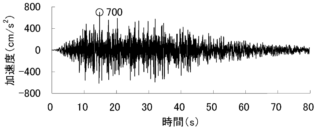
加速度 (水平方向 : Ss-1 H )
