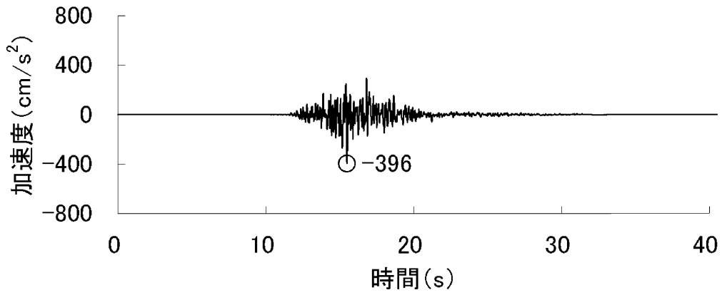
加速度（水平方向：Ss-3 H (NS)）
