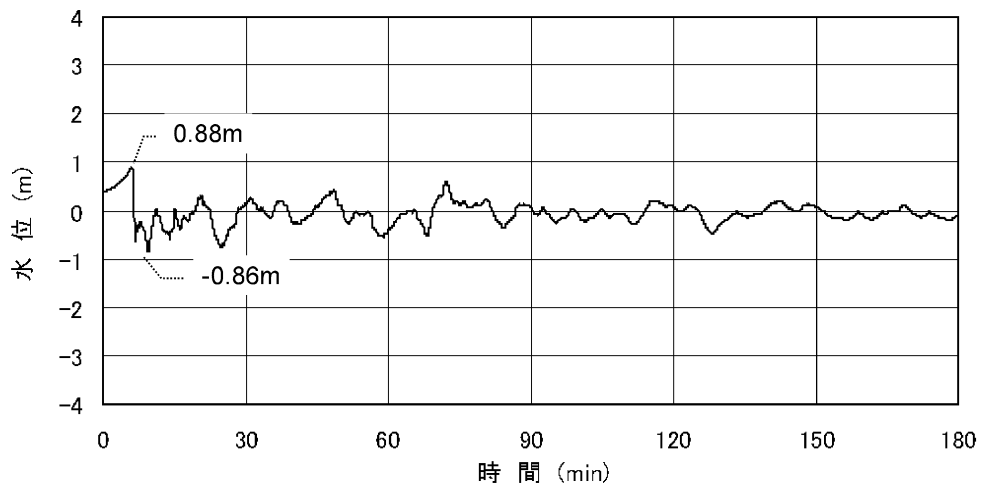
基準津波 2 F O - A ~ F O - B ~ 熊川断層と陸上地すべりを波源とする時刻歴波形
