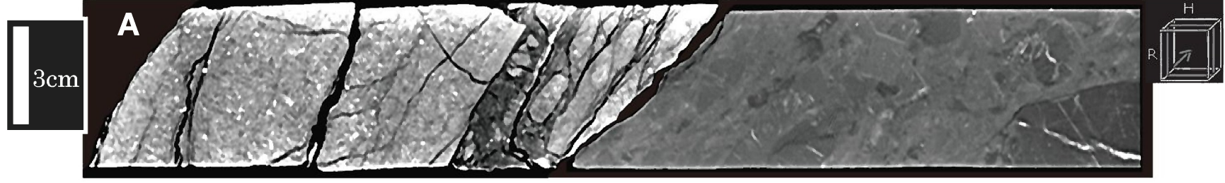
第1.2.3.3.8図 大浦層と音海流紋岩の境界部のボーリング調査結果 (T1-7孔)
