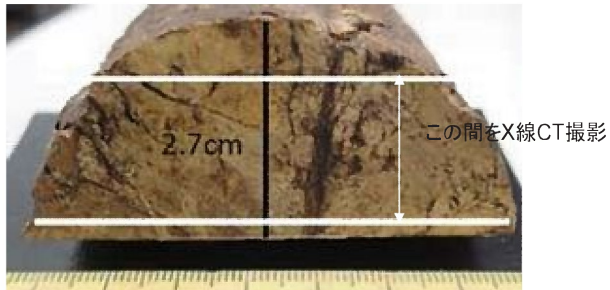
第1.2.3.3.10図(2) 音海流紋岩と内浦層群の境界部のボーリング調査結果 (T1-16' 孔)
