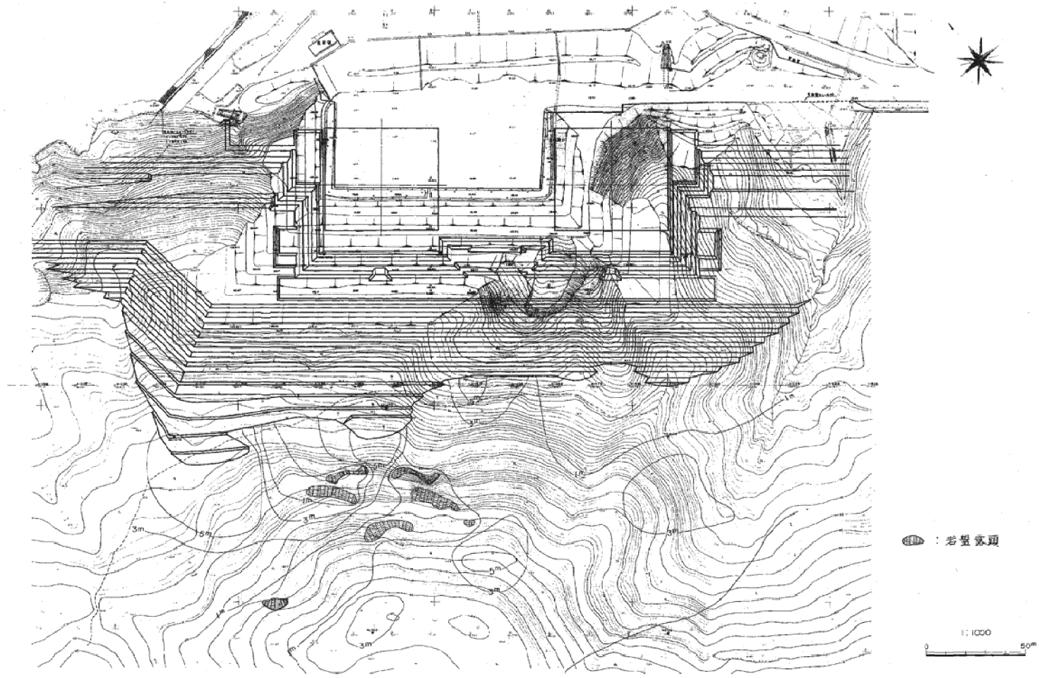
第1.2.3.4.4図 原子炉設置位置背後山地の表層土の厚さ分布図
