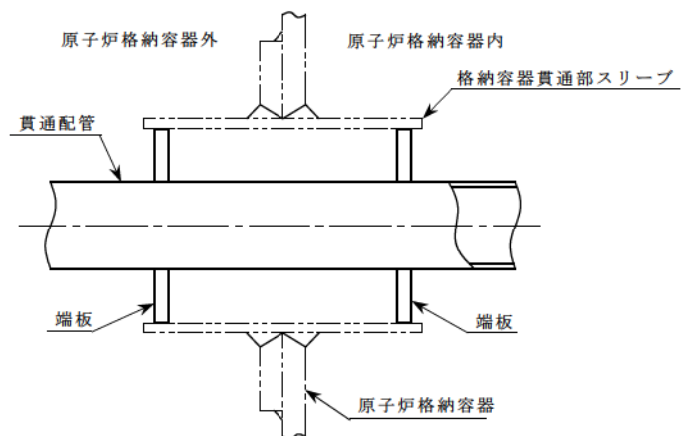
固定式配管貫通部
