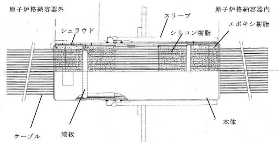
電線貫通部（キャニスター型）
