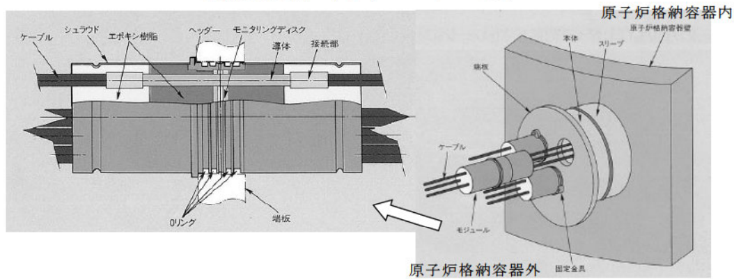
電線貫通部（キャニスター型）
