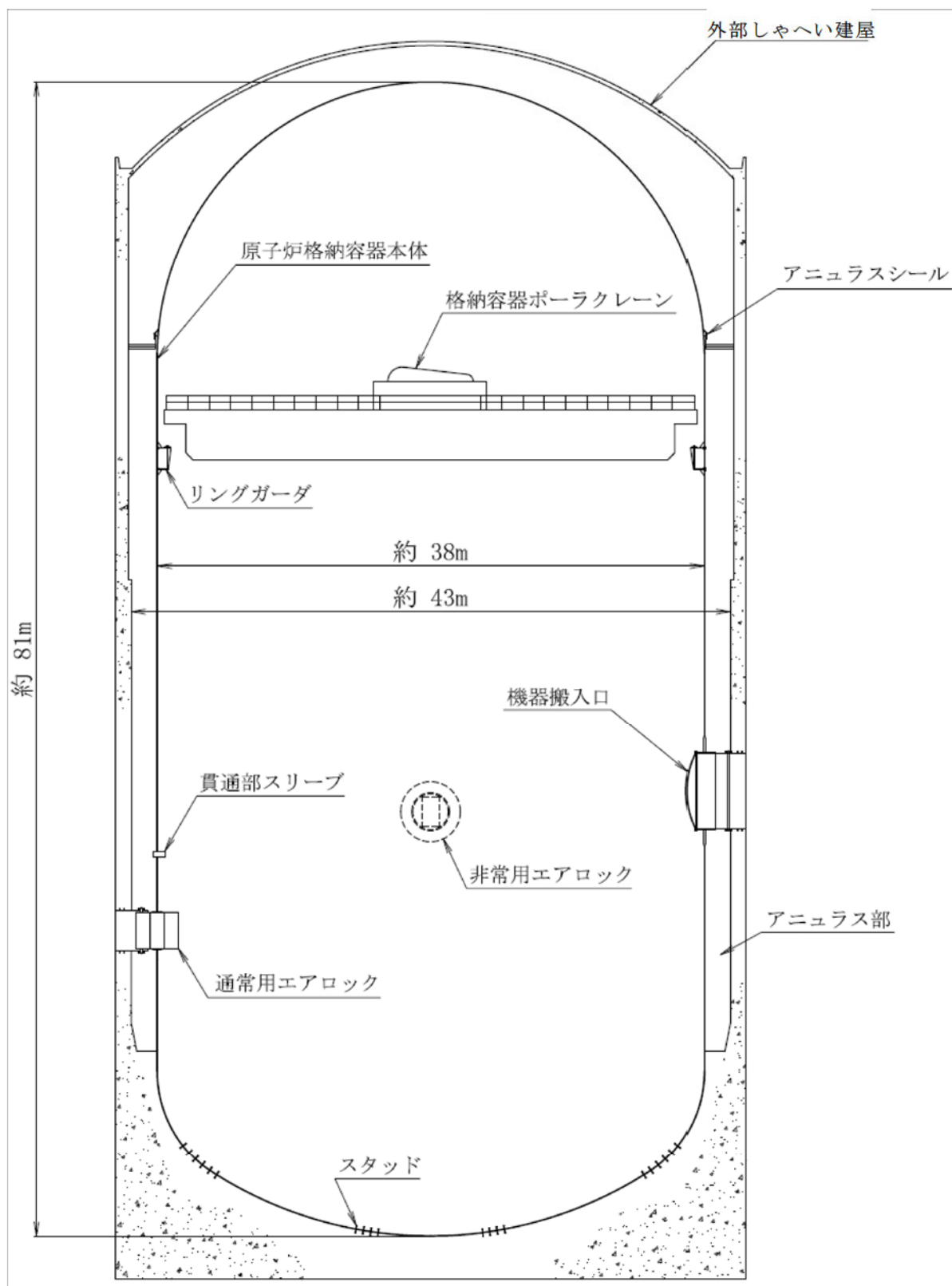
原子炉格納容器本体
