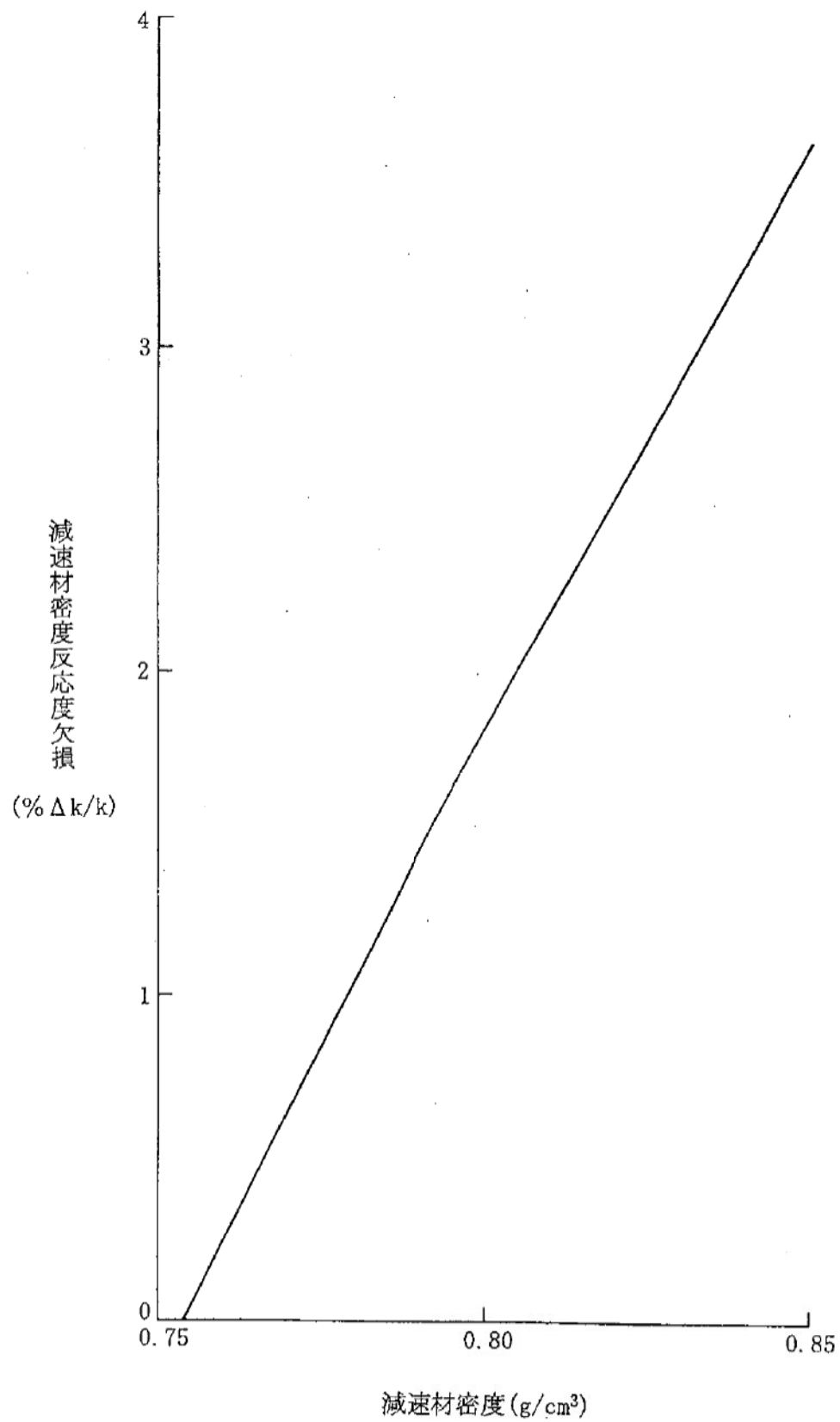
第10.5図 解析に使用した減速材密度反応度欠損
