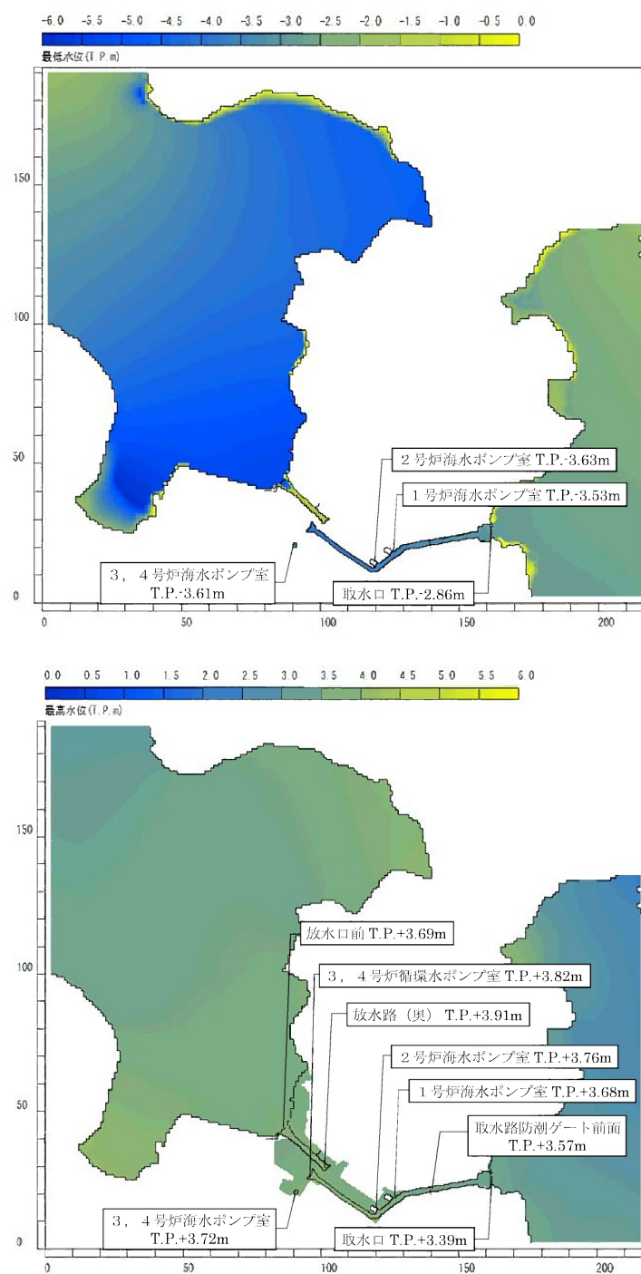
最低水位分布図
