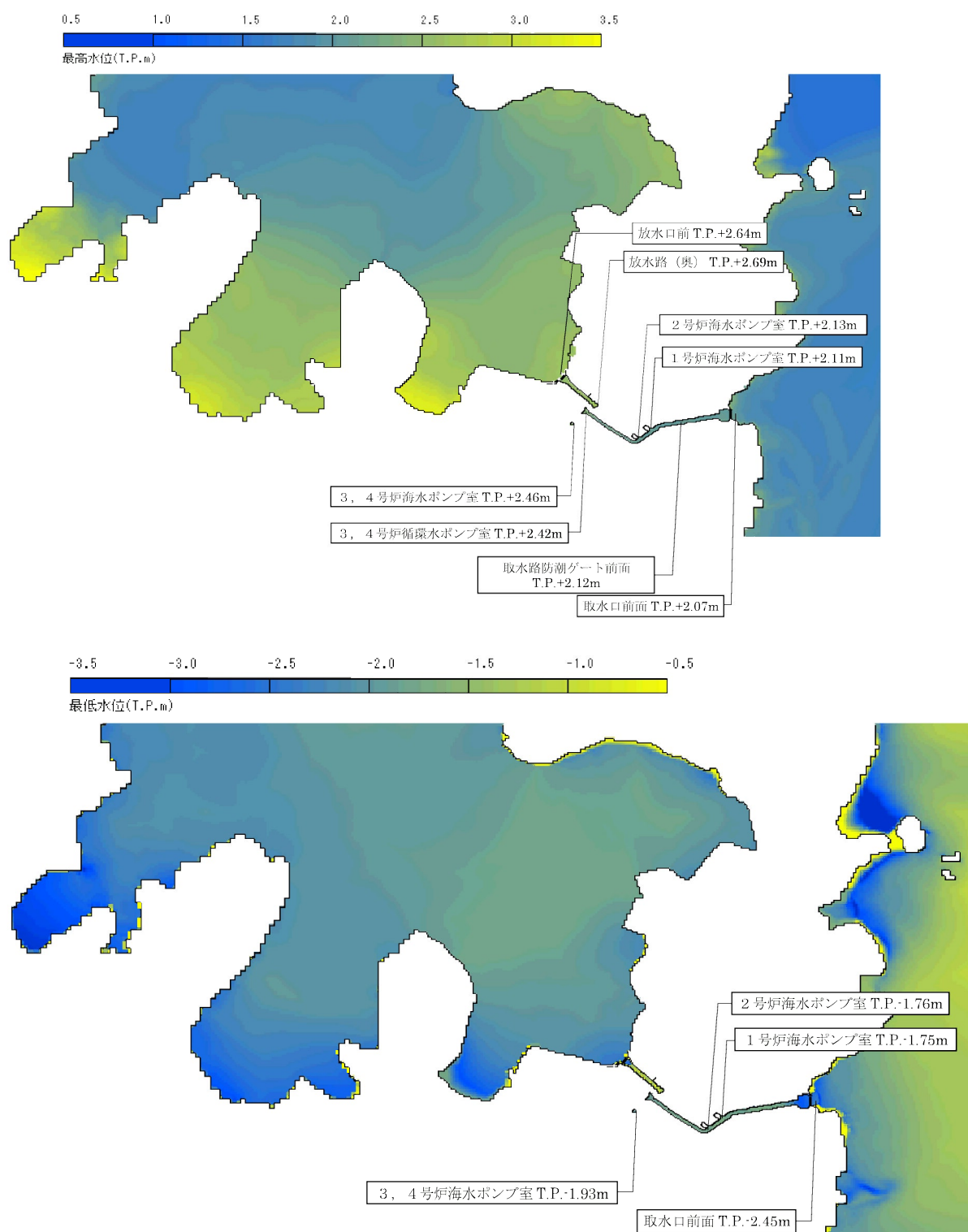
第 1.2.7.3.6 図 基準津波 2 による水位分布図
