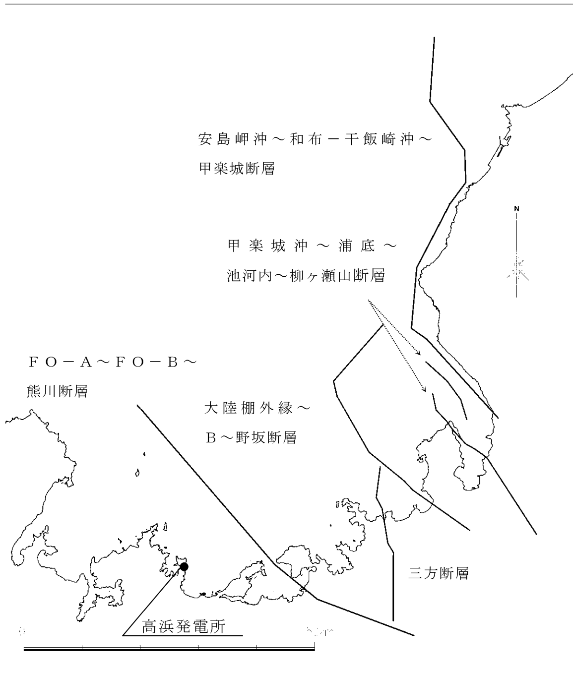
第 1.2.7.2.5 図 敷地周辺の海域における検討対象断層
