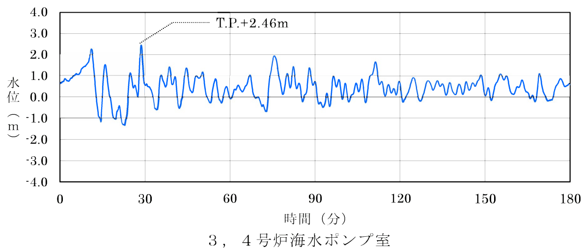
第 1.2.7.3.2 図(2) 基準津波 2 の時刻歴波形 (水位上昇側)
