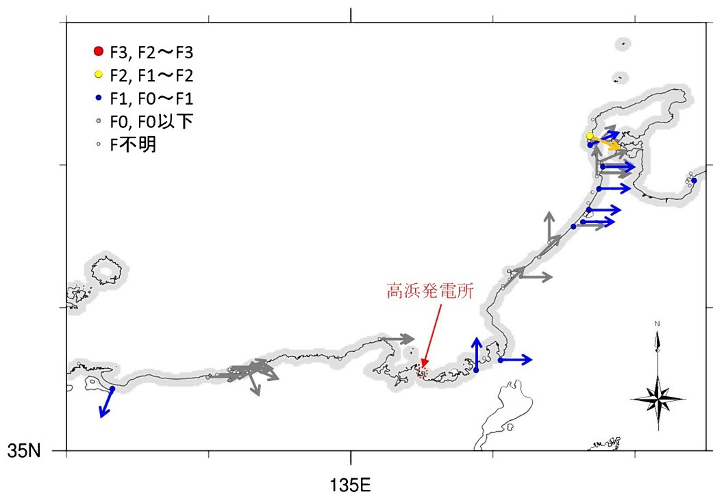
第 1.2.9.2.1 図 竜巻の移動方向の個数（鳥取県～石川県）
