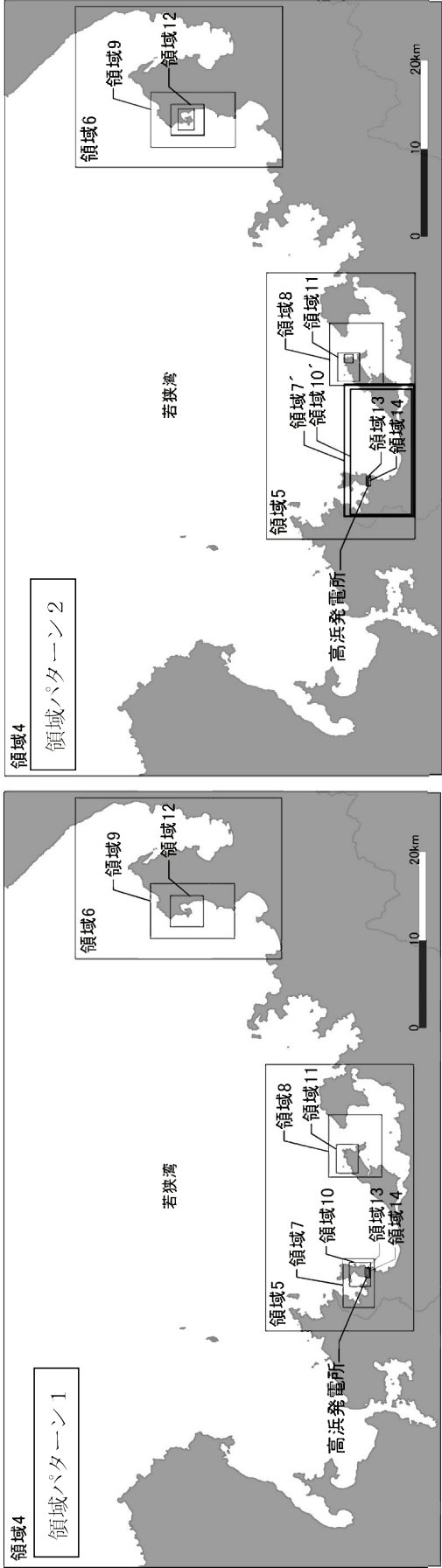
第 1.2.7.2.3 図(1) 詳細津波計算モデル (津波伝播計算領域及び空間格子間隔)
