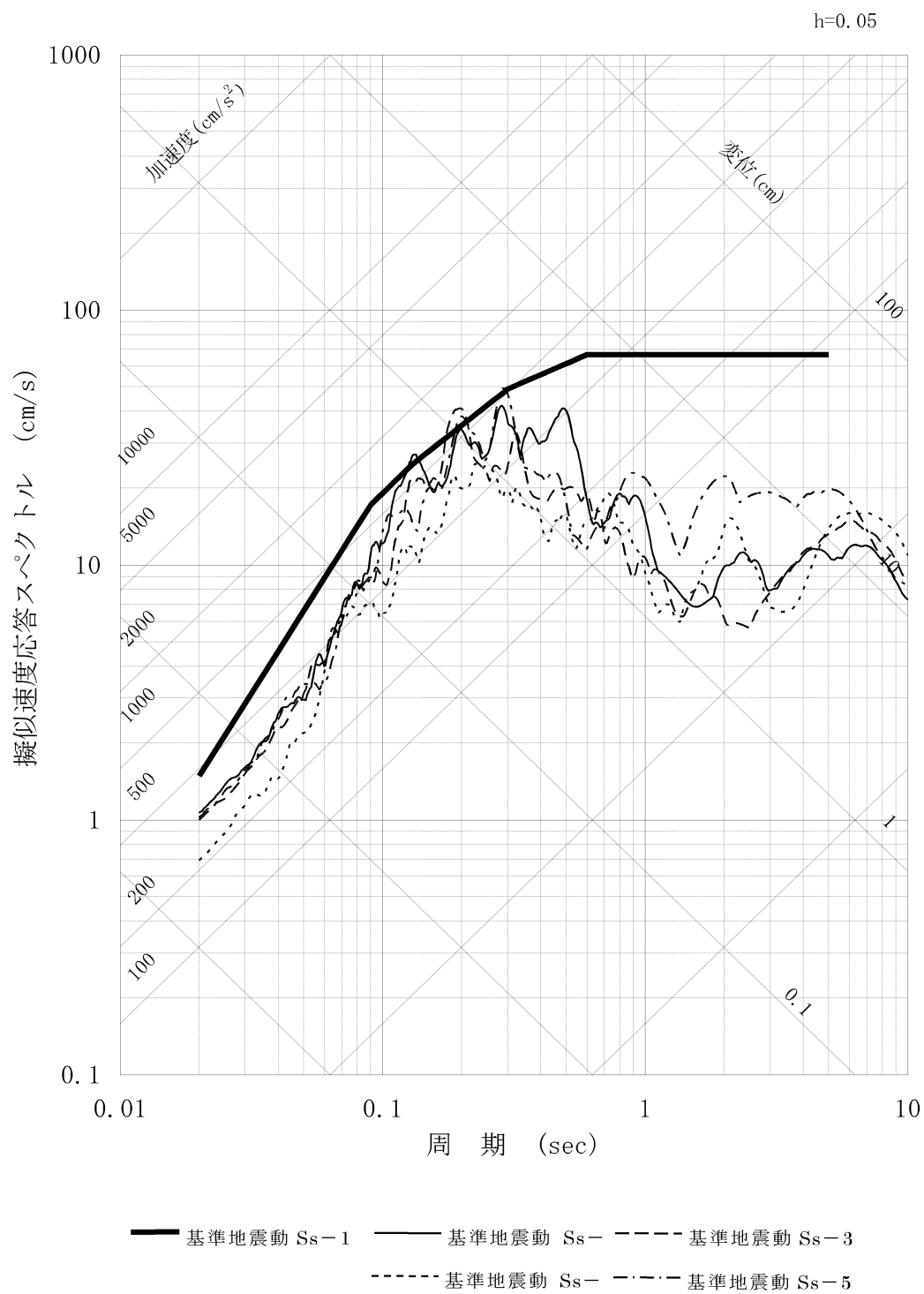
第 1.2.5.6.4 図(3) 基準地震動 Ss-1 と Ss-2～Ss-5 の応答スペクトル (UD 方向)
