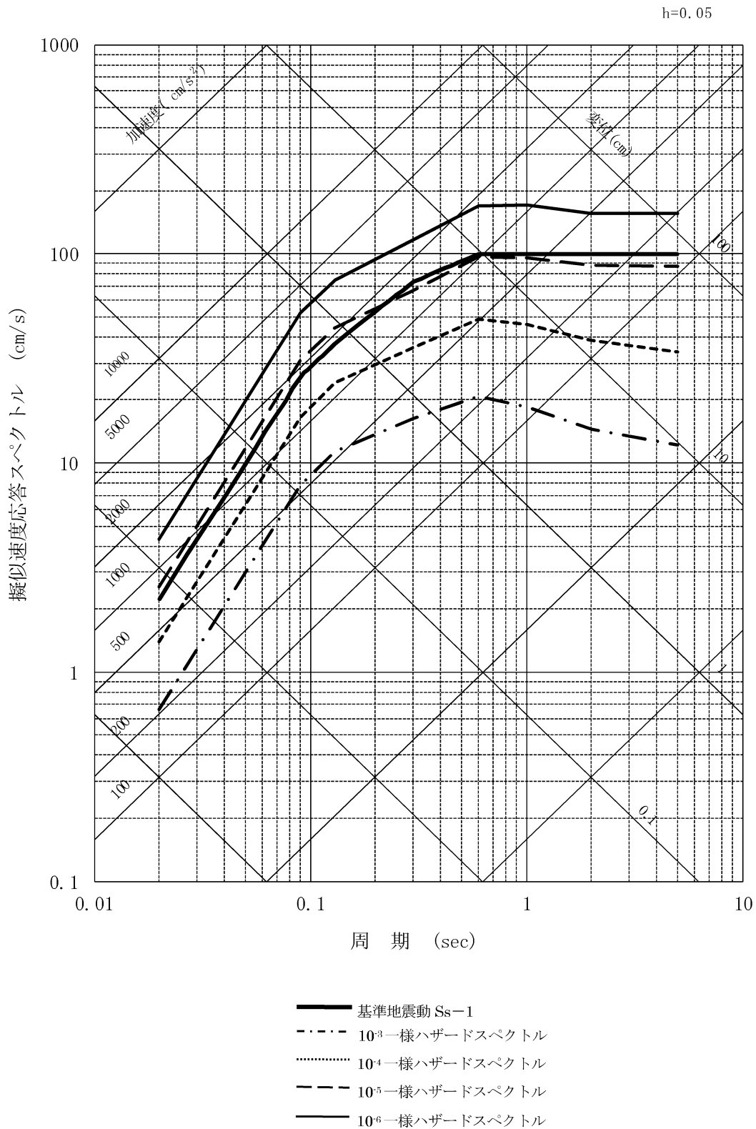
第 1.2.5.8.1 図(1) 基準地震動 S_s-1 と一様ハザードスペクトルの比較 (水平方向)
