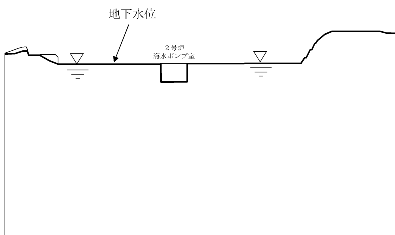
第 1.2.3.5.25 図 解析用地下水位（I－I'）
