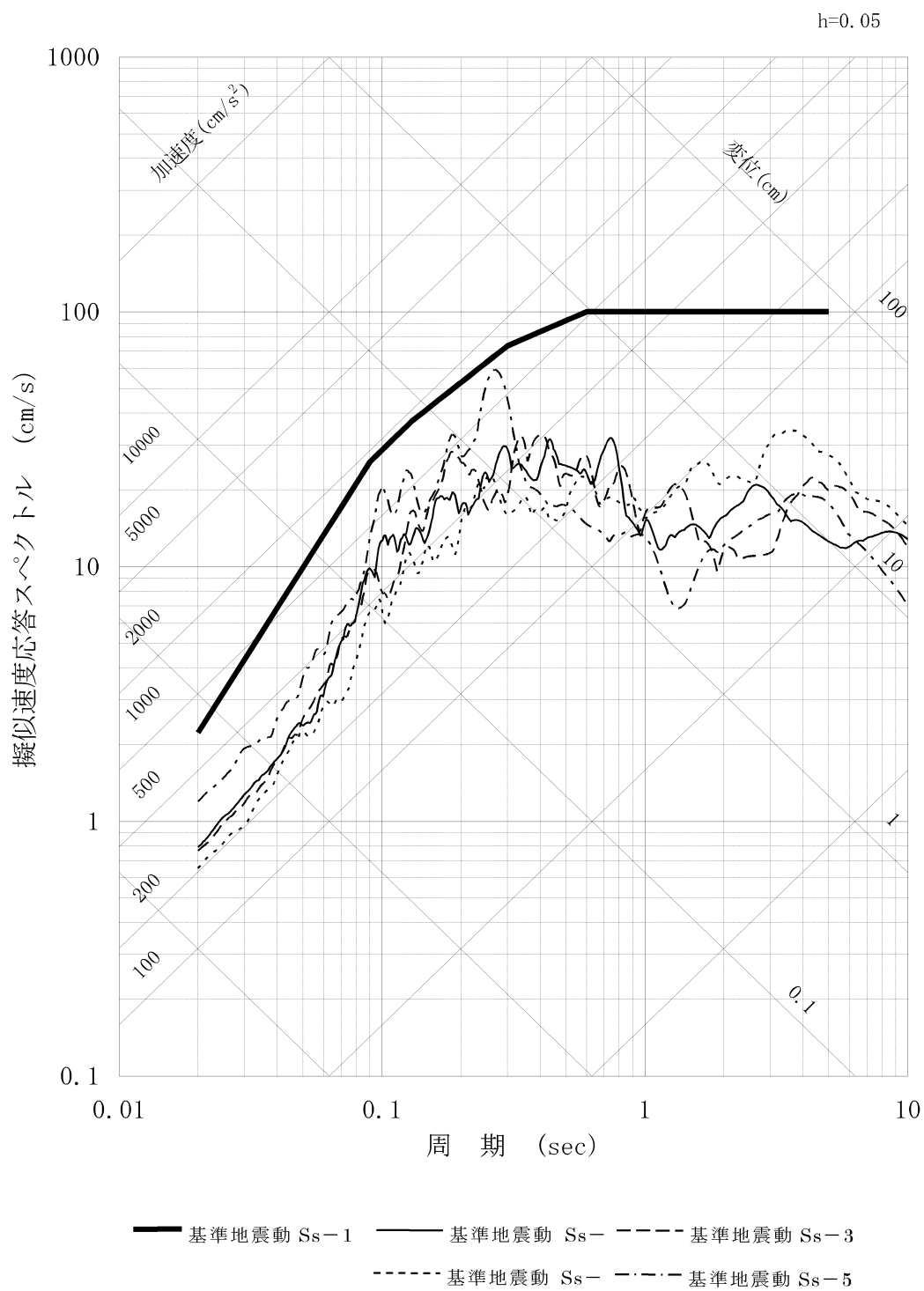
第 1.2.5.6.4 図(2) 基準地震動 Ss-1 と Ss-2～Ss-5 の応答スペクトル (EW 方向)
