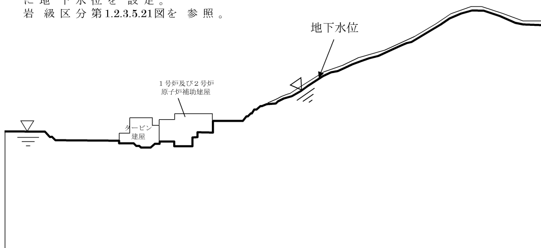
第 1.2.3.5.24 図 解析用地下水位（G－G'）
