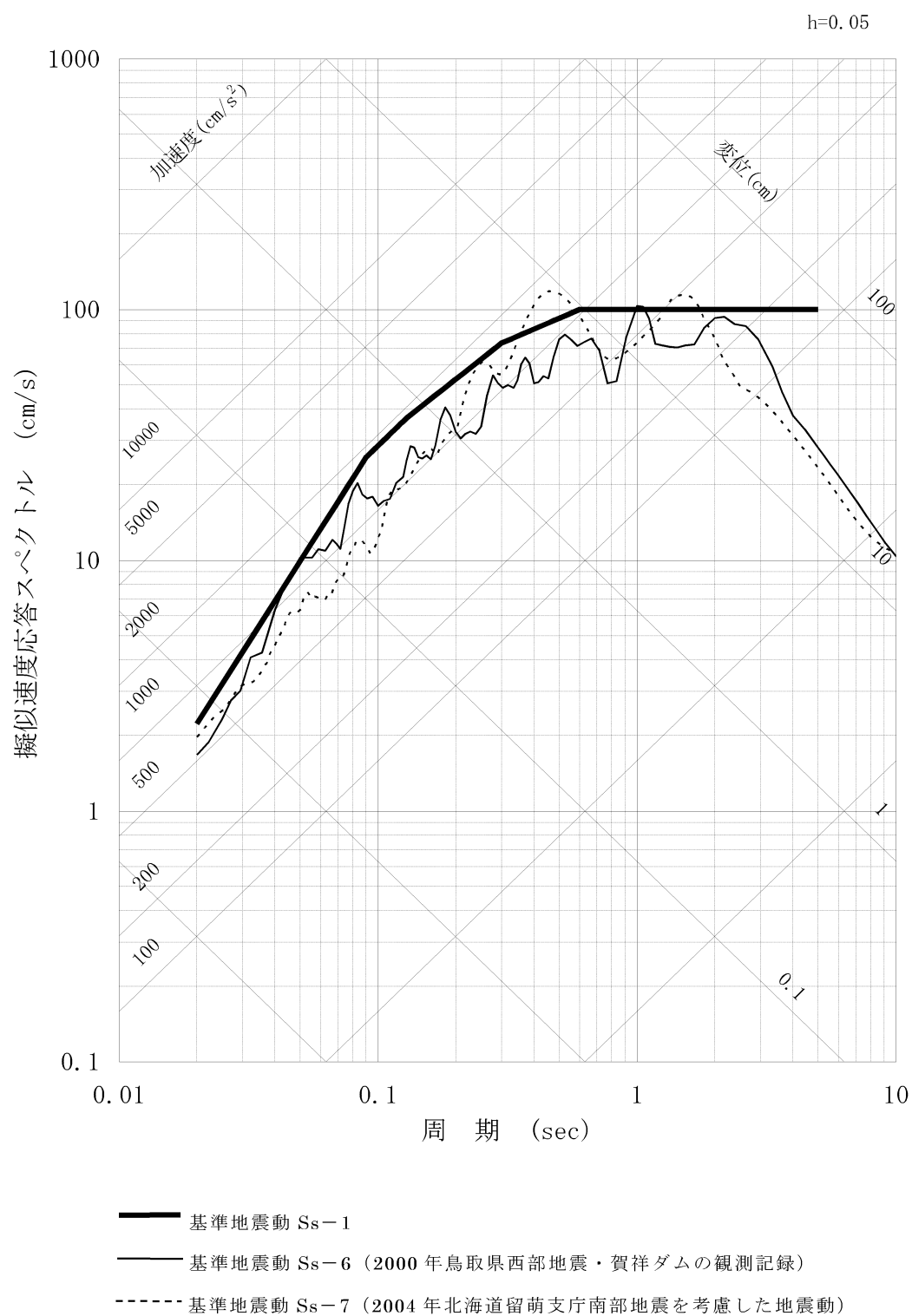
第 1.2.5.6.5 図(2) 基準地震動 Ss-1 と Ss-6, Ss-7 の応答スペクトル (EW 方向)
