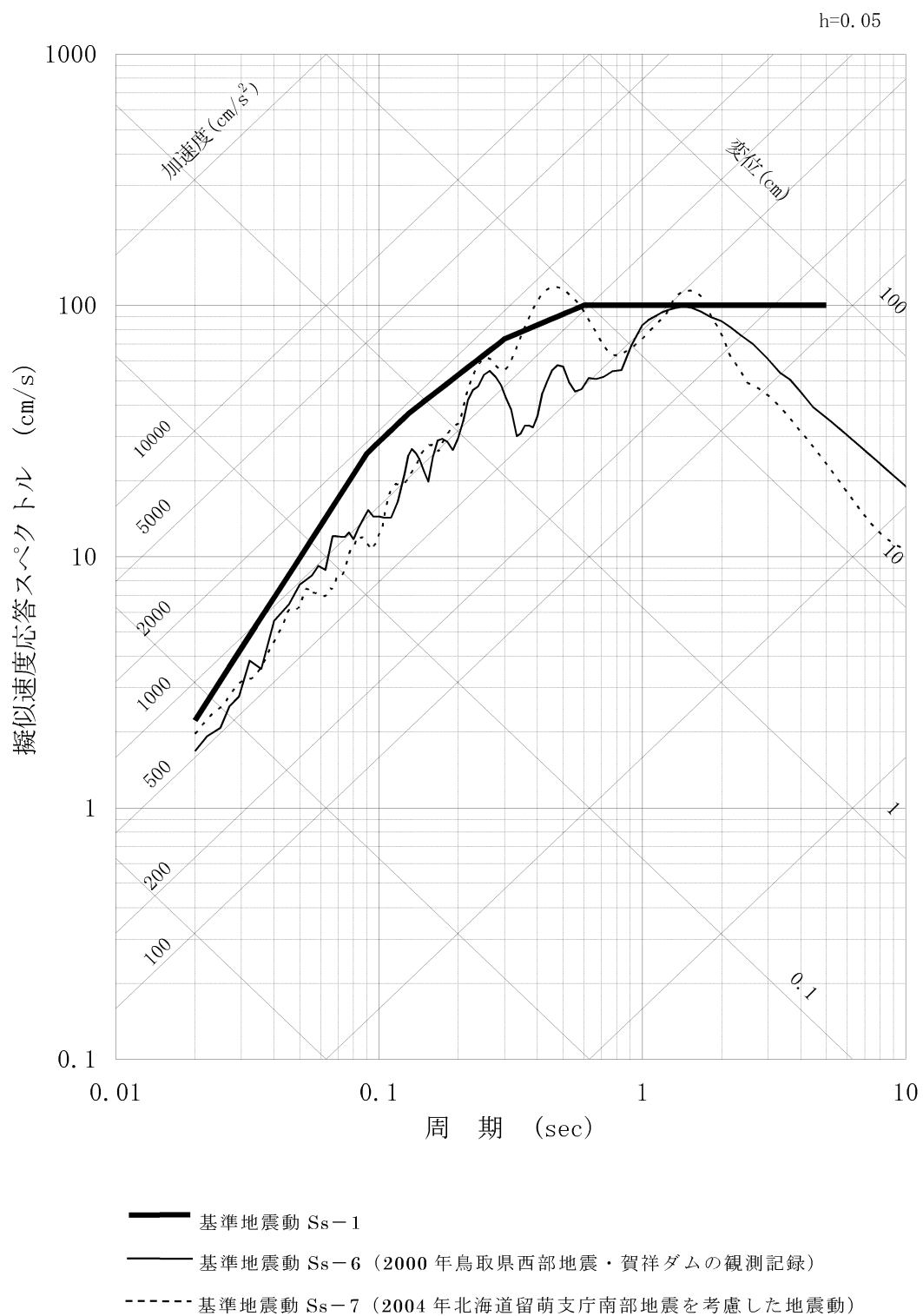
第 1.2.5.6.5 図(1) 基準地震動 Ss-1 と Ss-6, Ss-7 の応答スペクトル (NS 方向)
