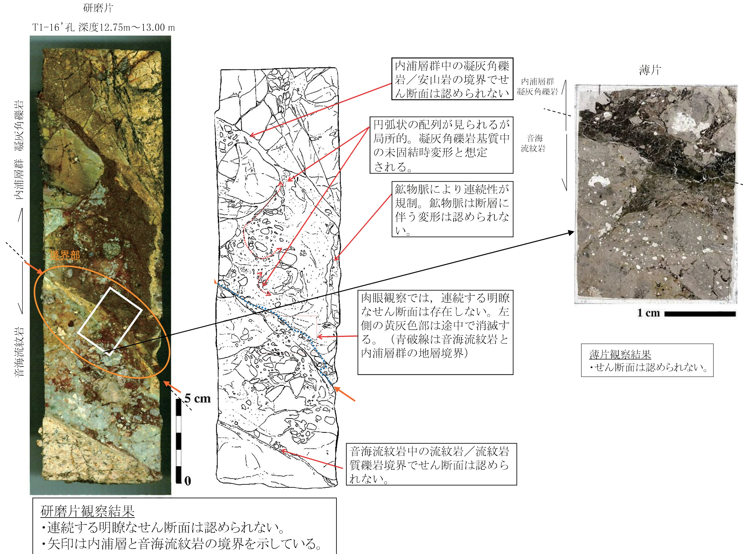
第 1.2.3.31 図 音海流紋岩と内浦層群の境界部の研磨片・薄片観察結果 (T1-16' 孔)
