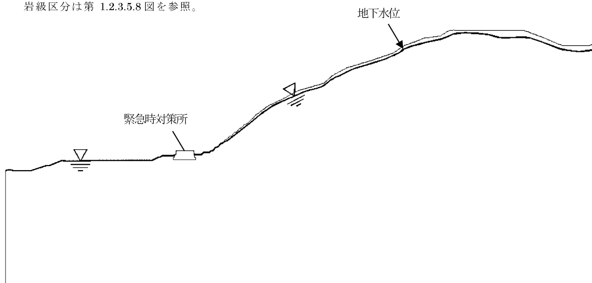
第 1.2.3.5.19 図 解析用地下水位（J－J'）
