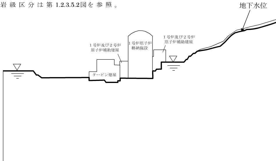
第1.2.3.5.13図 解析用地下水位（A－A'）
