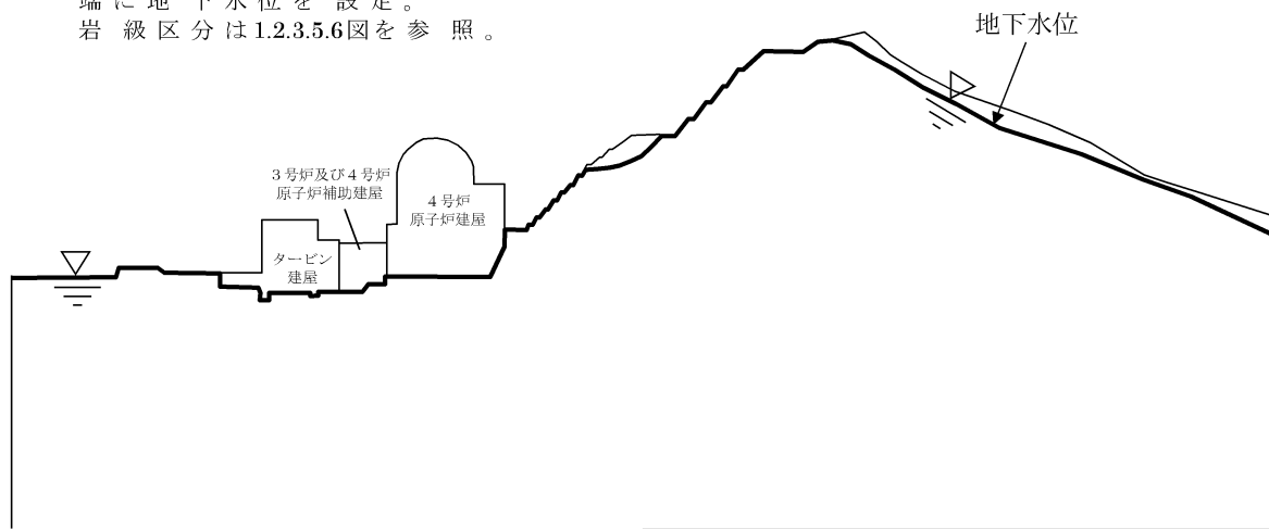
第 1.2.3.5.17図 解析用地下水位（E－E'）
