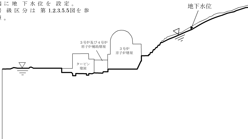
第 1.2.3.5.16図 解析用地下水位（D－D'）
