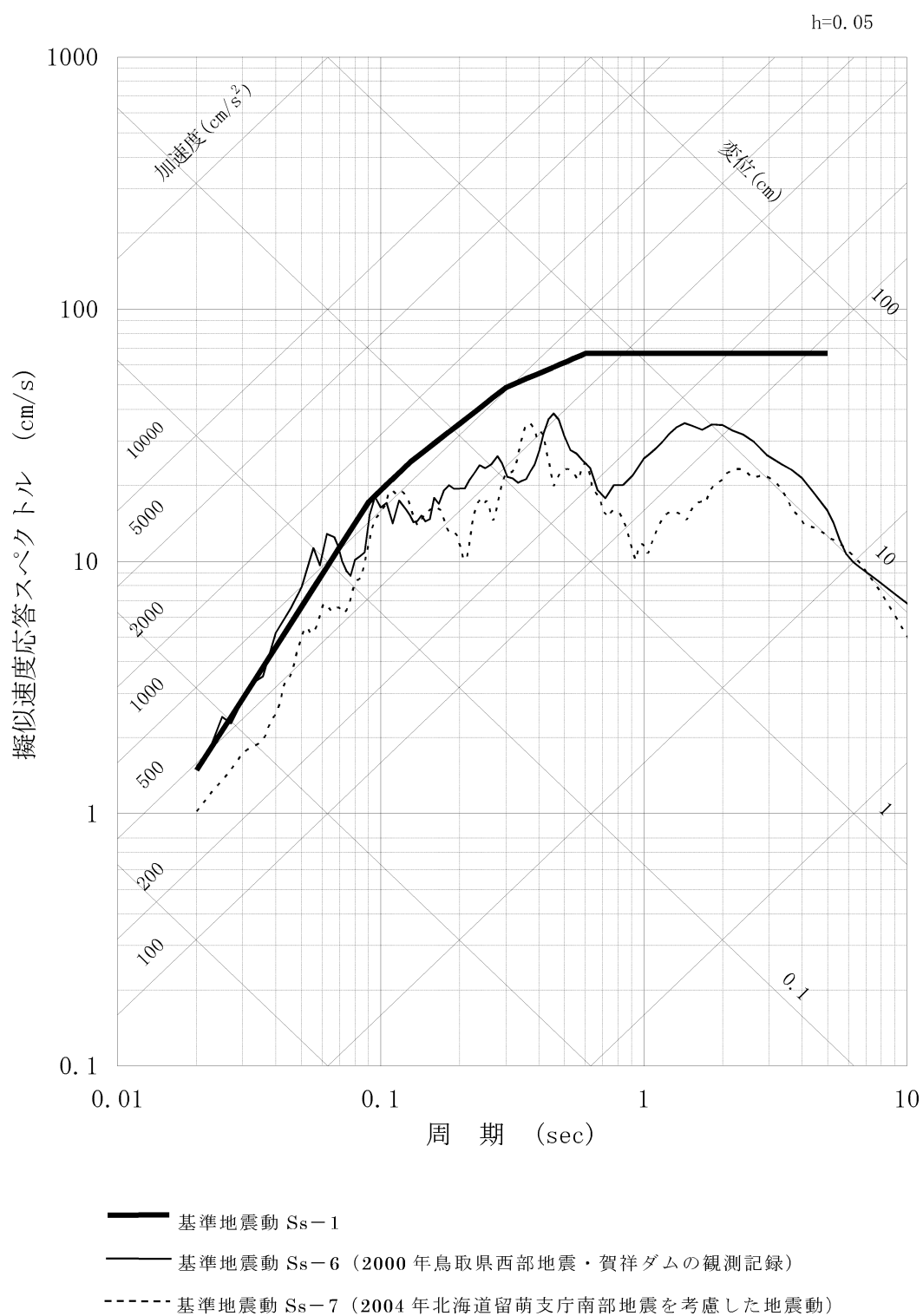
第 1.2.5.6.5 図(3) 基準地震動 Ss-1 と Ss-6, Ss-7 の応答スペクトル (UD 方向)
