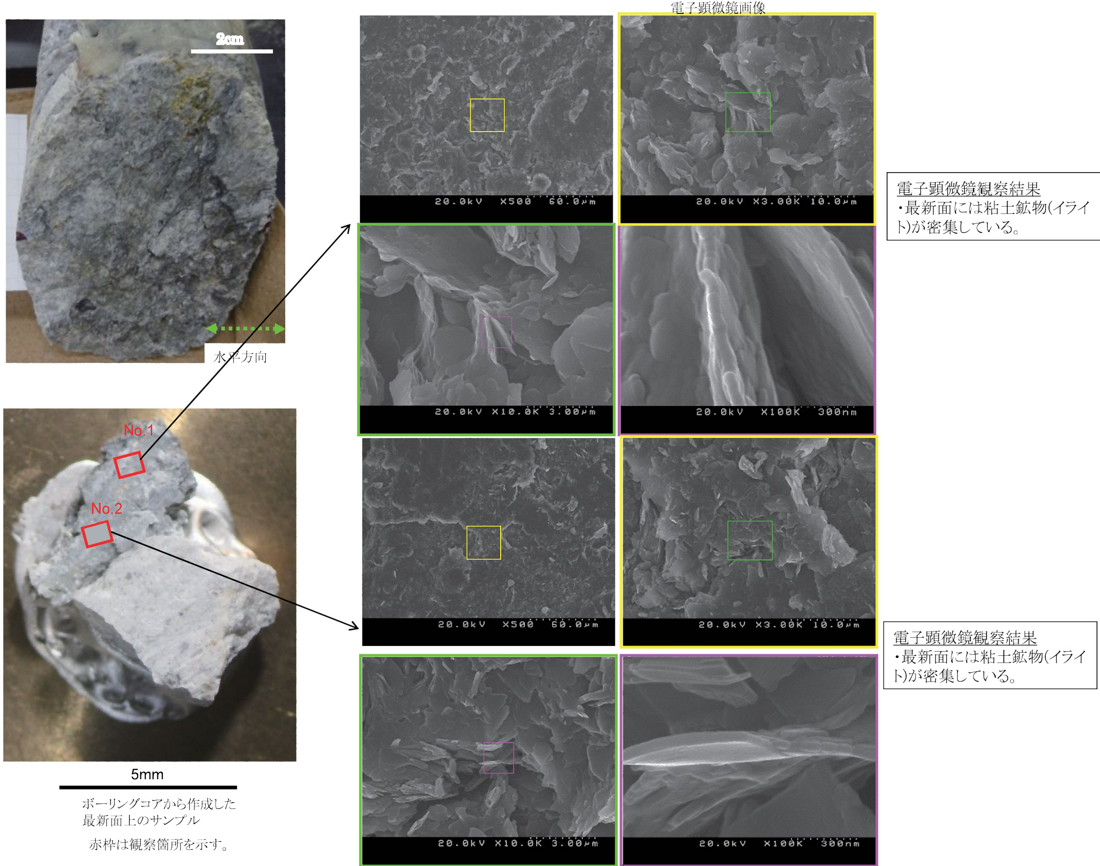
第 1.2.3.3.26図 F - A (H25-5 孔) 電子顕微鏡観察結果 1.2.3-123
