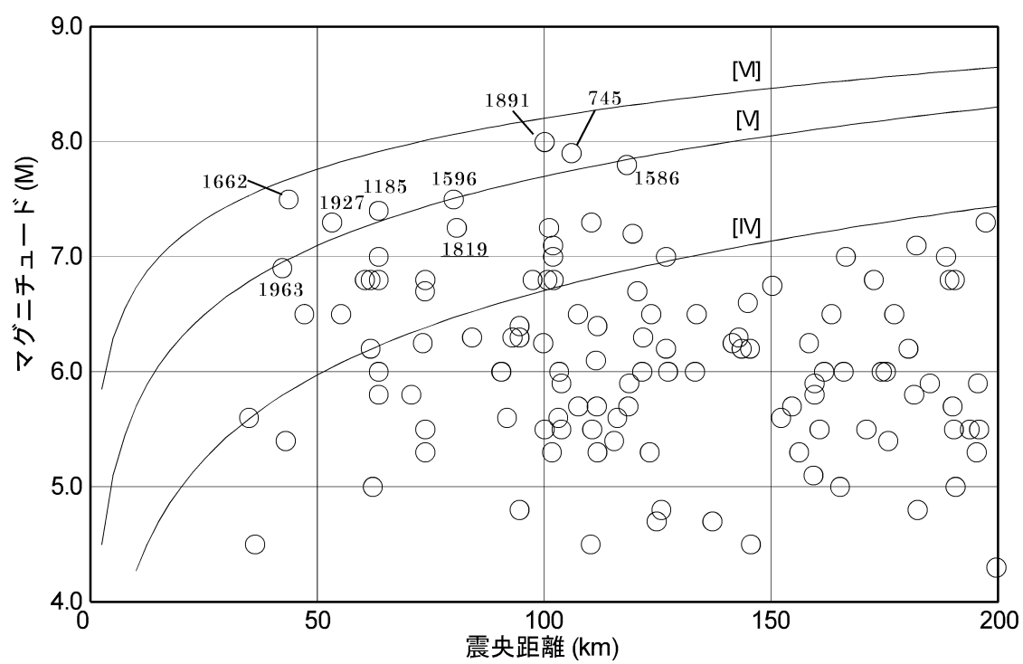
第 1.2.5.2.1 図 敷地周辺の被害地震のマグニチュードと震央距離の関係
