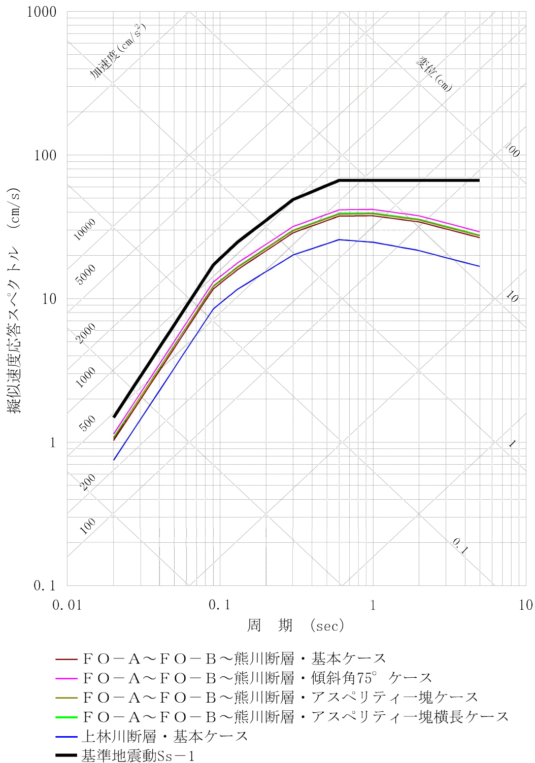
第 1.2.5.6.2 図(2) 基準地震動 Ss-1 の応答スペクトルと応答スペクトルに基づく地震動評価結果の比較 (鉛直方向)
