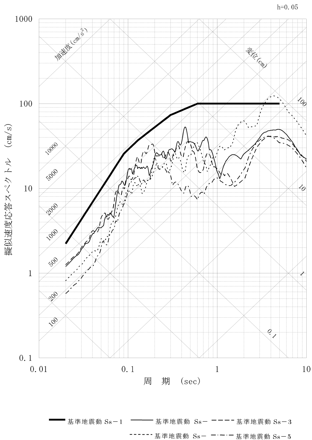
第 1.2.5.6.4 図(1) 基準地震動 Ss-1 と Ss-2～Ss-5 の応答スペクトル (NS 方向)
