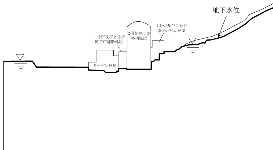
第1.2.3.5.14図 解析用地下水位（B－B'）
