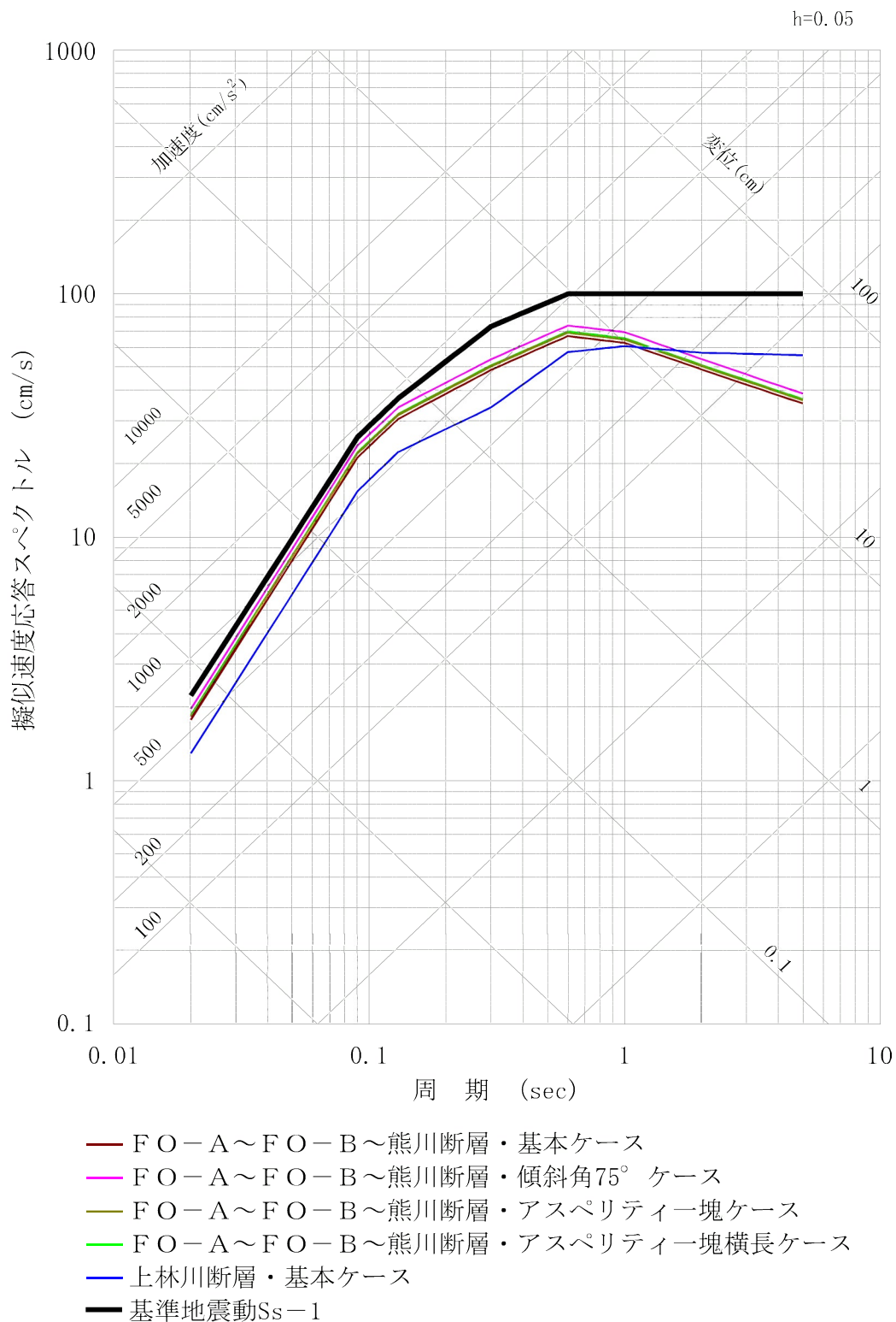
第 1.2.5.6.2 図(1) 基準地震動 Ss-1 の応答スペクトルと応答スペクトルに基づく地震動評価結果の比較 (水平方向)
