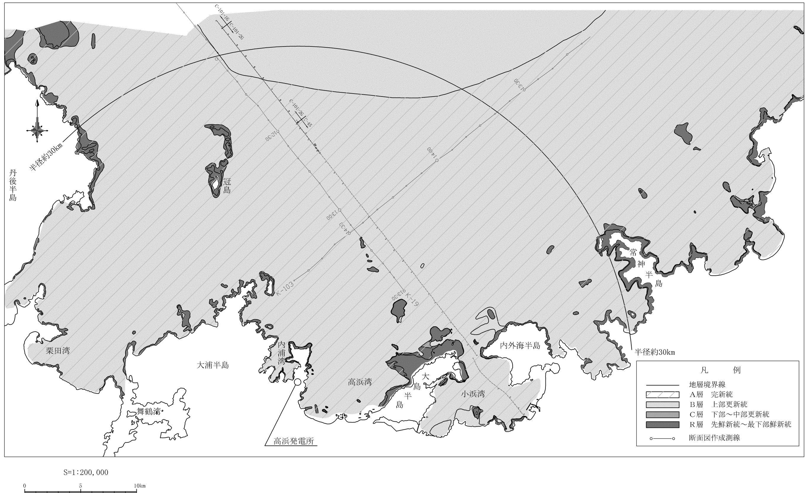
第1.2.3.1.21図 敷地前面海域の海底地質図
