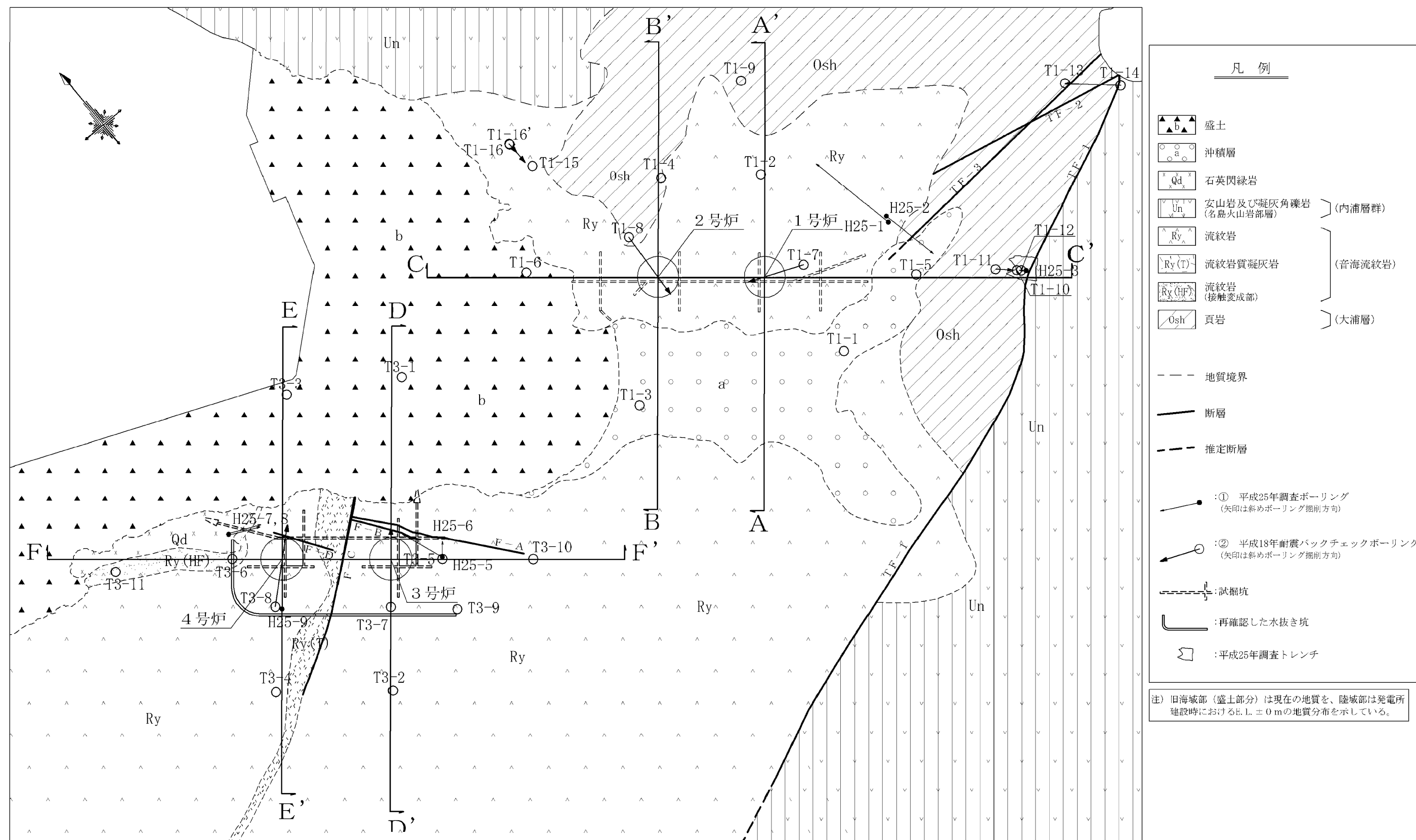
第1.2.3.3.3 図 敷地の水平地質断面図(E. L. ±0m)
