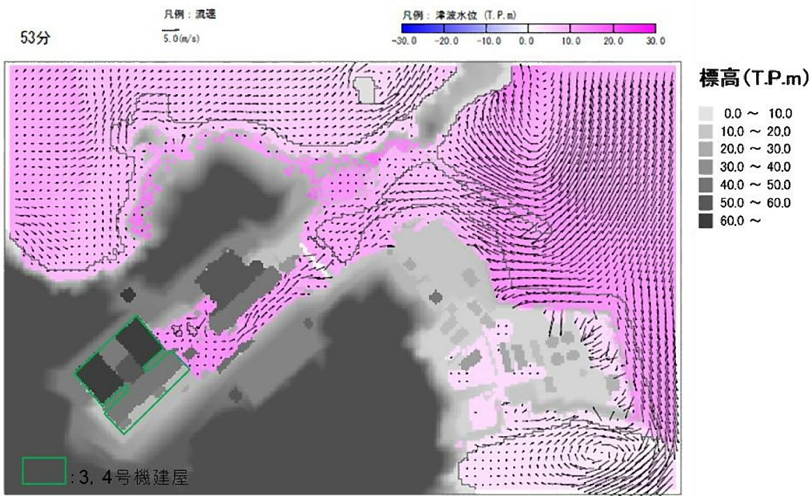
第 3.1.4.2.2.11 図 流速ベクトル分布 (3, 4号機海水ポンプ室前潮位 : E.L.+15.8m)
