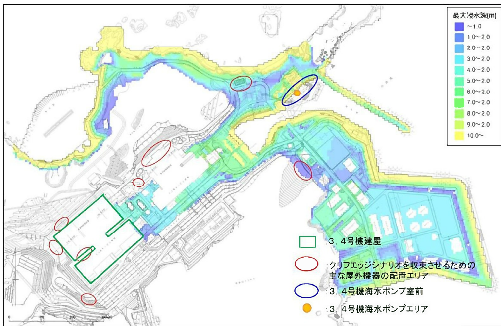
第 3.1.4.2.2.10 図 最大浸水深分布 (3, 4号機海水ポンプ室前潮位 : E.L.+15.8m)
