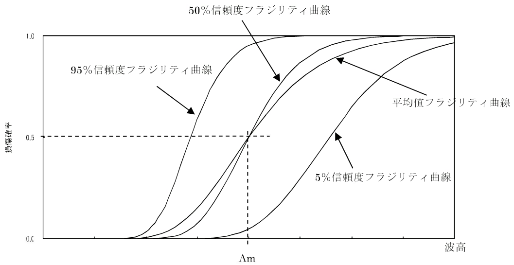
第 3.1.3.2.2.3.1 図 信頼度に応じた fragility 曲線のイメージ
