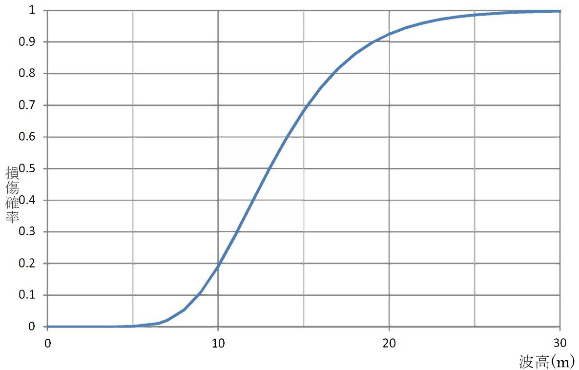
第 3.1.3.2.2.3.2 図 fragility 曲線 (被水・没水 (屋外)) : 設置 E.L.13.0m)
