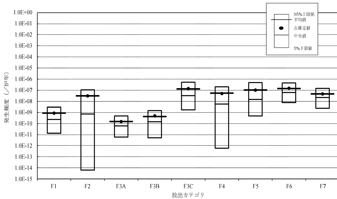
第 3.1.3.2.1.5.5 図 格納容器機能喪失頻度の不確かさ解析結果 (放出カテゴリ別)
