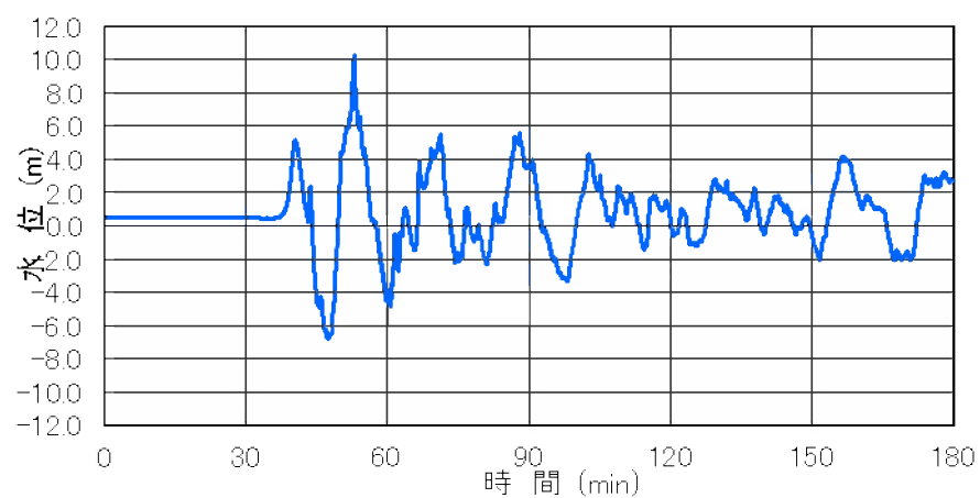
第 3.1.4.2.2.12 図 遡上解析で想定する入力津波の時刻歴波形 (鋸崎から約 1km 離れた海域 (水深 40m 地点)) (3, 4 号機海水ポンプ室前潮位 : E.L. + 15.8m) (初期潮位 : E.L. + 0.49m)
