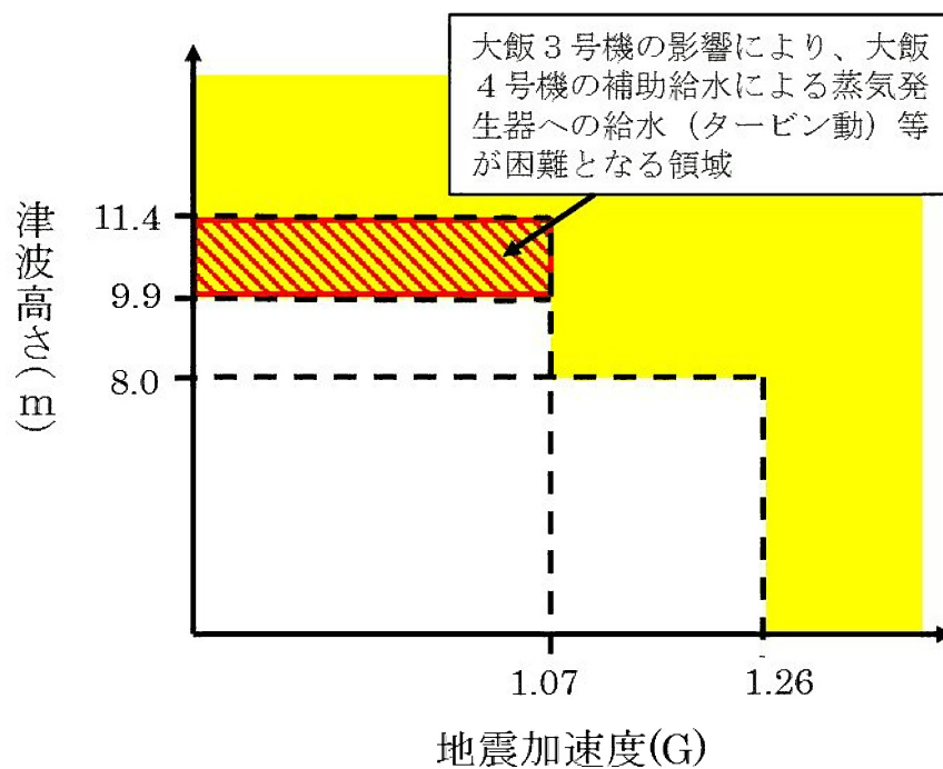
第 3.1.4.4.1.2 図 大飯3号機からの影響を考慮した大飯4号機の地震と津波の重畳に関するクリフエッジ評価結果（出力運転時炉心）
