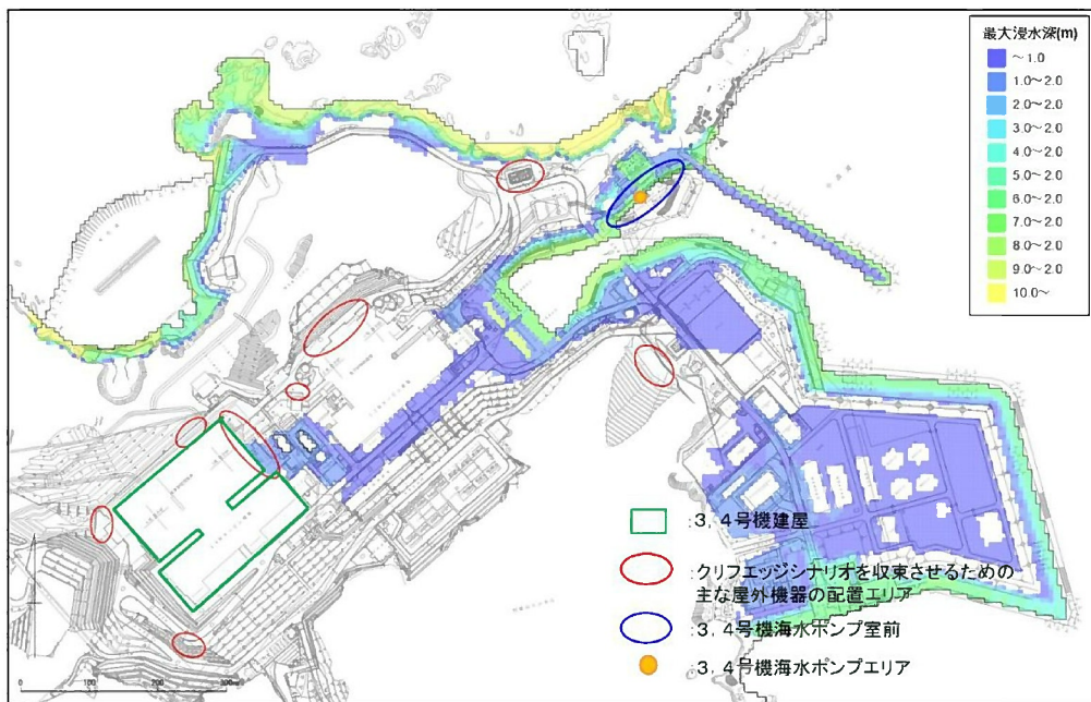
第 3.1.4.2.2.8 図 最大浸水深分布 ( 3 , 4 号機海水ポンプ室前潮位 : E.L.+9.9m)
