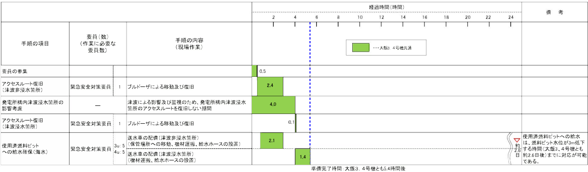
第 3.1.4.3.1.7 図 使用済燃料ピットへの送水車ポンプによる海水注水の 対応手順と所要時間
