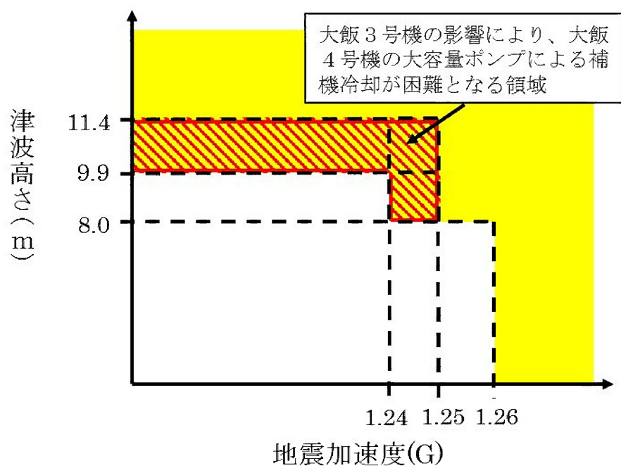
第 3.1.4.4.1.3 図 大飯 3 号機からの影響を考慮した大飯 4 号機の地震と津波の重畳に関するクリフエッジ評価結果（運転停止時炉心）
