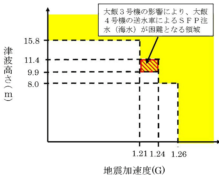
第 3.1.4.4.1.4 図 大飯 3 号機からの影響を考慮した大飯 4 号機の地震と津波の重畳に関するクリフエッジ評価結果（S F P 燃料損傷）
