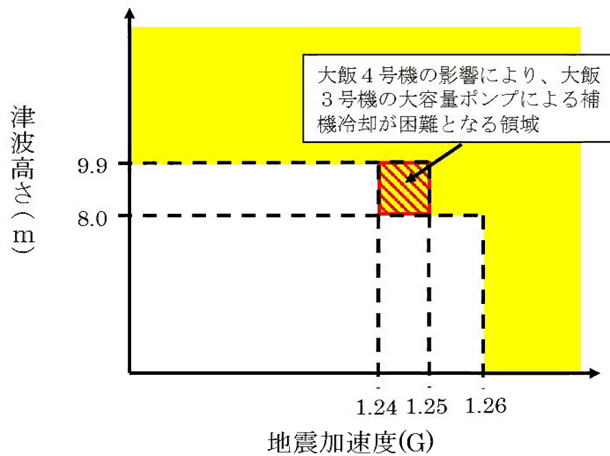
第 3.1.4.4.1.1 図 大飯4号機からの影響を考慮した大飯3号機の地震と津波の重畳に関するクリフエッジ評価結果（運転停止時炉心）
