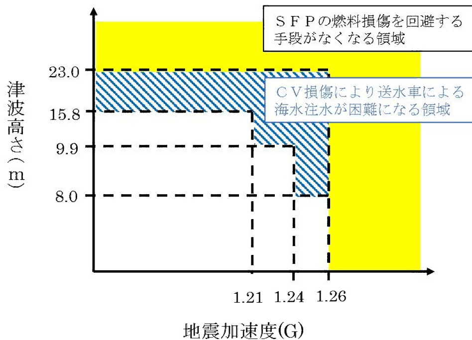
第 3.1.4.2.3.9 図 遡上を考慮した地震と津波の重畳に関するクリフエッジ評価結果（SFP 燃料損傷）
