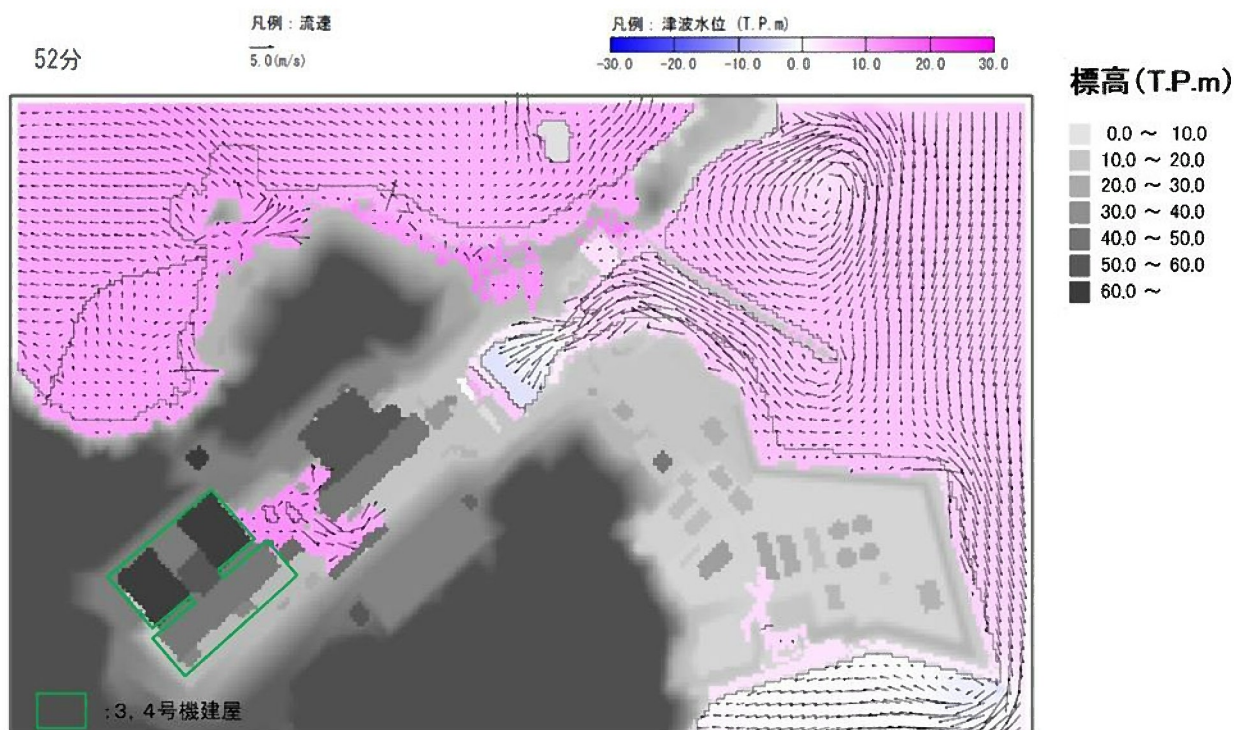
第 3.1.4.2.2.5 図 流速ベクトル分布
