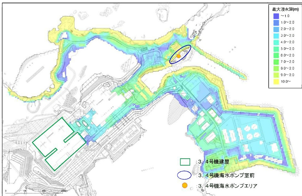
第 3.1.4.2.2.14 図 最大浸水深分布 ( 3 , 4 号機海水ポンプ室前潮位 : E.L.+15.8m )
