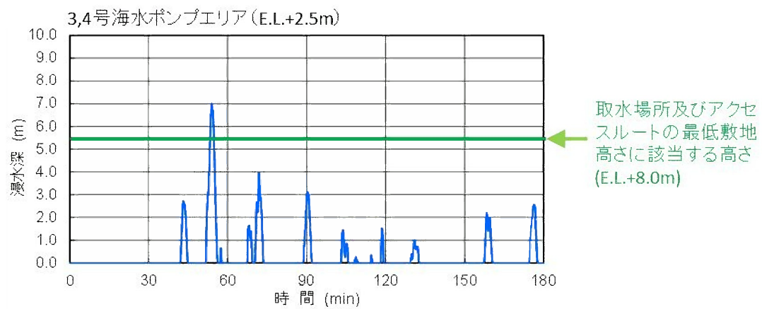
第 3.1.4.2.2.10 図 3, 4 号機海水ポンプエリア(E.L.+2.5m) の津波水位変化
