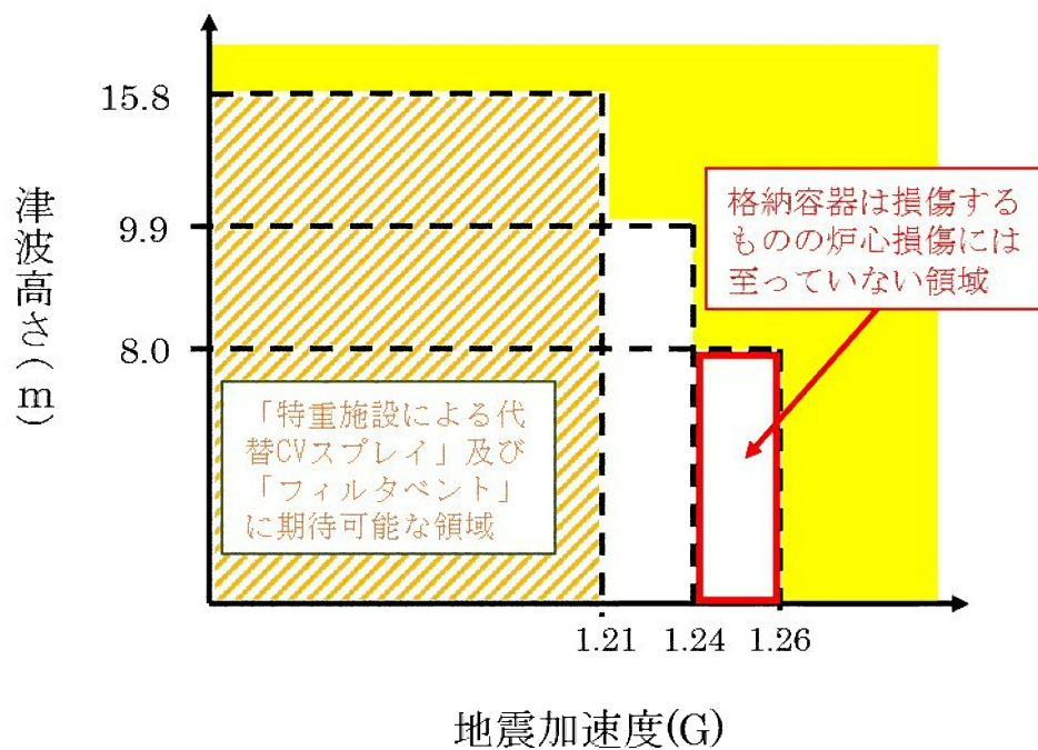
第 3.1.4.2.3.8 図 遡上を考慮した地震と津波の重畳に関するクリフエッジ評価結果（格納容器損傷）
