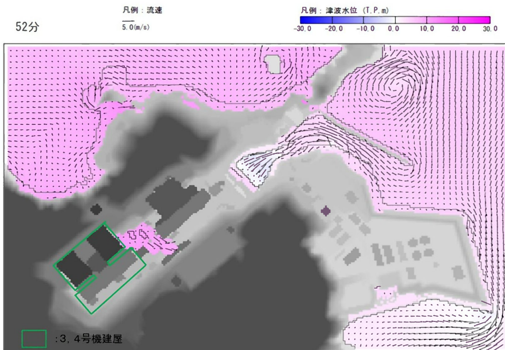
第 3.1.4.2.2.9 図 流速ベクトル分布 ( 3 , 4 号機海水ポンプ室前潮位 : E.L.+9.9m)
