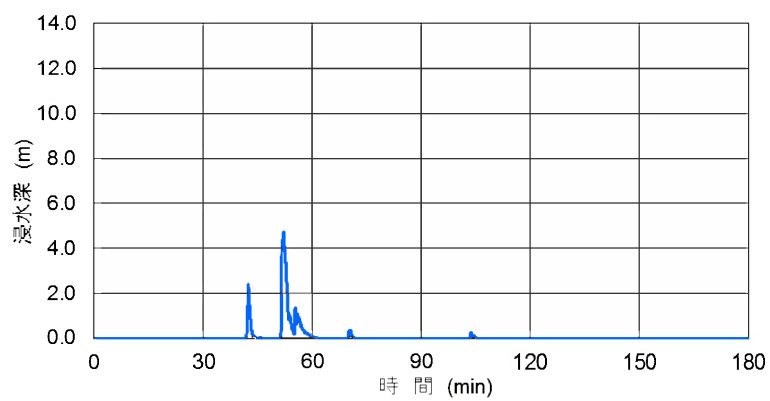
第 3.1.4.2.2.16 図 3, 4 号機建屋周辺エリアの津波水位変化
