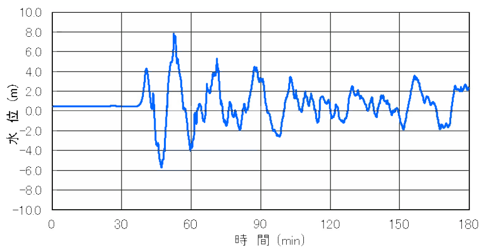
第 3.1.4.2.2.2 図 遡上解析で想定する入力津波の時刻歴波形 (鋸崎から約 1km 離れた海域 (水深 40m 地点)) (3, 4 号機海水ポンプ室前潮位 : E.L. + 11.4m) (初期潮位 : E.L. + 0.49m)
