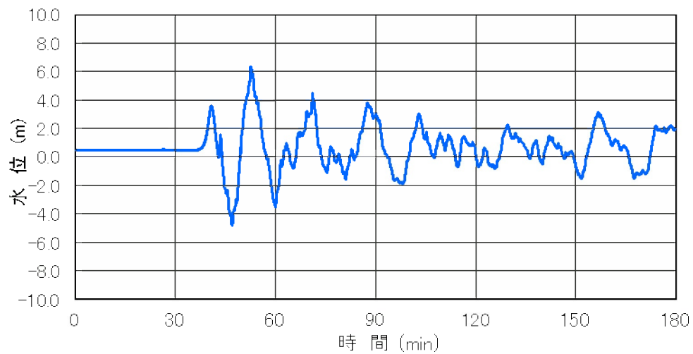
第 3.1.4.2.2.6 図 遡上解析で想定する入力津波の時刻歴波形 (鋸崎から約 1km 離れた海域 (水深 40m 地点)) (3, 4 号機海水ポンプ室前潮位 : E.L.+9.9m) (初期潮位 : E.L.+0.49m)
