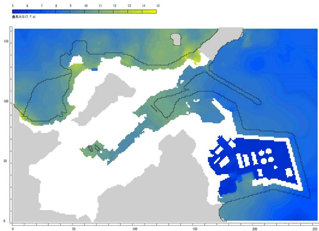
第 3.1.4.2.2.7 図 最高水位分布 (3, 4 号機海水ポンプ室前潮位 : E.L.+9.9m)
