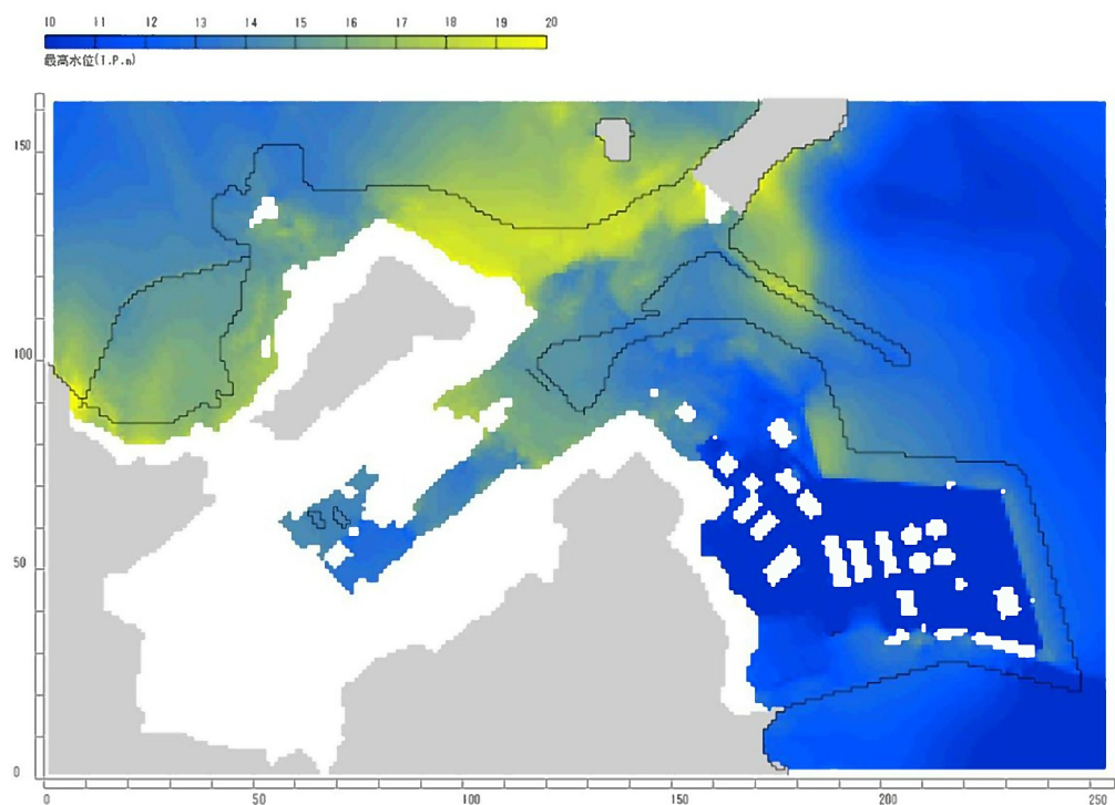
第 3.1.4.2.2.13 図 最高水位分布 (3, 4 号機海水ポンプ室前潮位 : E.L. + 15.8m)
