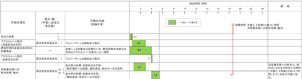
第 3.1.4.3.1.3 図 2 次系冷却継続のための海水の復水ピット補給の 対応手順と所要時間
