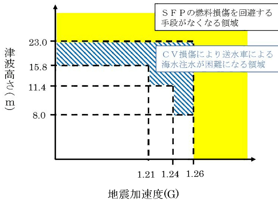
第 3.1.4.2.3.5 図 地震と津波の重畳に関するクリフエッジ評価結果 (SFP燃料損傷)
