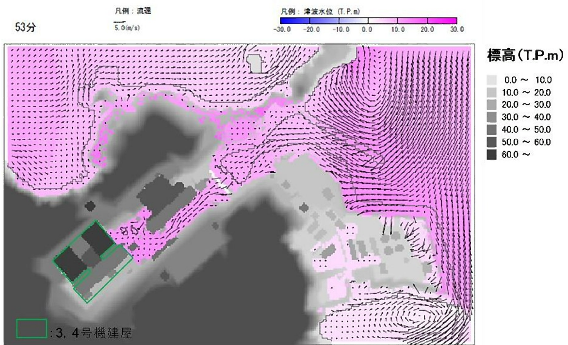
第 3.1.4.2.2.15 図 流速ベクトル分布 ( 3 , 4 号機海水ポンプ室前潮位 : E.L.+15.8m )
