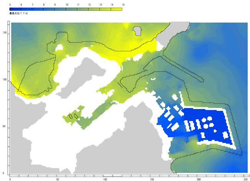
第 3.1.4.2.2.3 図 最高水位分布 (3, 4 号機海水ポンプ室前潮位 : E.L. + 11.4m)
