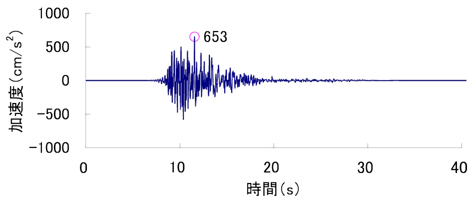
Ss-5 (EW 方向)
