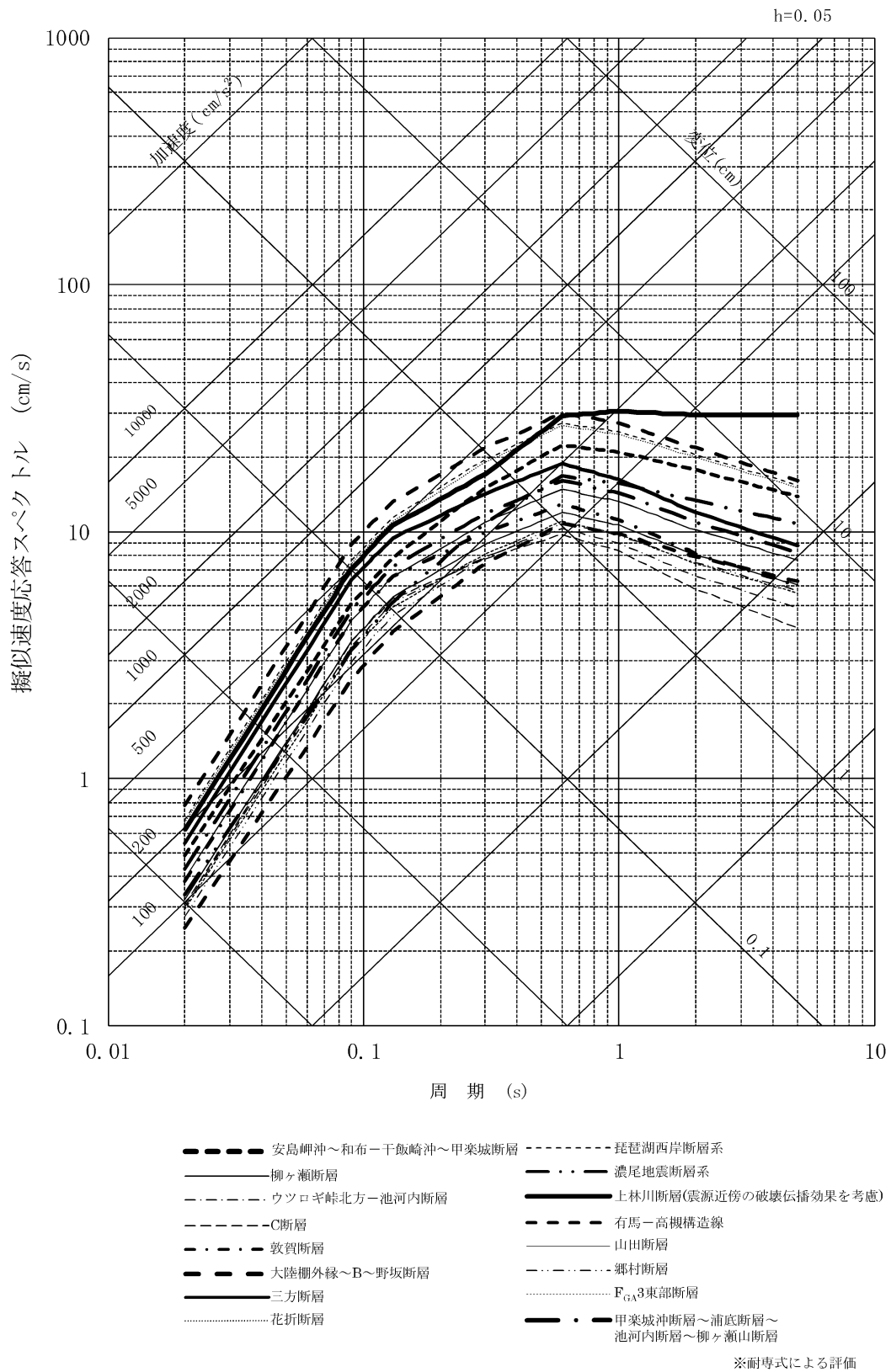
第 1.2.5.4.2 図 敷地に影響を及ぼすと考えられる活断層の地震による応答スペクトル
