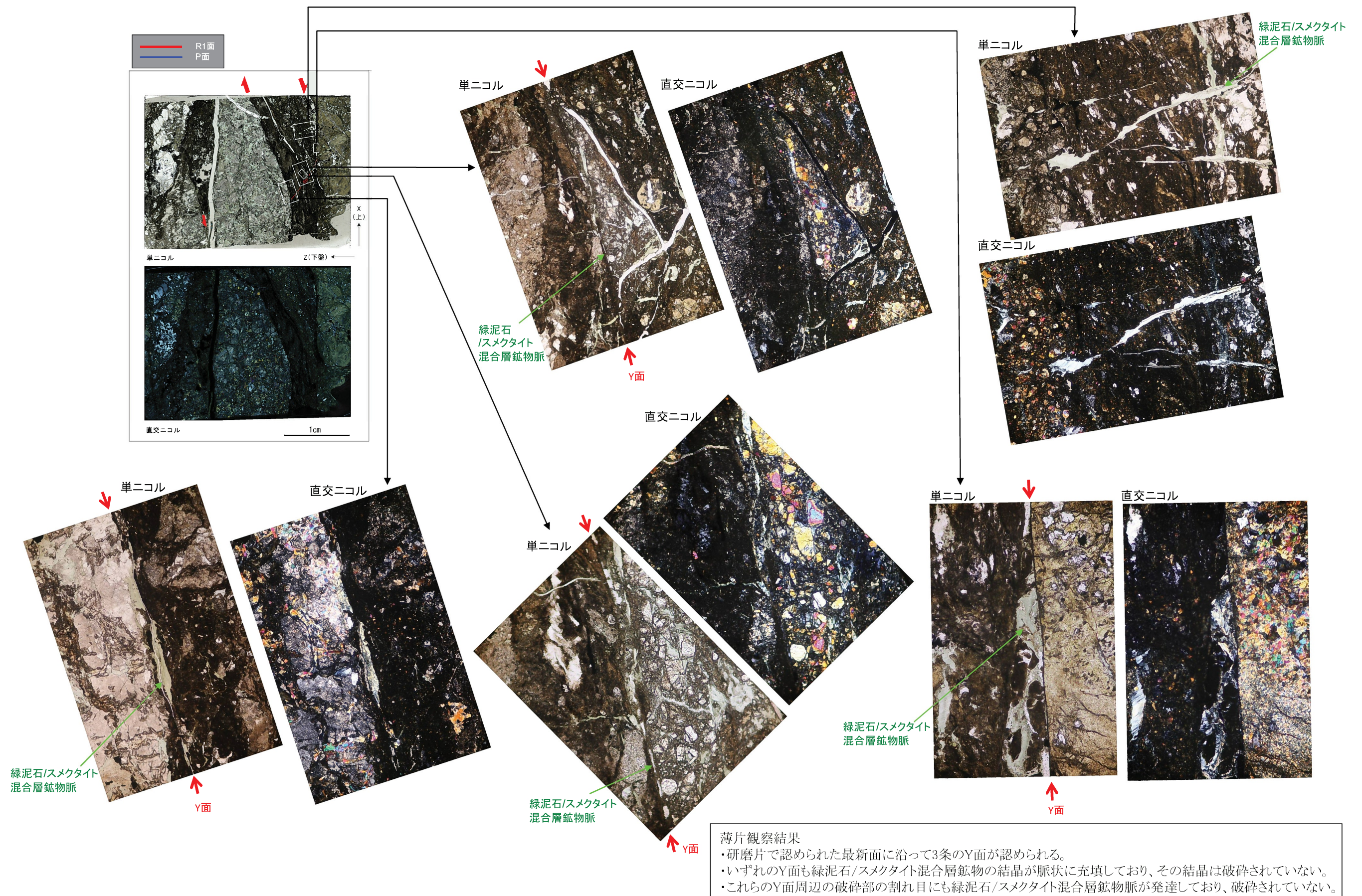
第1.2.3.4.27图(2) F-6破碎带 薄片观察结果 (No.3孔) (2)
