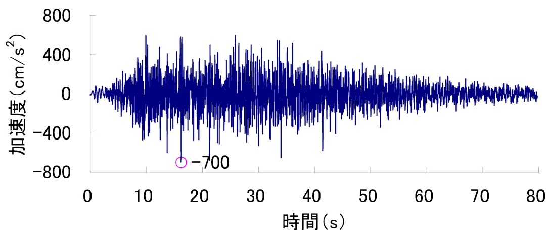
Ss-1（水平方向）
