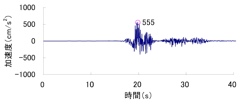
Ss-8 (EW 方向)
