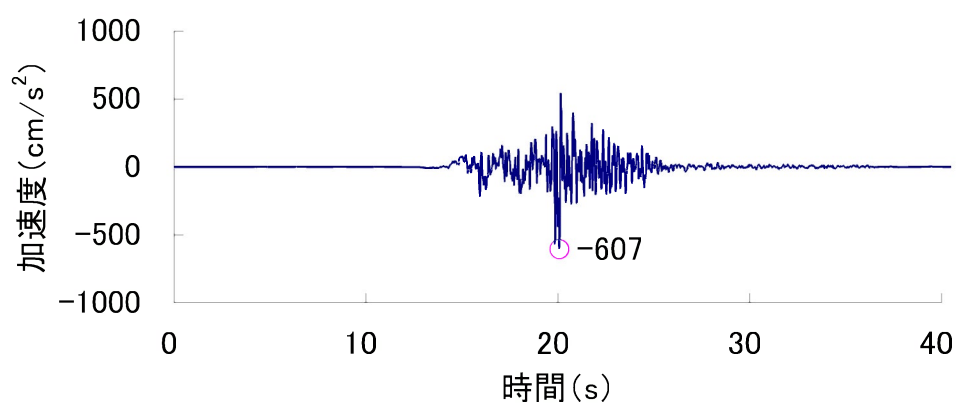
Ss-17 (EW 方向)
