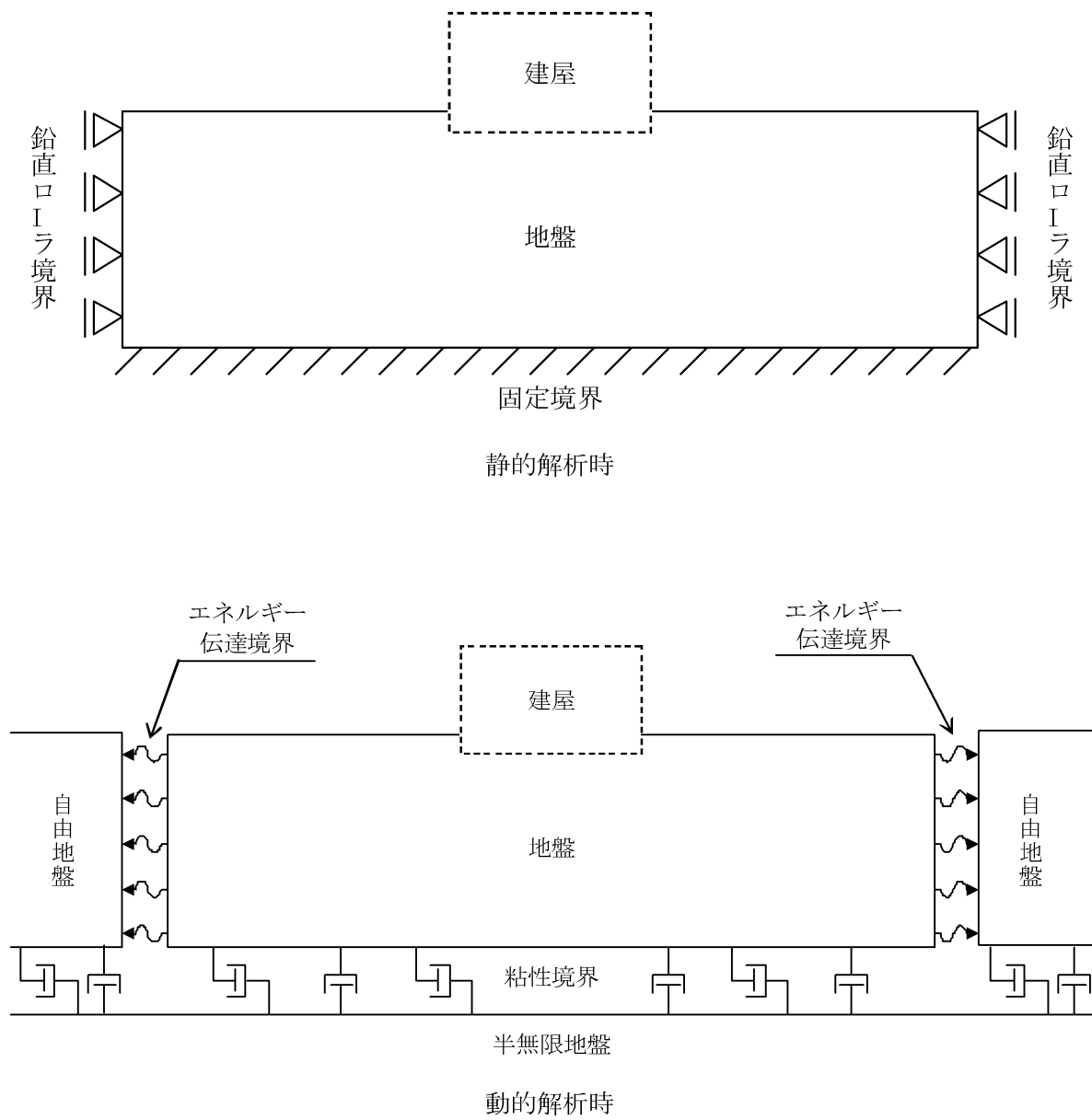
第1.2.3.5.7図 境界条件
