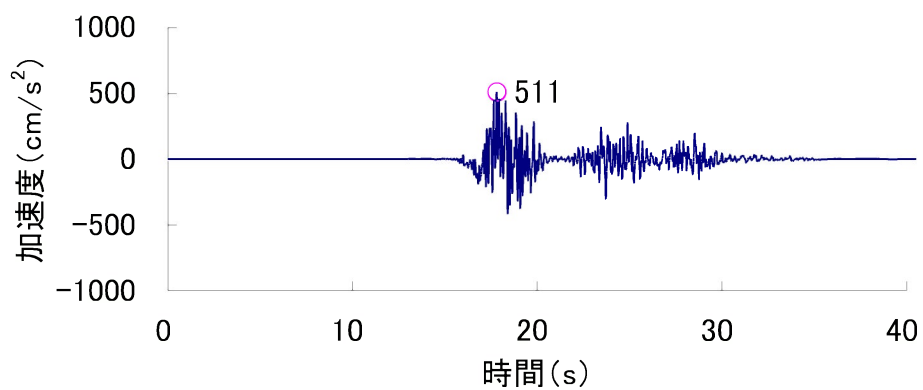
Ss-10 (NS 方向)
