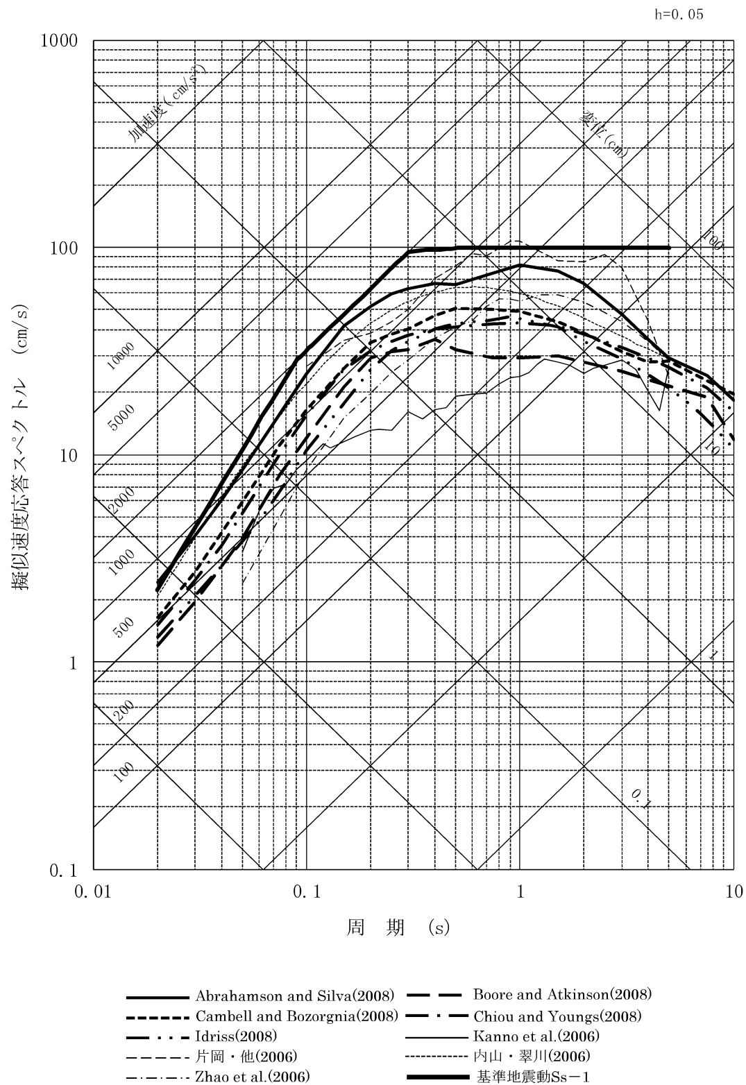
第 1.2.5.6.3 図(2) 基準地震動 Ss-1 の応答スペクトルと各種距離減衰式に基づく地震動評価結果の比較（傾斜角 75° ケース）
