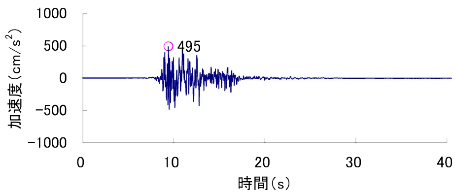
Ss-12 (NS 方向)
