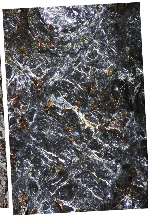
直交ニコル
