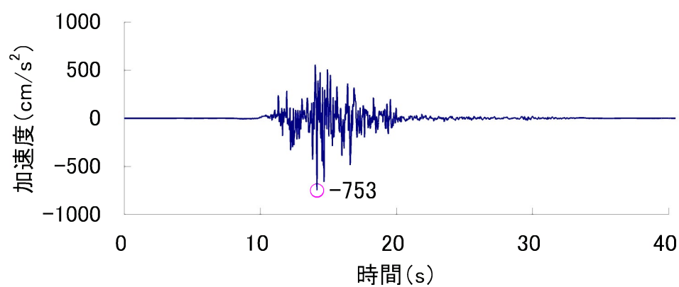
Ss-16 (EW 方向)
