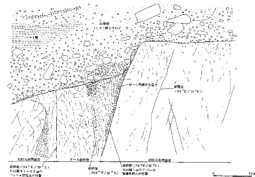
既往トレンチF-6破碎帯詳細スケッチ(北西側側壁基底部)
