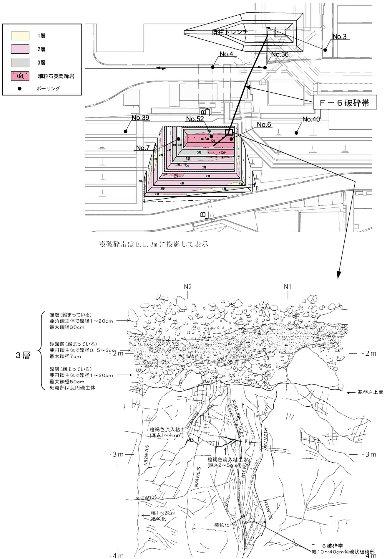
第1.2.3.4.16図 南側トレンチ北壁スケッチ
