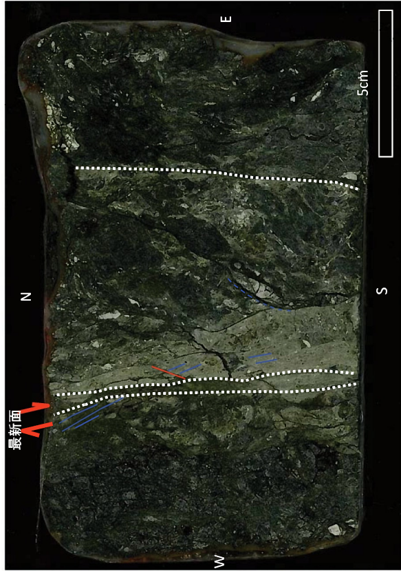
研磨片(横ずれ成分観察用)
