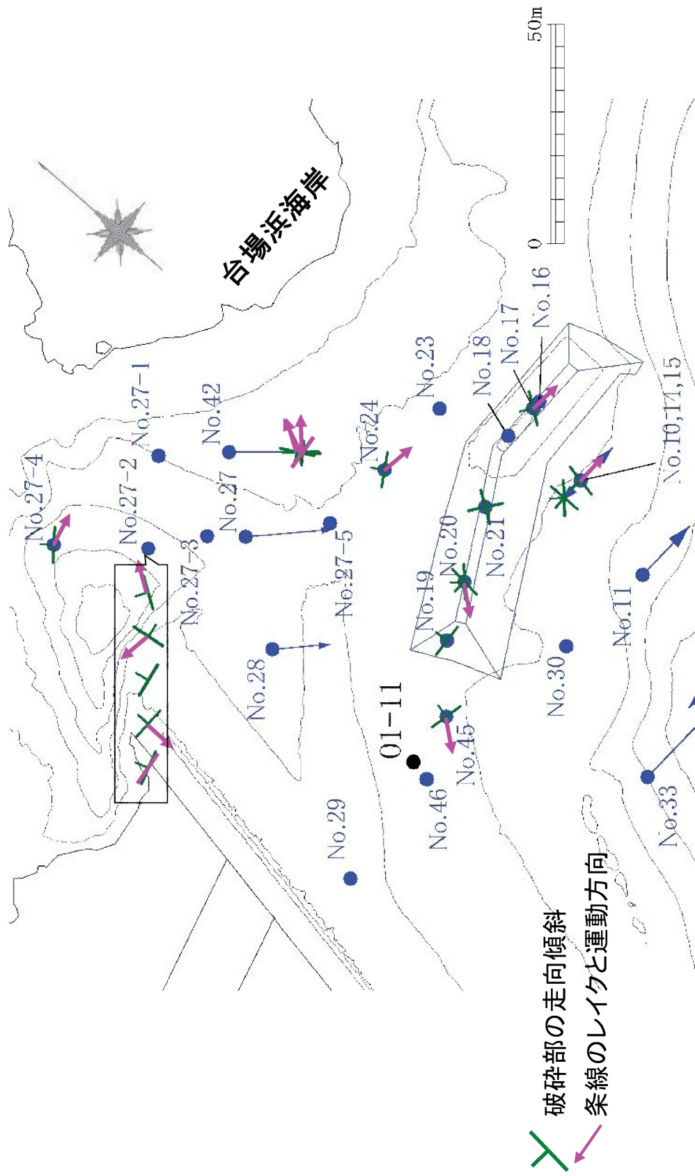
第1.2.3.3.20図 「B.超苦鉄質岩下部の貫入の影響ゾーンで認められる破砕部（主に逆断層センス）」の平面運動方向
