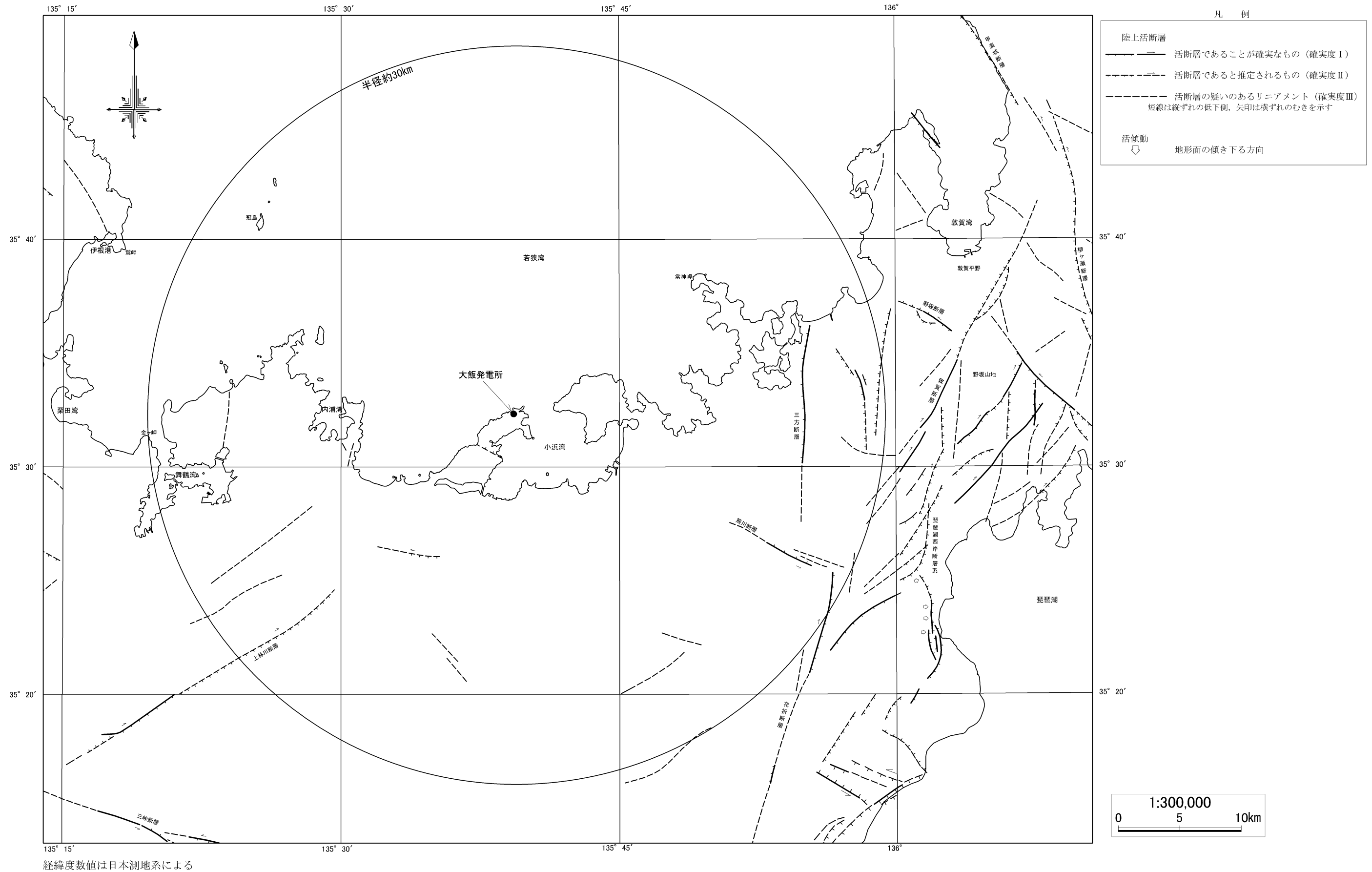
第1.2.3.1.3図 敷地周辺陸域の活断層分布図 「〔新編〕日本の活断層」
