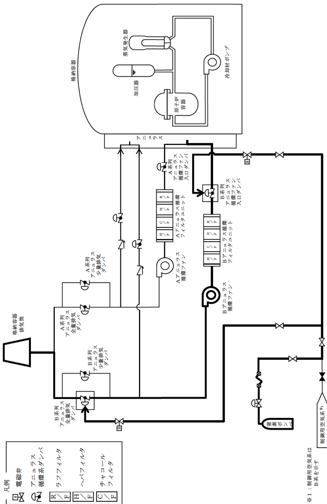
第 1.10.2 図 窒素ポンプ（アニュラス循環系ダンパ作動用）によるアニュラス空気再循環設備の運転 概略系統
