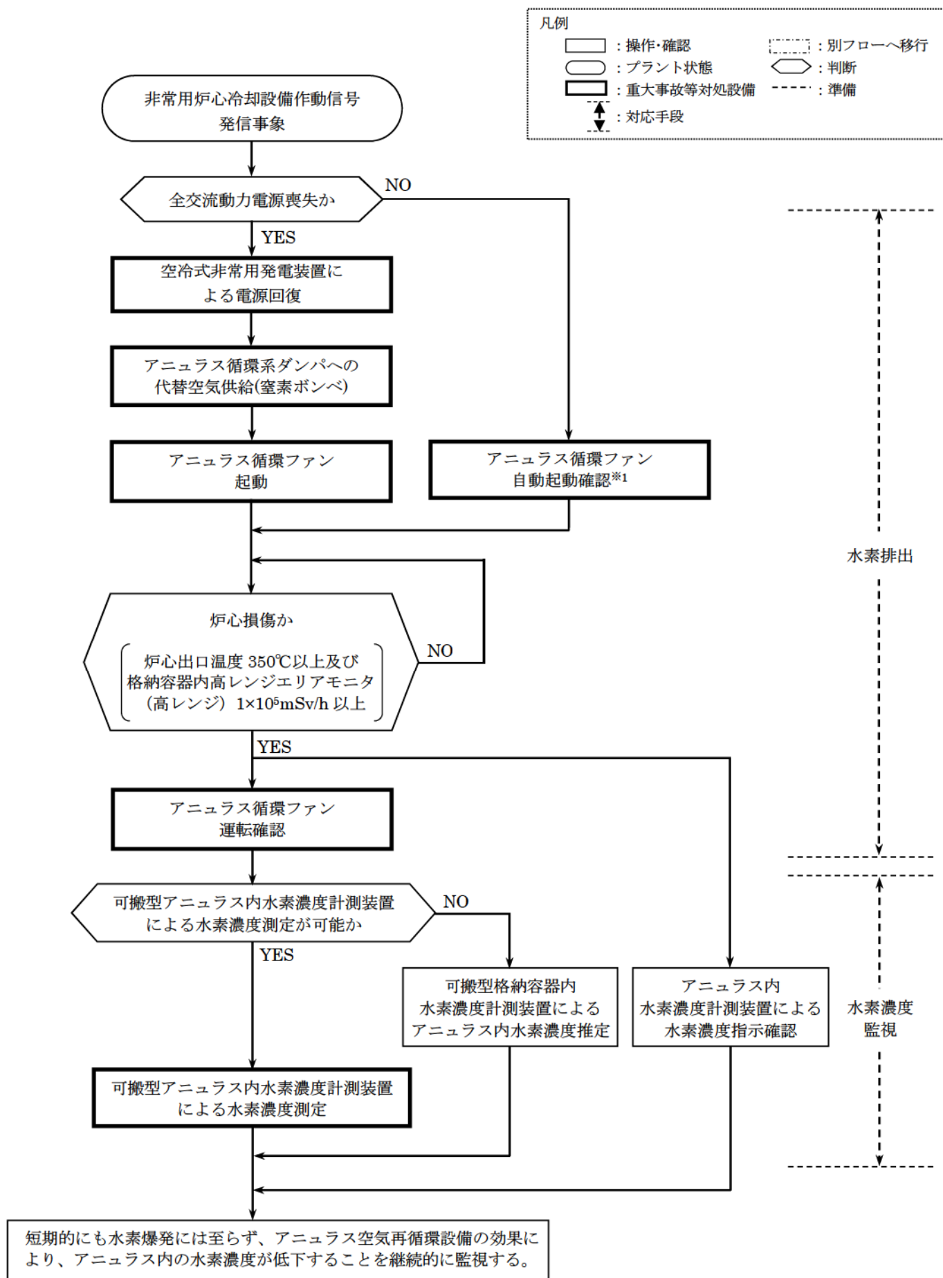
第 1.10.7 図 水素爆発による原子炉建屋等の損傷を防止するための対応手順
