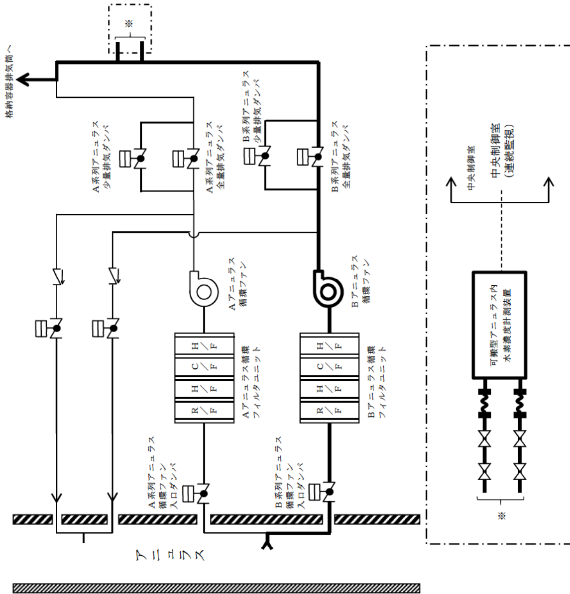
第1.10.4 図 可搬型アニュラス内水素濃度計測装置による水素濃度測定 概略系統
