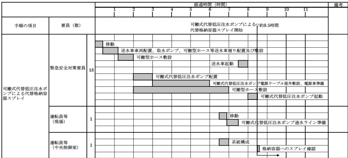
第1.8.13図 可搬式代替低圧注水ポンプによる代替格納容器スプレイ タイムチャート
