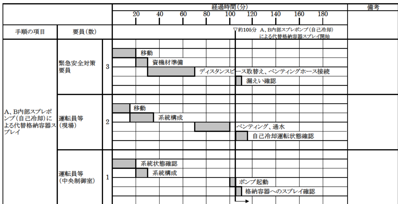
第1.8.16図 A、B内部スプレポンプ(自己冷却)による代替格納容器スプレイ タイムチャート
