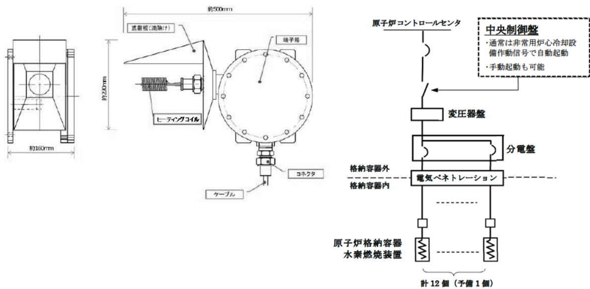
第 1.9.4 図 原子炉格納容器水素燃焼装置構造図
