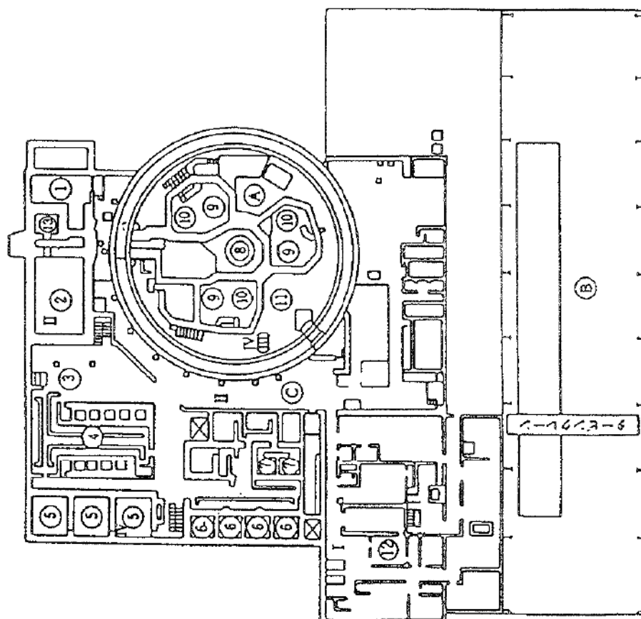
第2.2.4図 遮へい設計区分概略図（4階）
