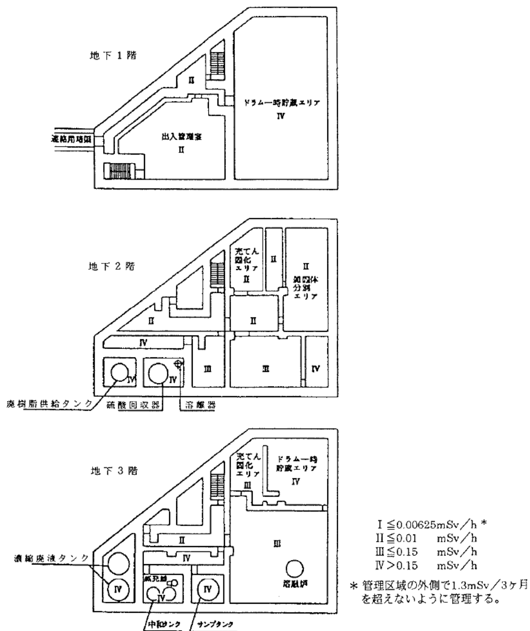
第2.2.8図 遮へい設計区分概略図（第2固体廃棄物処理建屋）（その1）
