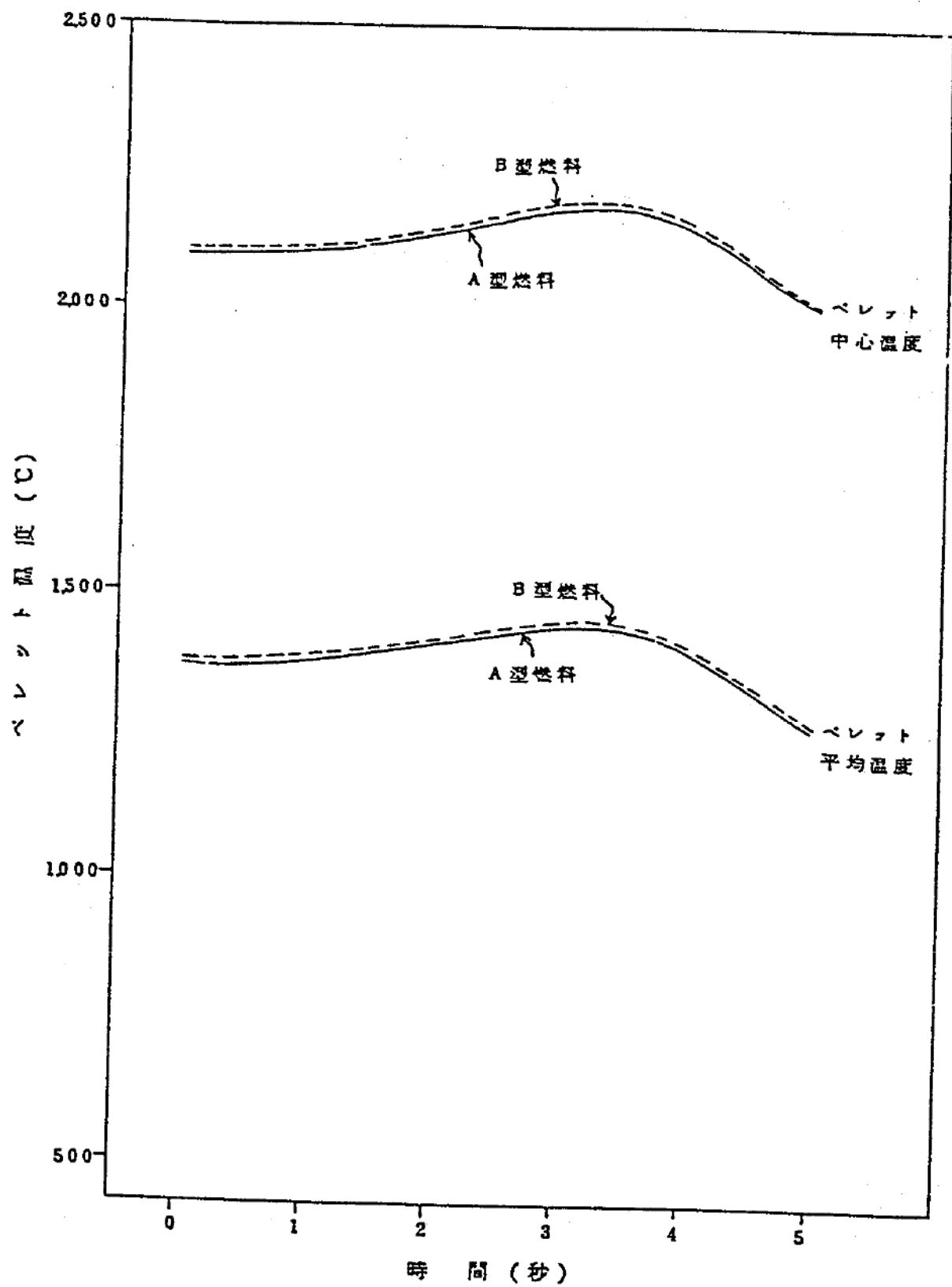
第6図 出力状態からの制御棒クラスタ引抜きの 時のペレット温度の時間変化
