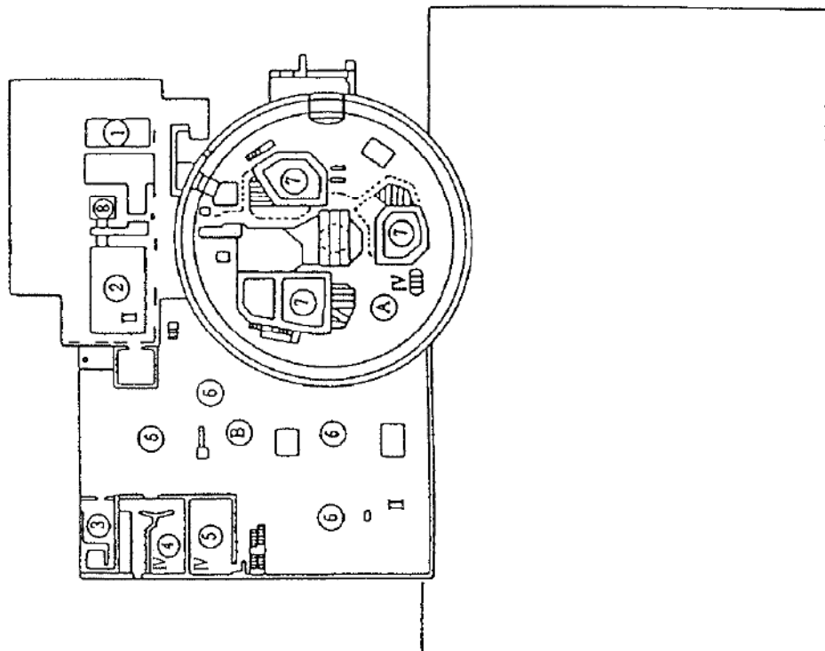
第2.2.5図 遮へい設計区分概略図（5階）
