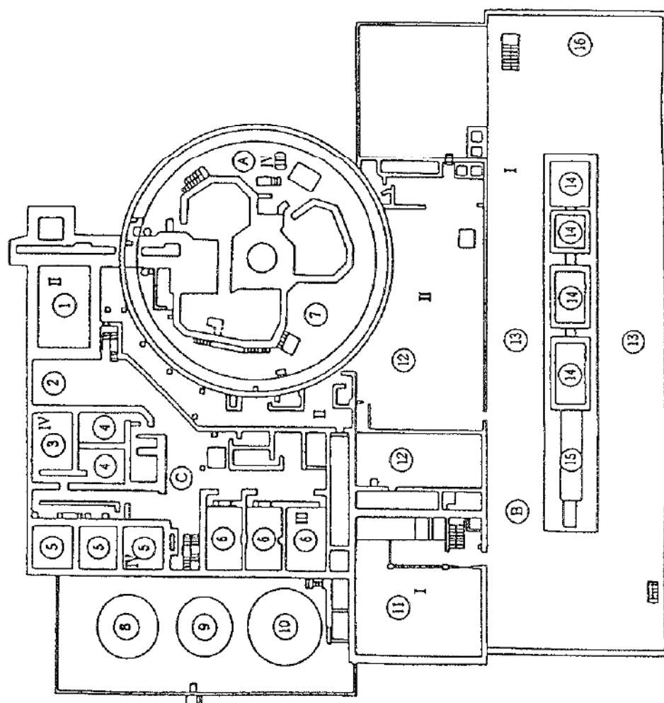
第2.2.3図 遮へい設計区分概略図 (3階)
