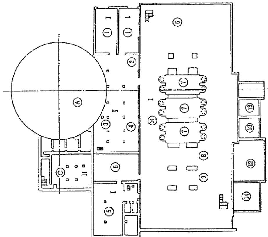
第2.2.1図 遮へい設計区分概略図（1階、地下1階）
