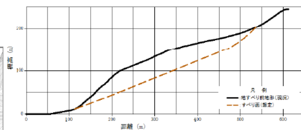
断面2
