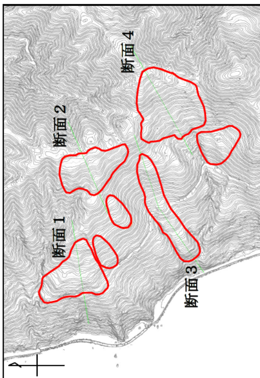
【崩壊範囲】
