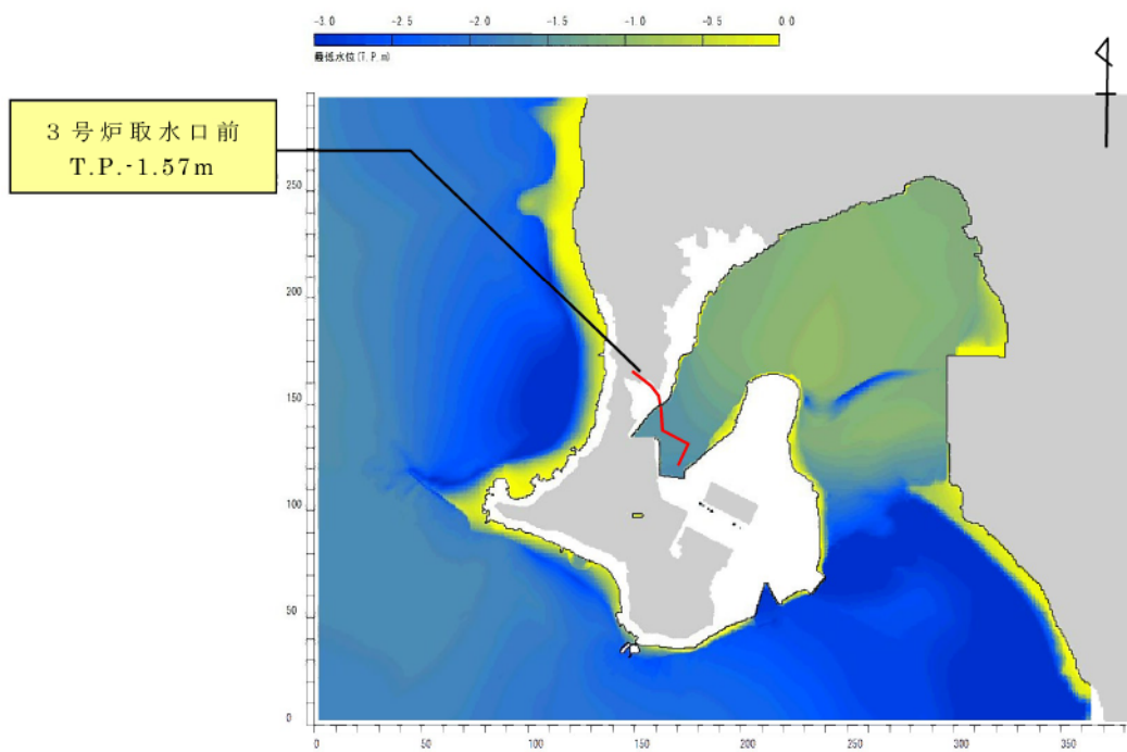
第 6.3.9 図 基準津波 3 による水位分布図
