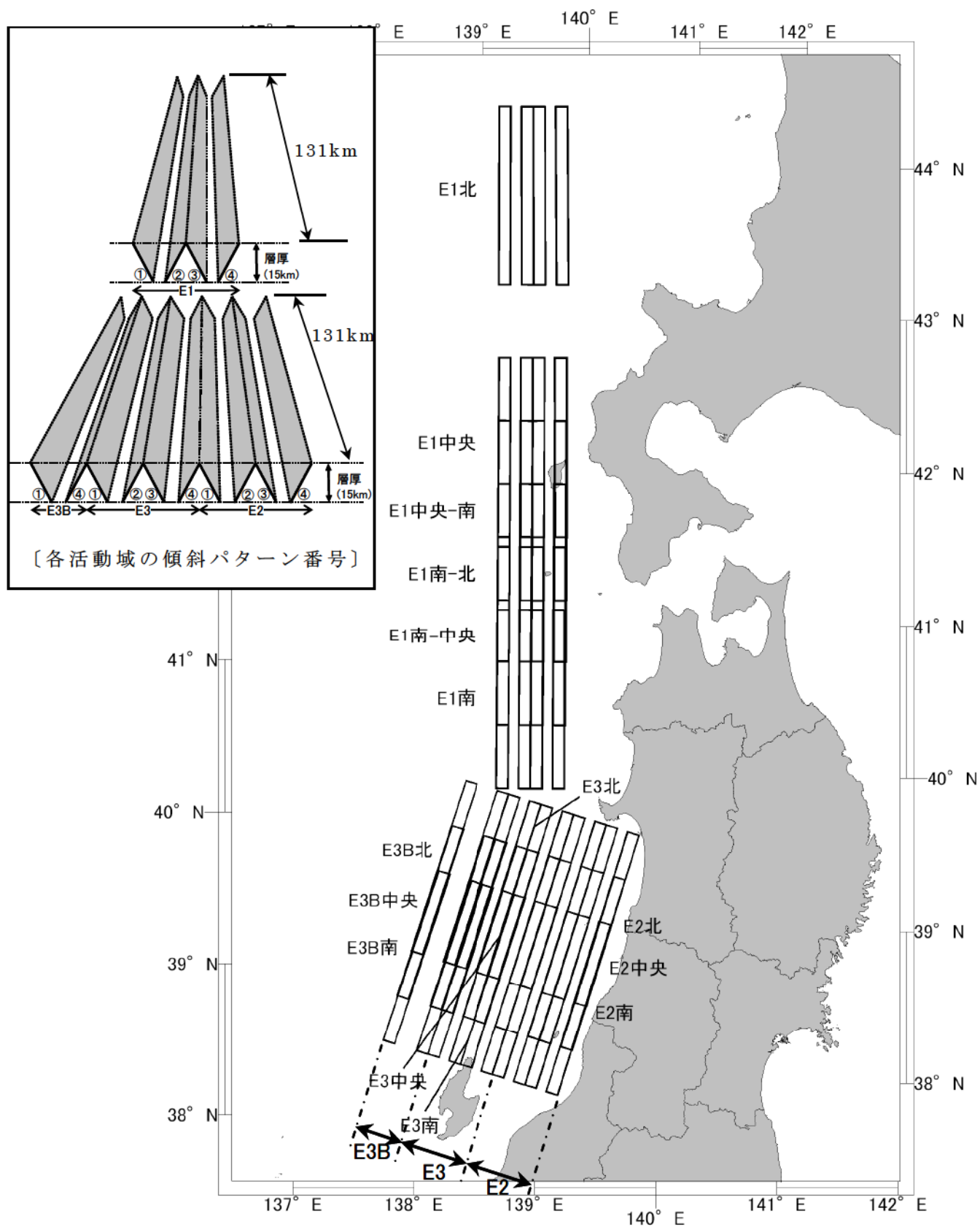
第 6.2.11 図 日本海東縁部における検討対象断層
