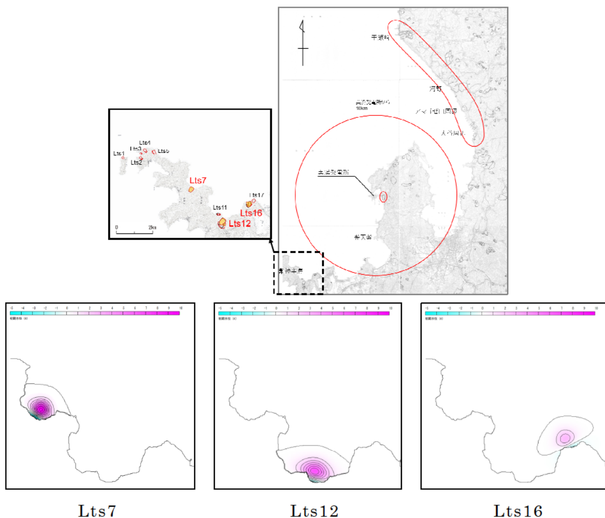
第 6.2.25 図 Watts 他による方法の初期水位波形及び計算条件 (Lts7、Lts12、Lts16)
