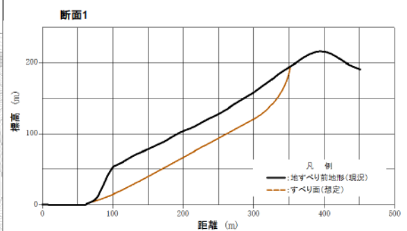
【推定断面図】
