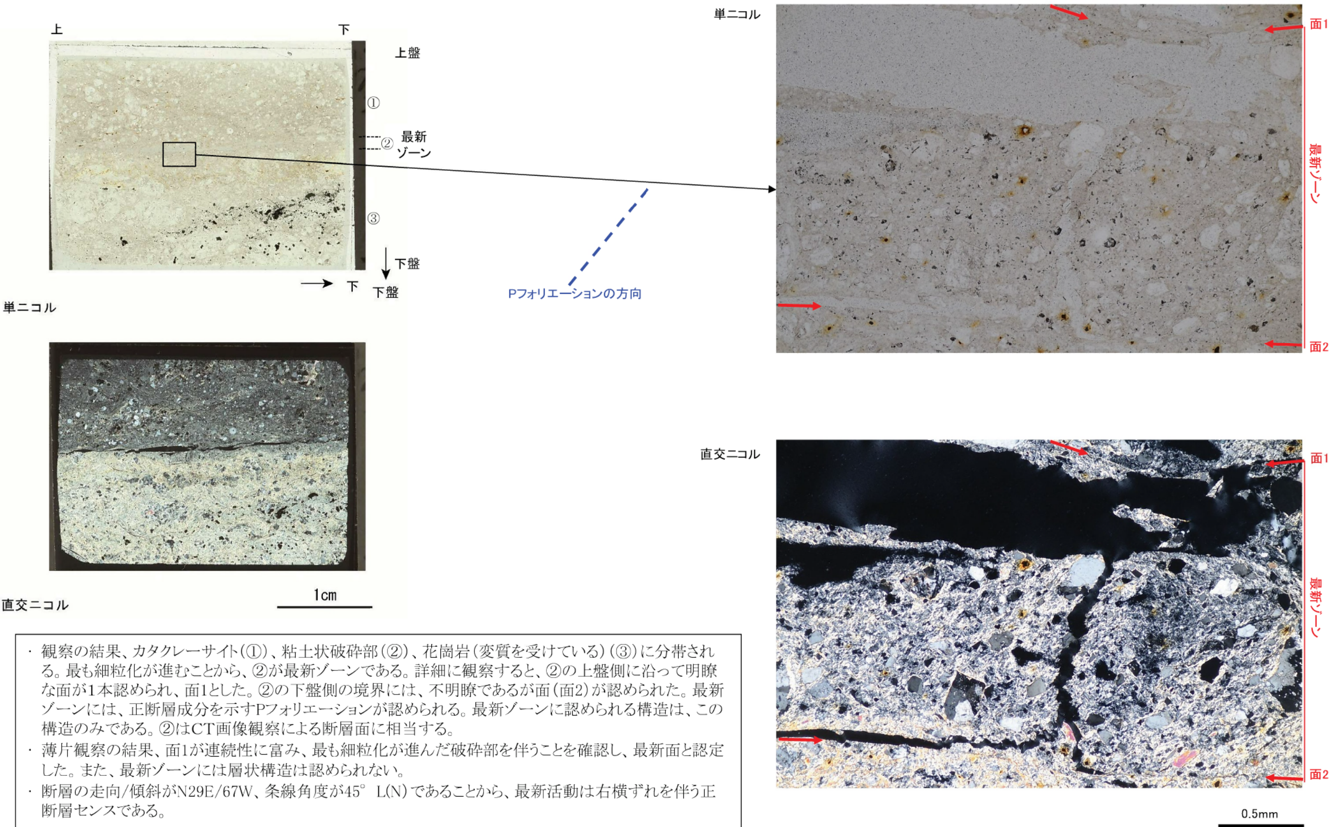
第 1.8.38 図(2) 活動性評価を代表する破砕帯があるその他の破砕部 薄片観察結果(2)
