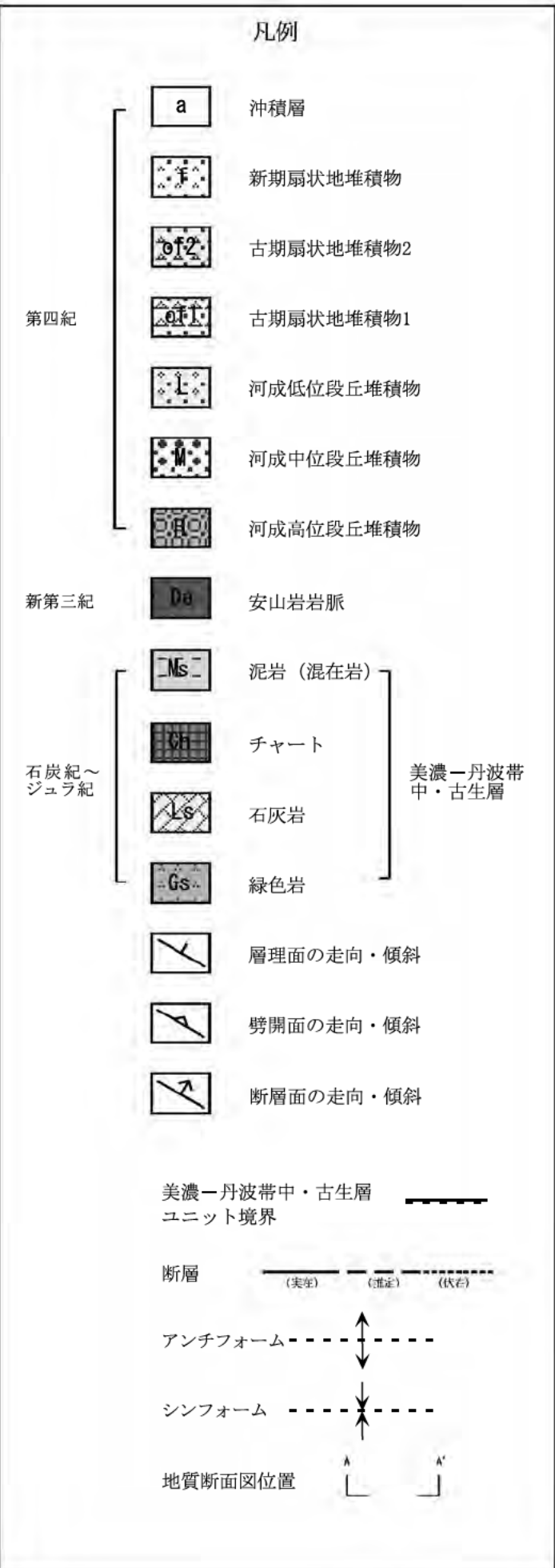
第1. 3. 70図(2) 柳ヶ瀬断層周辺の地質図（その2）
