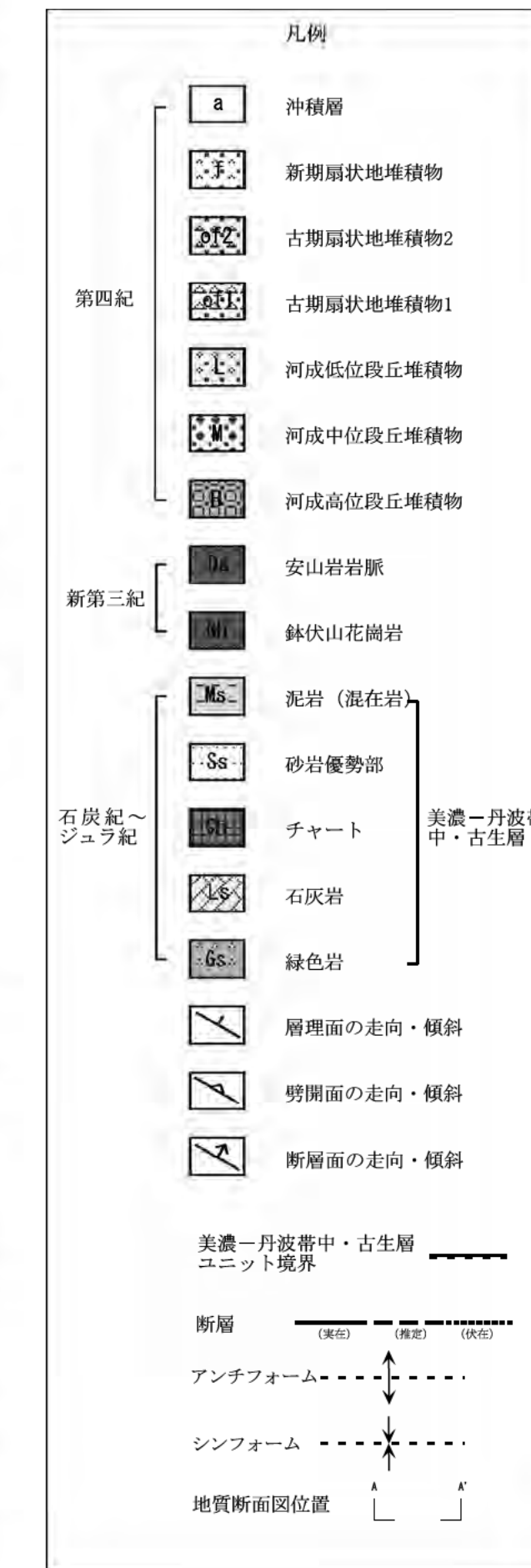
第1.3.70図(1) 柳ヶ瀬断層周辺の地質図 (その1)
