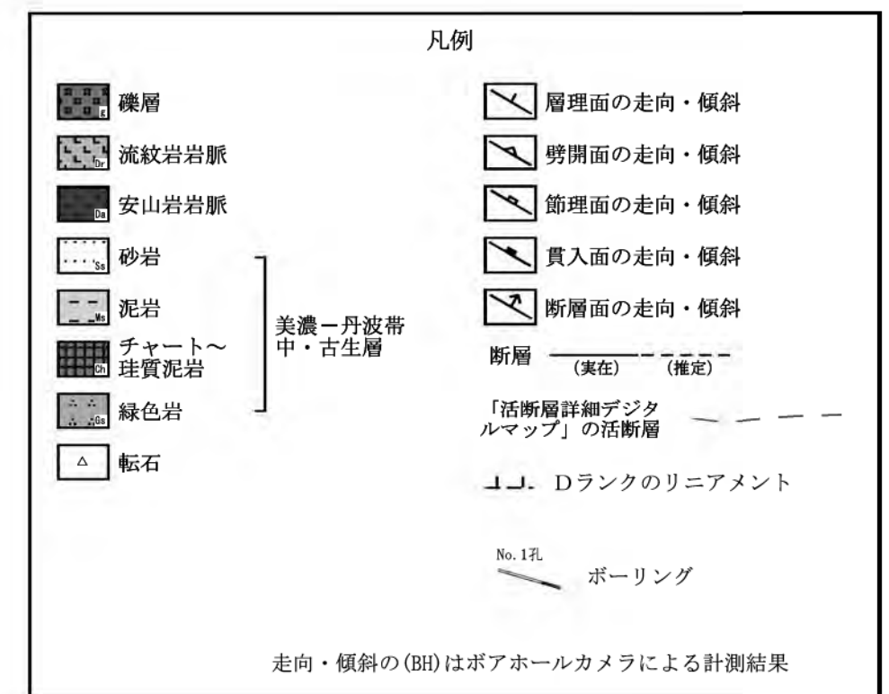
第1.3.72図 柳ヶ瀬断層 ニッ屋南西方付近のルートマップ (Loc. Yt-1)
