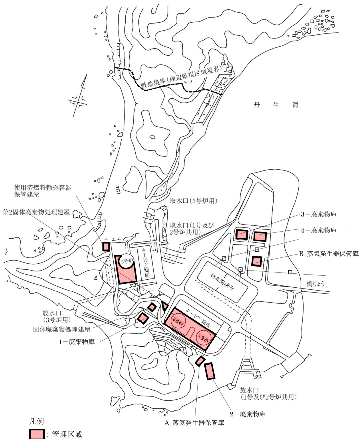
第 4-2 図 廃止措置対象施設の管理区域全体図 (1 号炉の廃止措置対象施設を含む。)
