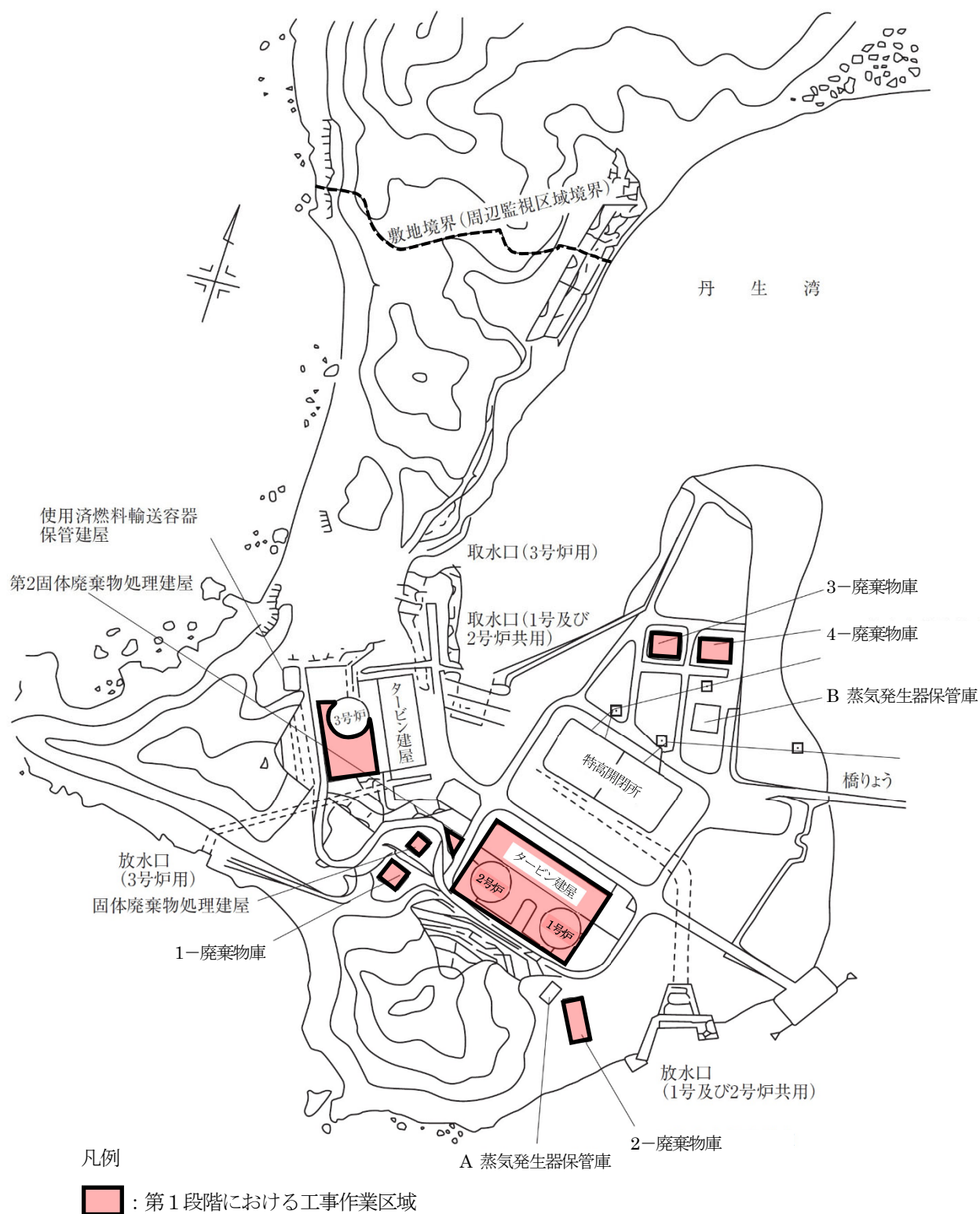
第1図 廃止措置対象施設の敷地及び廃止措置（第1段階）に係る 工事作業区域（1号炉の工事作業区域を含む。）
