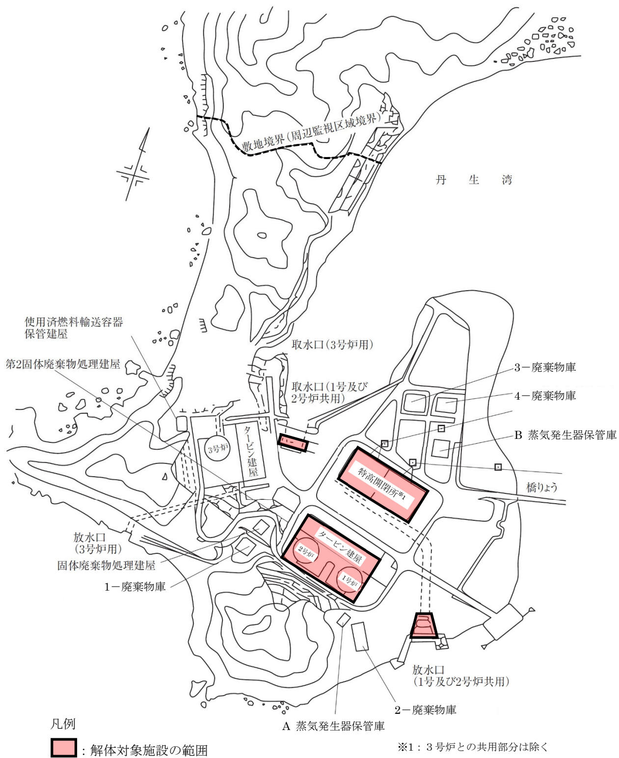
第5-1図 解体対象施設の範囲（1号炉の解体対象施設を含む。）
