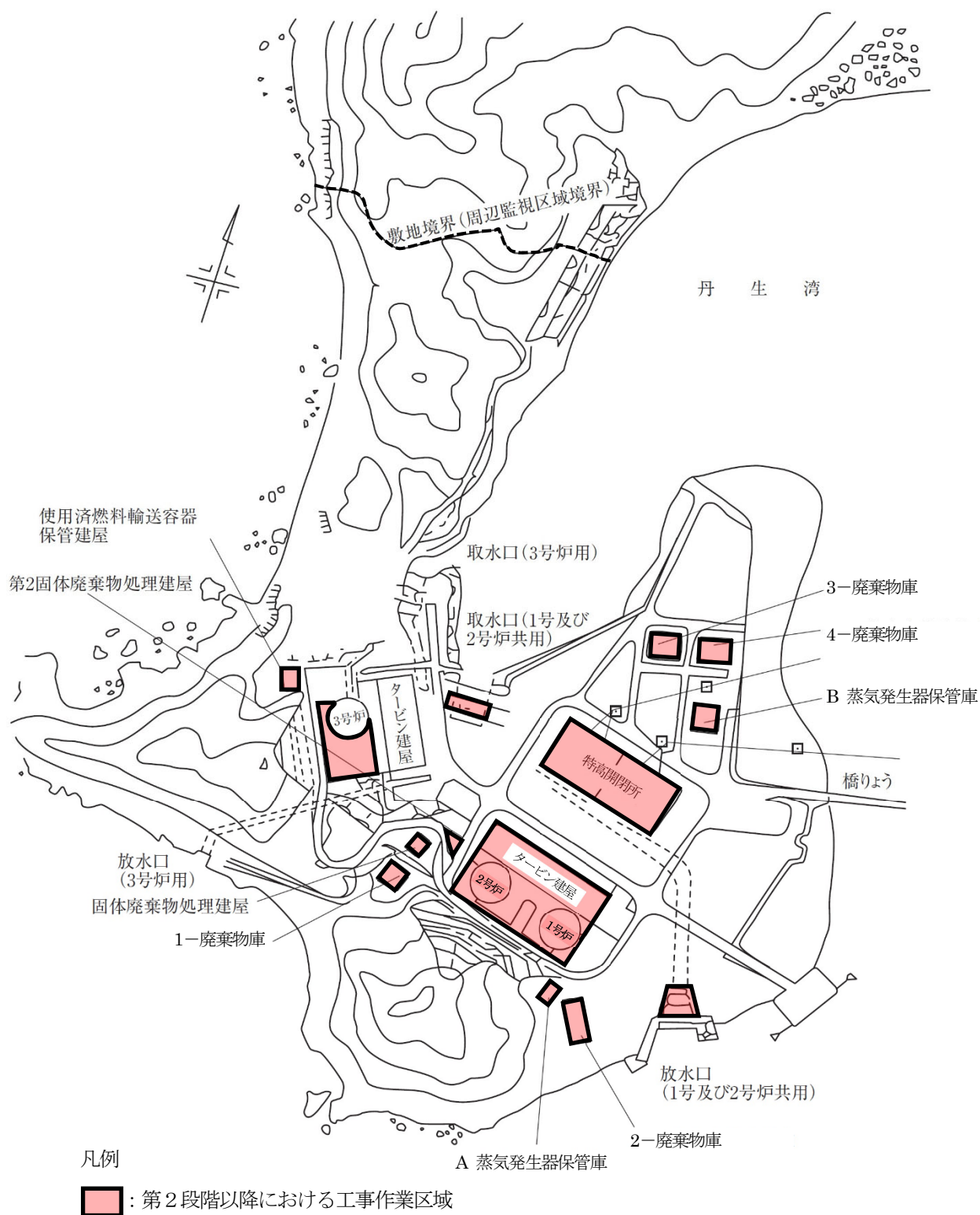
第2図 廃止措置対象施設の敷地及び廃止措置(第2段階以降) に係る工事作業区域(1号炉の工事作業区域を含む。)
