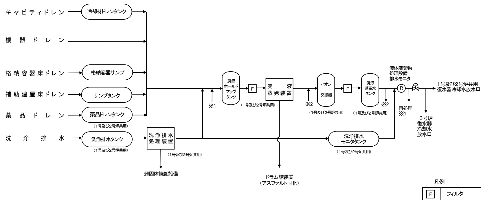
第 10-4 図 第 2 段階以降における放射性液体廃棄物の処理流路線図（1 号炉及び 2 号炉）
