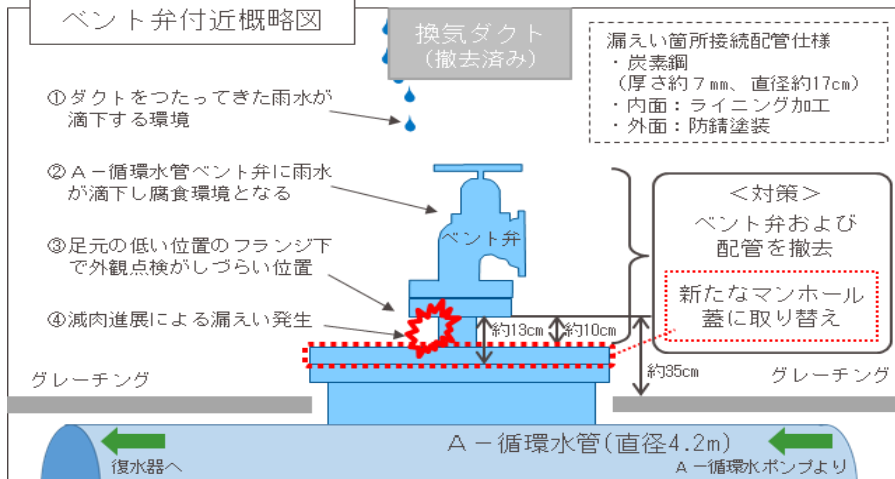
ベント弁付近概略図
