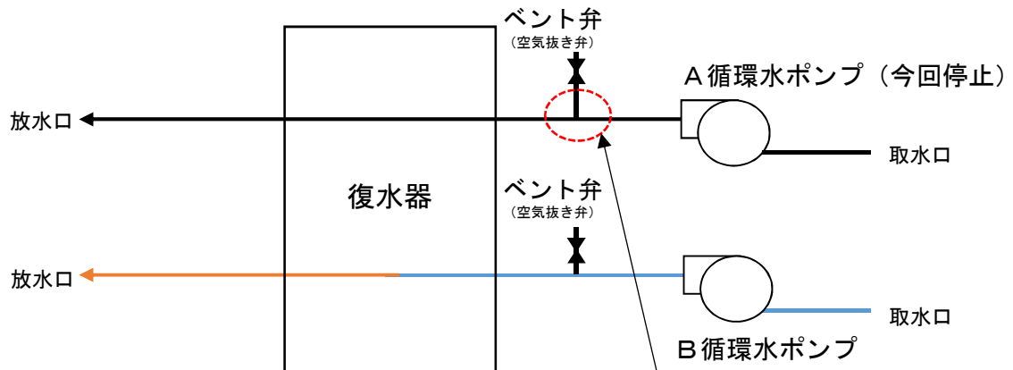
復水器系統概略図
