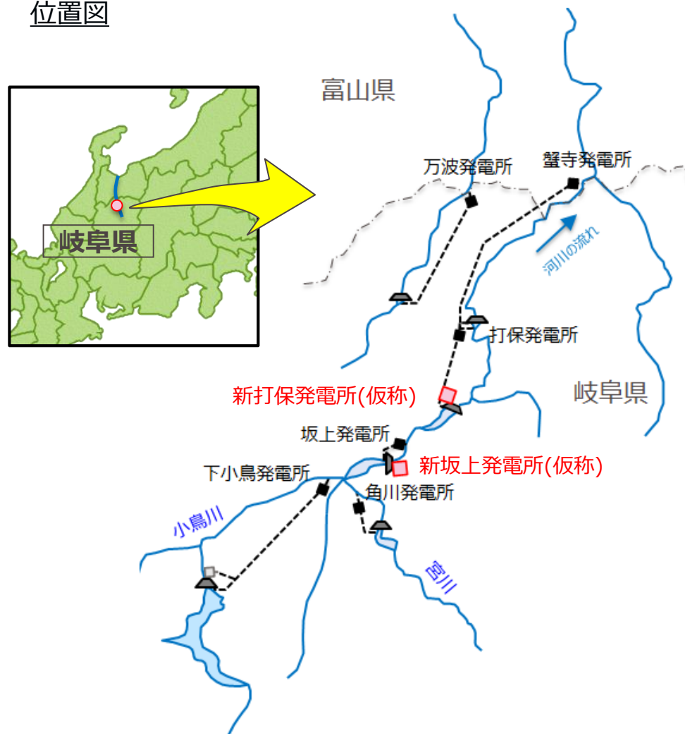
神通川水系発電所模式図
