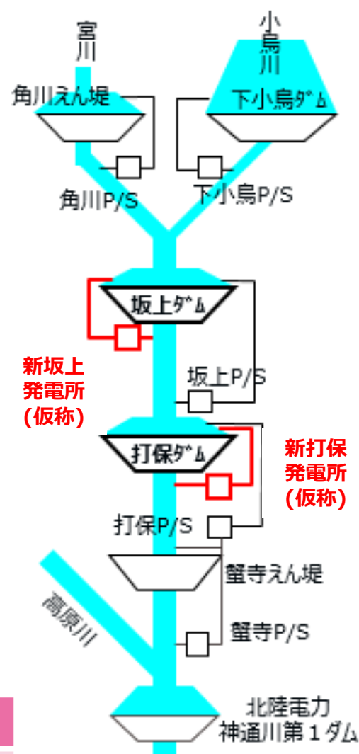
神通川水系発電所模式図
