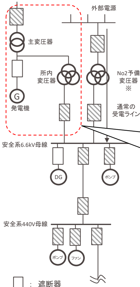
<電源系統構成(イメージ)>
