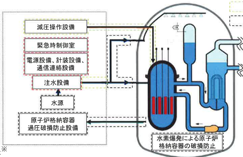
【特定重大事故等対処施設の主な設備の概要図】
