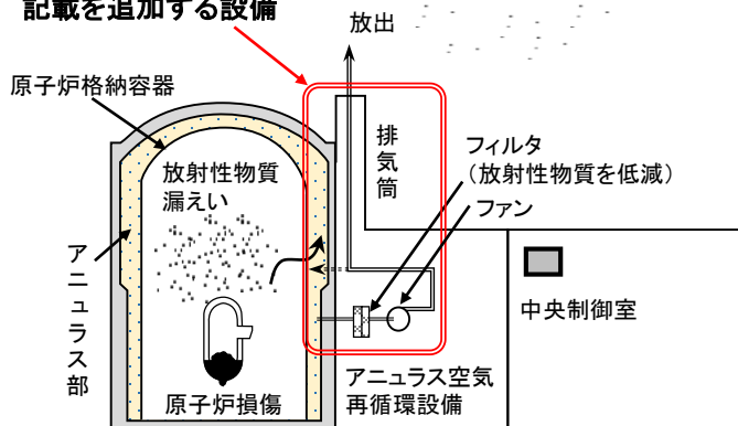
美浜発電所3号機 中央制御室の居住性確保に関するイメージ図
