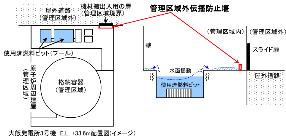
管理区域外伝播防止堰(断面図)
