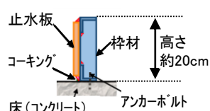
管理区域外伝播防止堰(断面図)
