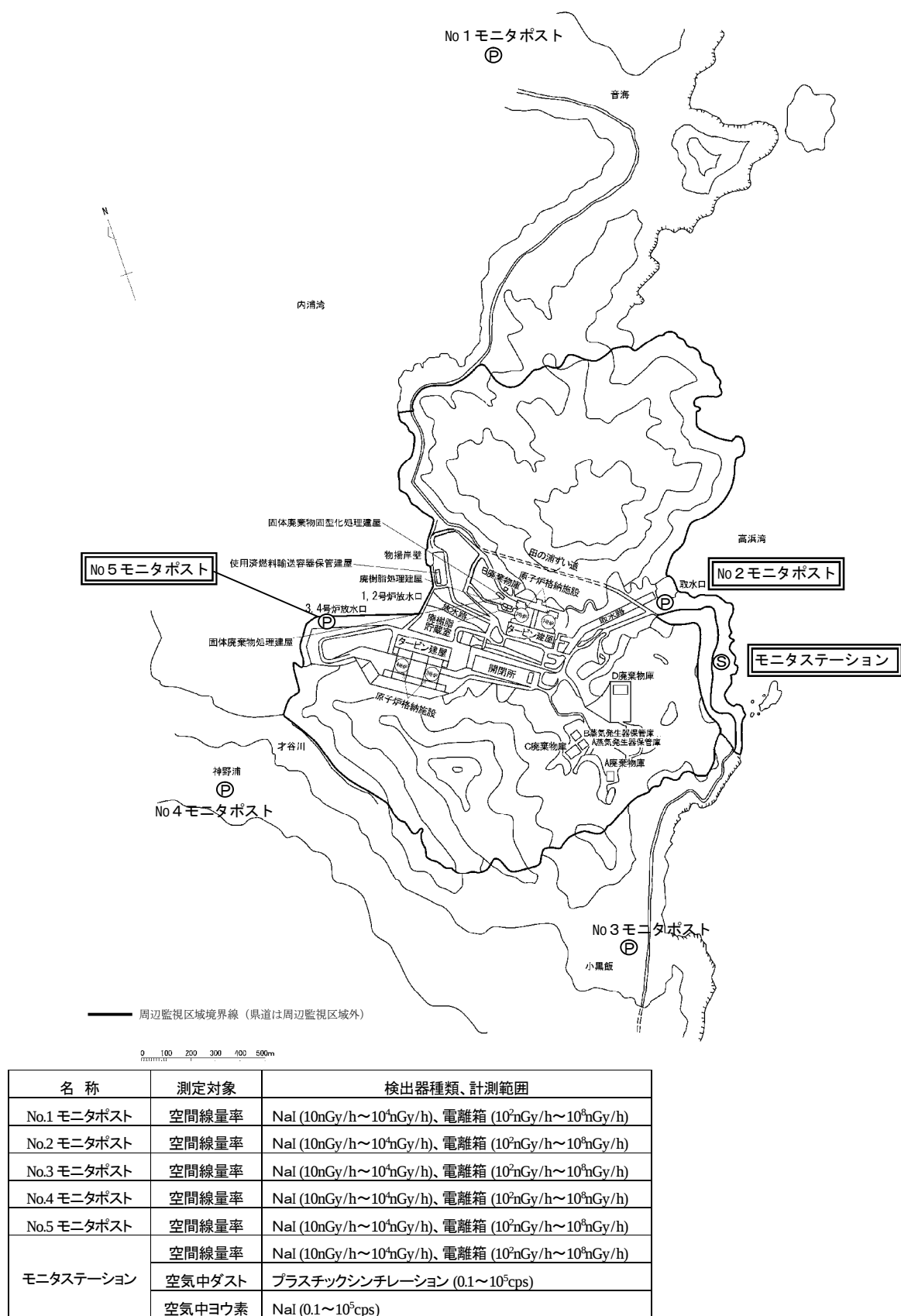
別図 2-3-13 発電所敷地周辺の放射線測定設備
