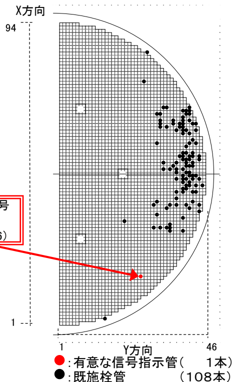
A-蒸気発生器(高温側)上部より見た伝熱管位置を示す図
