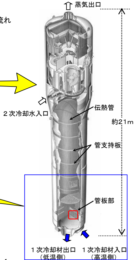
蒸気発生器の概要図
