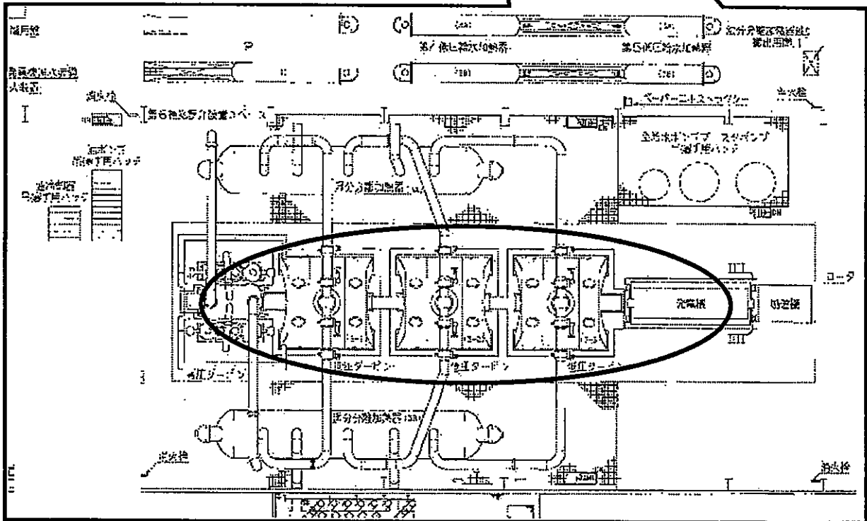
3号機 タービン建屋 EL21.8m タービン
