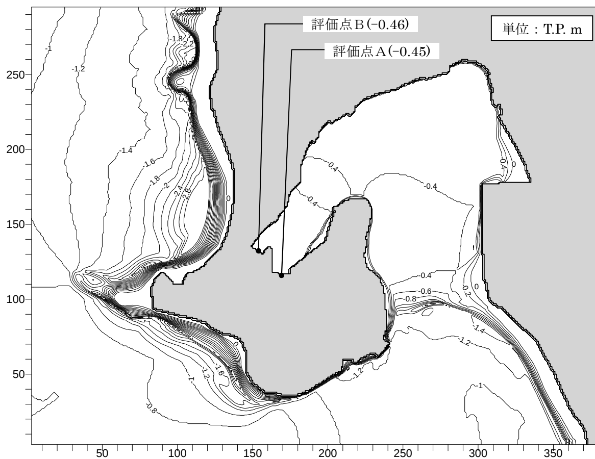
第 3-11 図 水位下降の最大水位分布 (水位下降側: C 断層 [傾斜角 55°, 広域応力場 100°, 上縁深さ 0km])
