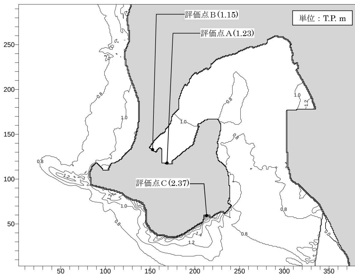
第 3-7 図 最大水位上昇量の分布 (水位上昇側：白木－丹生断層 [広域応力場 100^\circ , 上縁深さ 0km])
