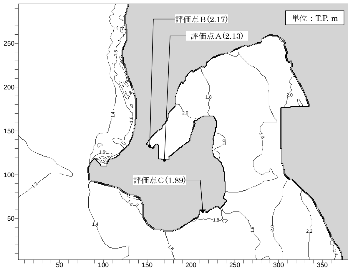
第 3-5 図 最大水位上昇量の分布
