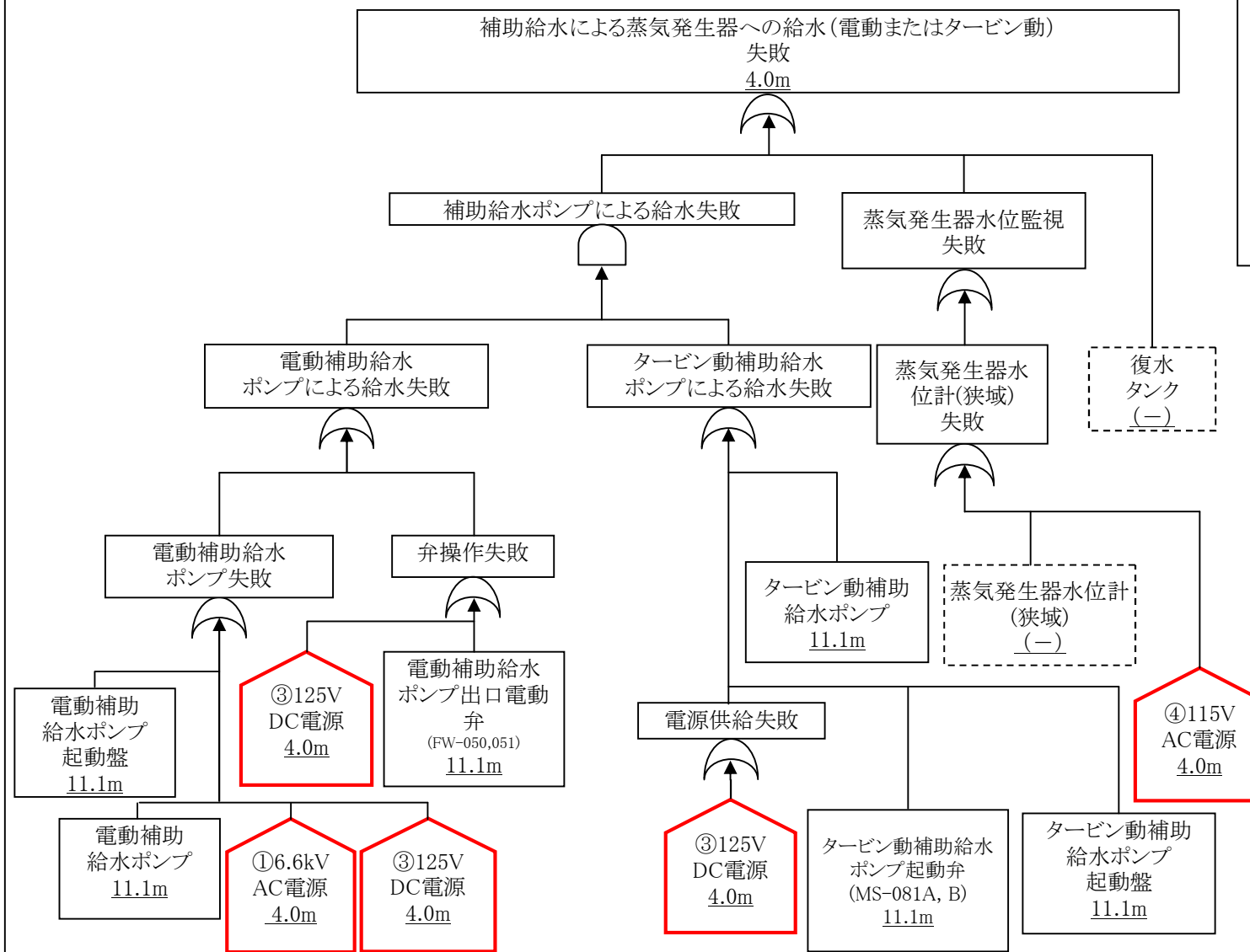
各影響緩和機能のフォールトツリー(津波:炉心損傷)
