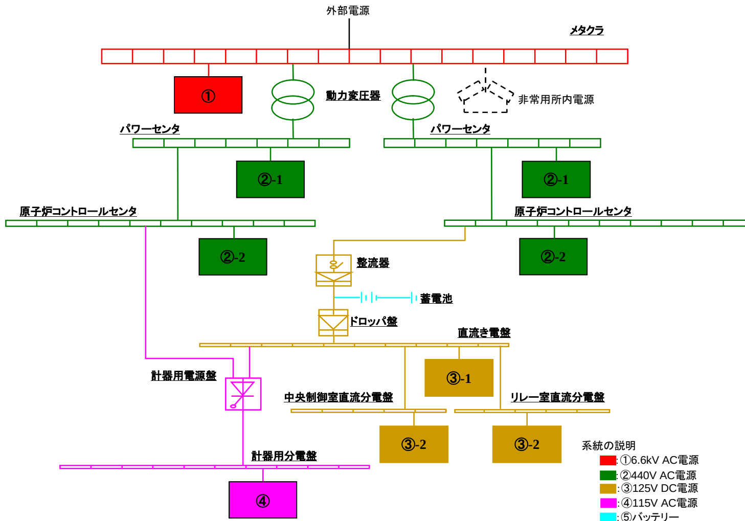
各影響緩和機能の系統図(津波:SFP燃料損傷)
