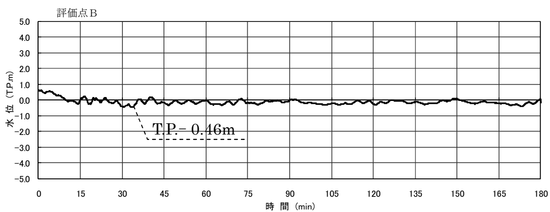
第 3-12 図 代表地点位置における水位の時系列変化 (水位下降側: C 断層 [傾斜角 55°, 広域応力場 100°, 上縁深さ 0km])
