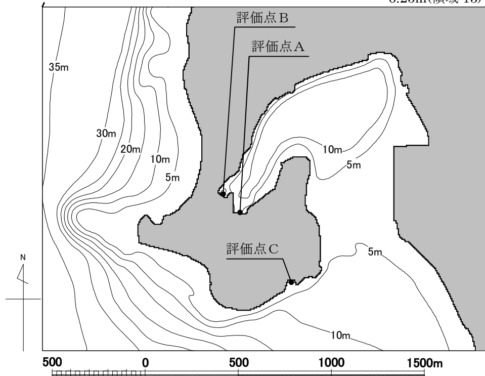
第 3-4 図 詳細格子分割の数値計算モデル
