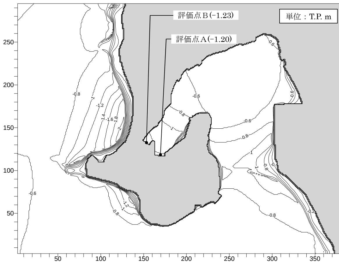
第 3-9 図 最大水位下降量の分布
