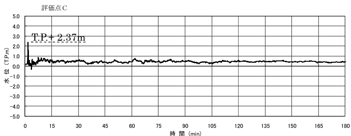
第 3-8 図 代表地点位置における水位の時系列変化 (水位上昇側：白木－丹生断層 [広域応力場 100^\circ , 上縁深さ 0km])
