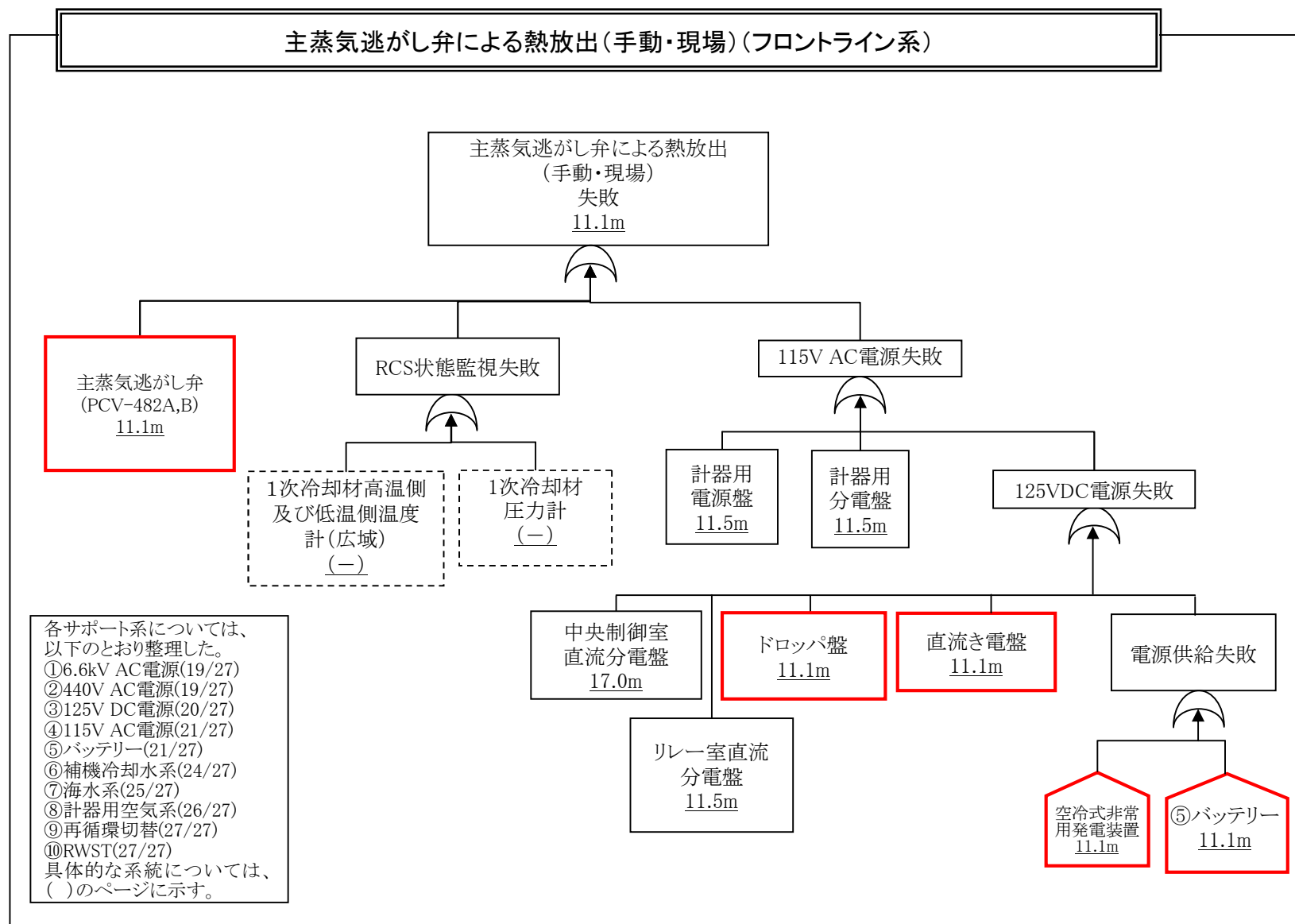
各影響緩和機能のフォールトツリー(津波:炉心損傷)
