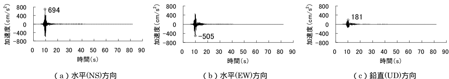
図10 基準地震動Ss - 5の加速度時刻歴波形
