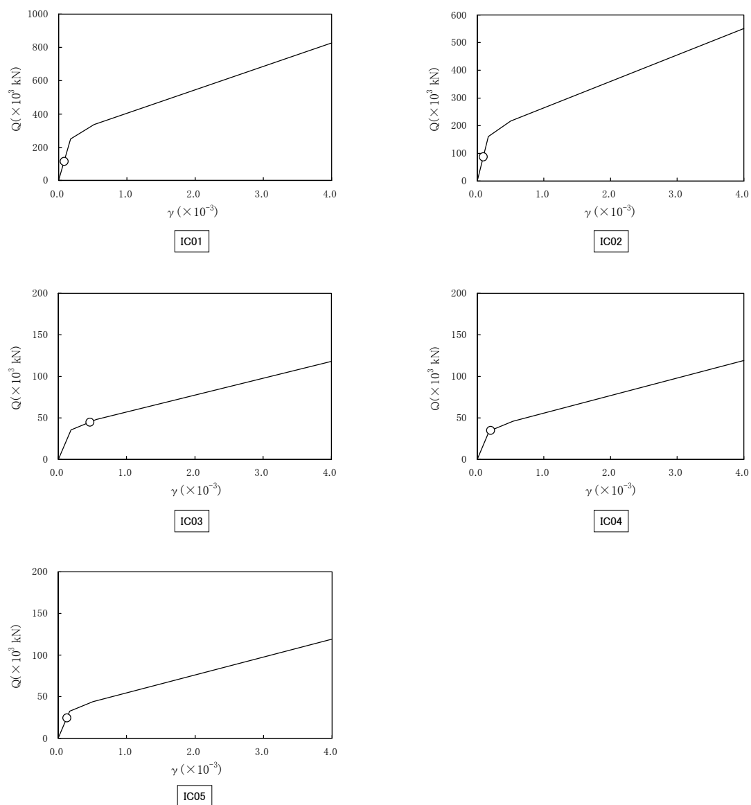
図 2 - 7 - 4 Q- \gamma 関係と最大応答値 (原子炉建屋 I/C S S-1 NS 方向)
