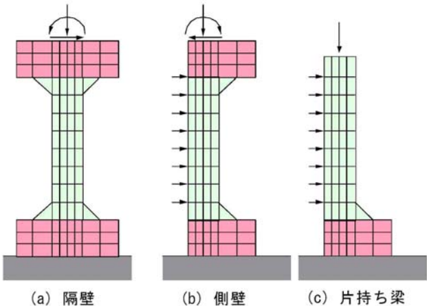
解析モデルと外力設定の例
