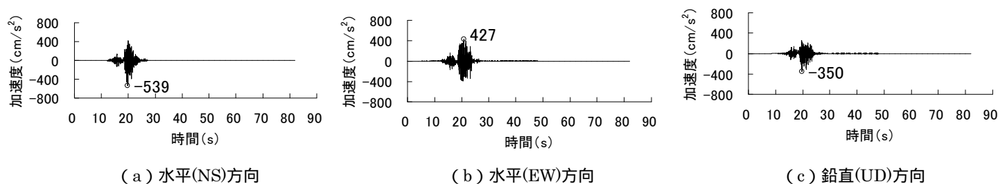
図11 基準地震動Ss - 6の加速度時刻歴波形
