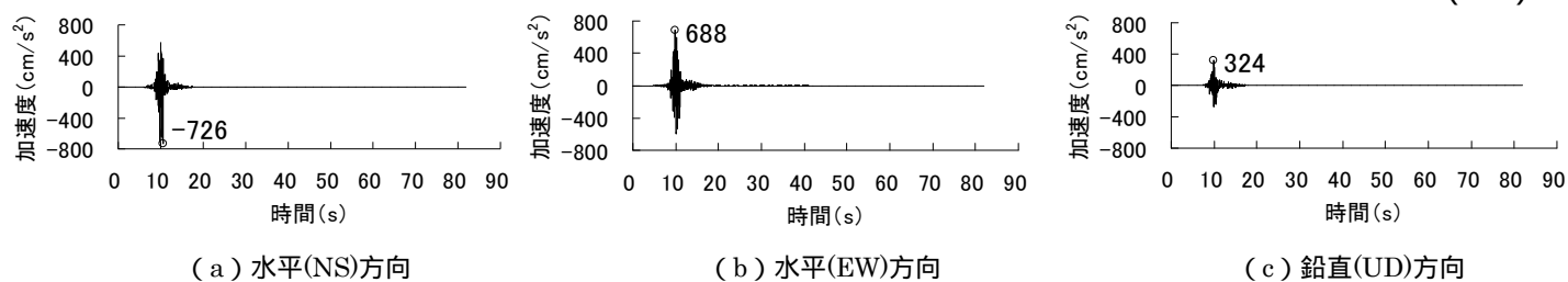
図9 基準地震動Ss - 4の加速度時刻歴波形
