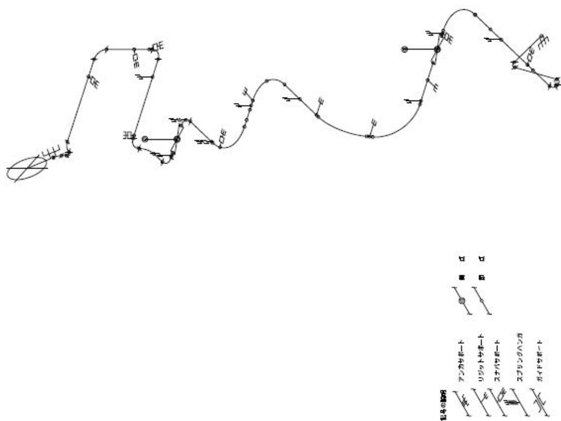
図 3 - 6 地震応答解析モデル（配管系の例）
