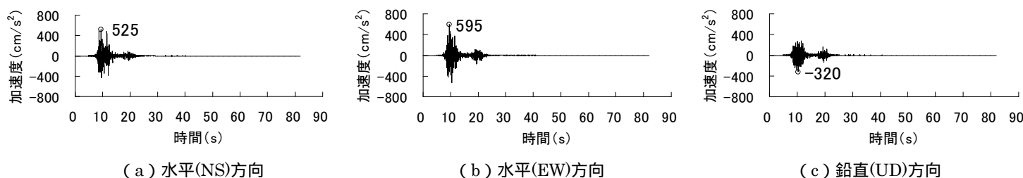
図13 基準地震動Ss - 8の加速度時刻歴波形
