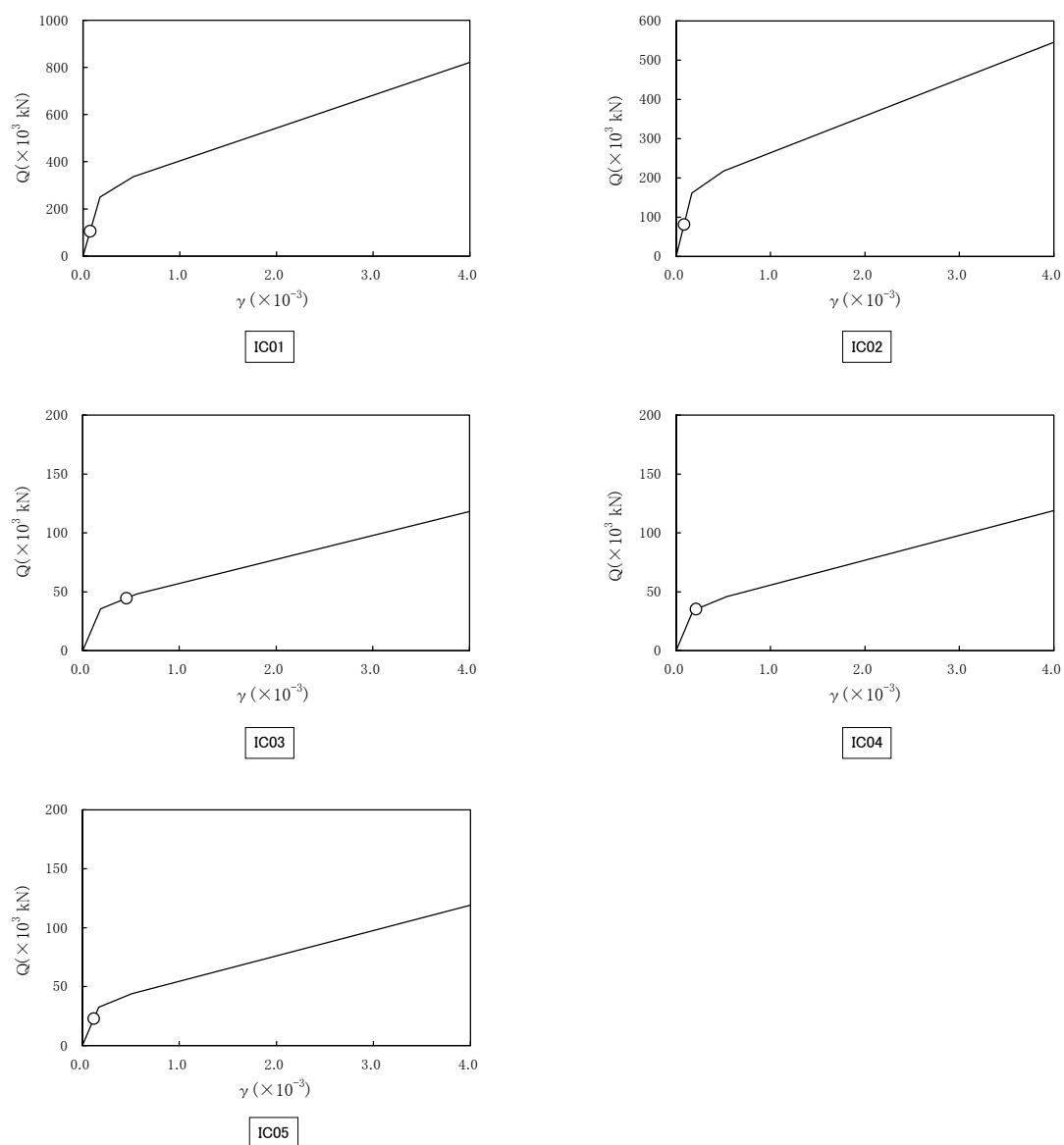
図 2 - 7 - 2 Q- \gamma 関係と最大応答値 (原子炉建屋 I/C S S-1 EW 方向)
