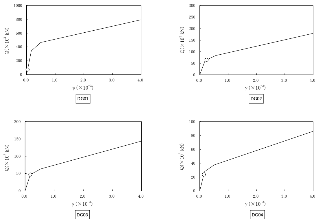
図 2 - 7 - 6 Q - \gamma 関係と最大応答値 (原子炉補助建屋(D/G) S_{S-1} EW 方向)
