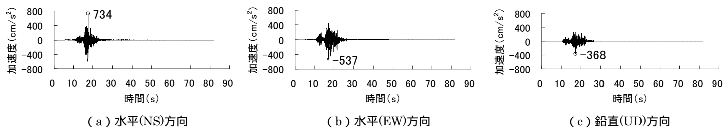
図12 基準地震動Ss - 7の加速度時刻歴波形
