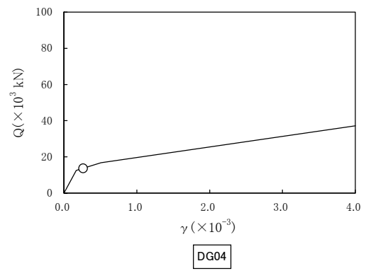
図 2 - 7 - 8 Q- \gamma 関係と最大応答値 (原子炉補助建屋(D/G) S_{S-1} NS 方向)
