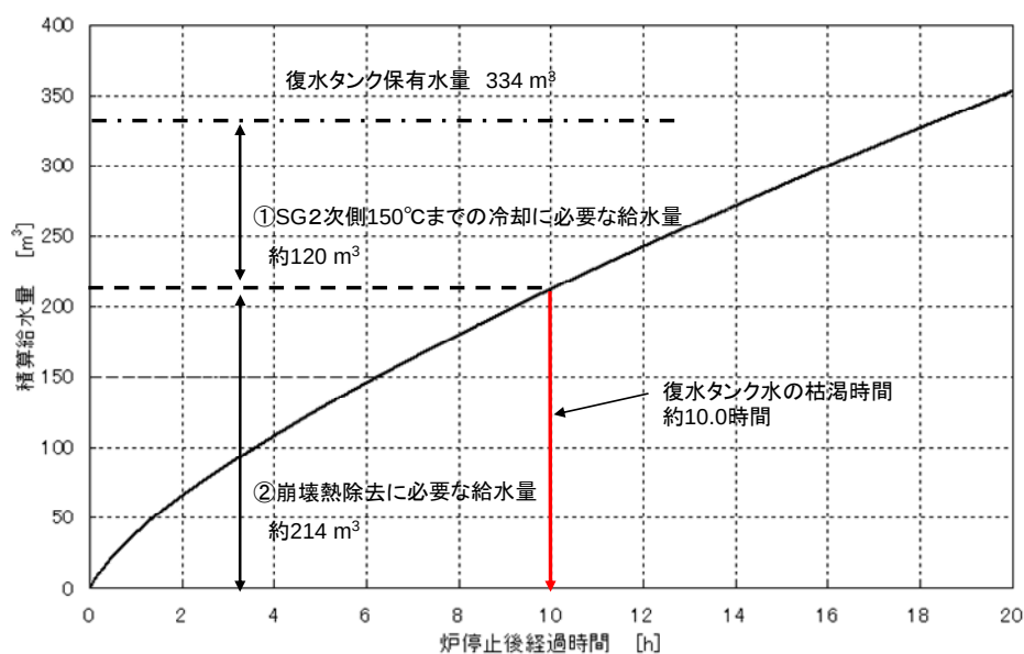
図 5-(6)-8 美浜2号機復水タンク水の枯渇時間評価
