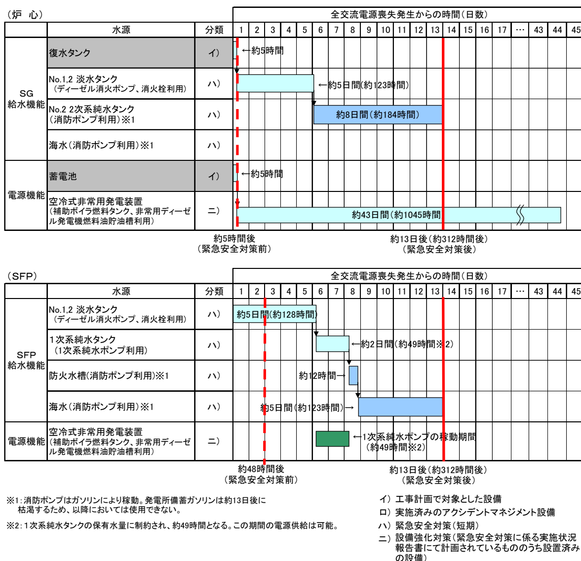
図 5-(4)-10 運転時における事象の過程の進展を防止する措置の効果の評価結果
