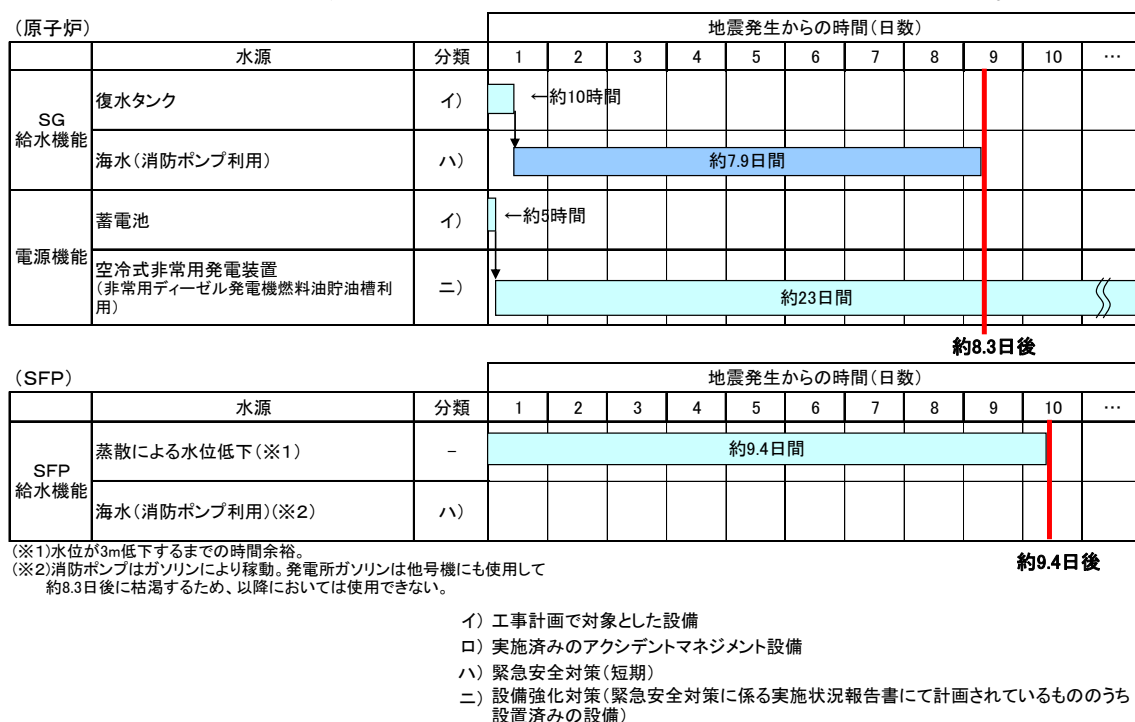
図 5-(6)-12 運転時における給水及び電源機能の継続時間評価結果（地震時）
