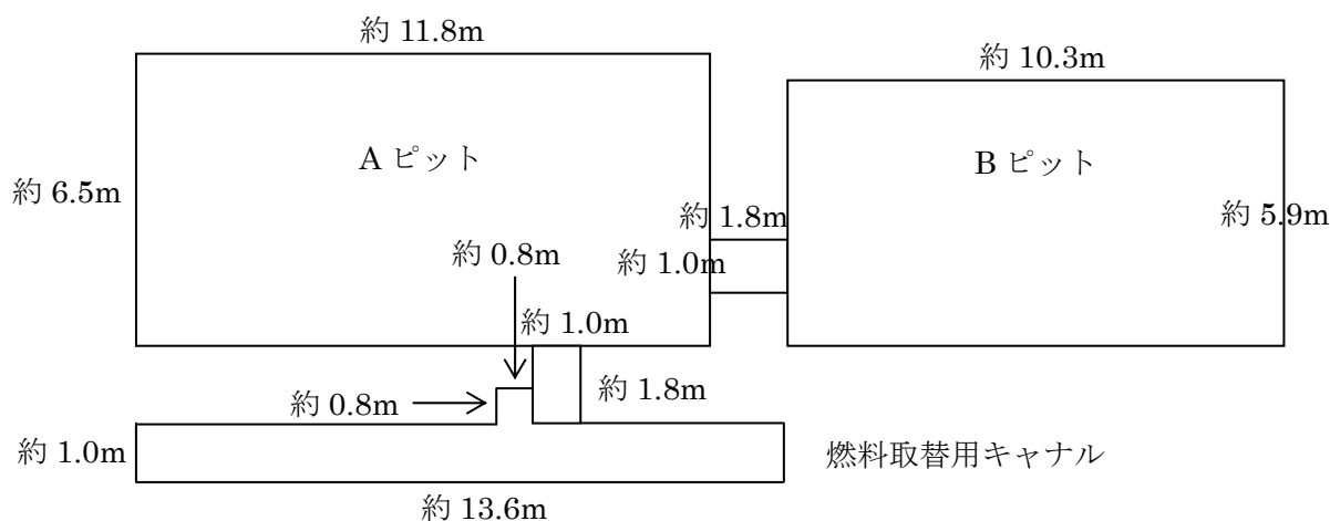
美浜 2 号機使用済燃料ピット概略図
