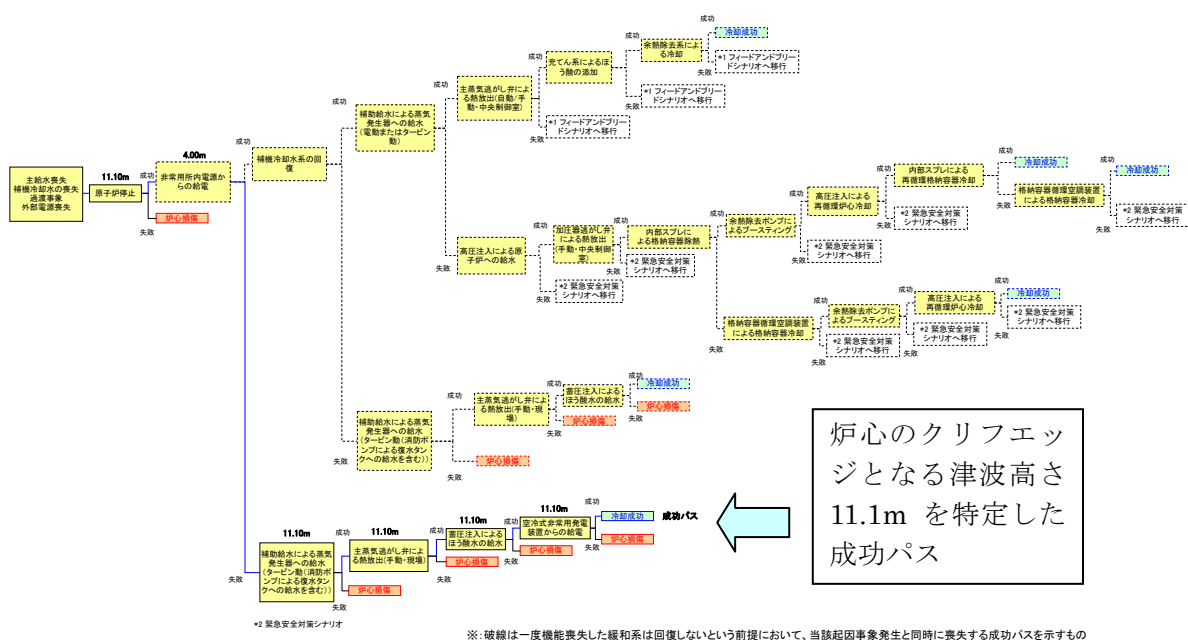
図5-(6)-2 津波時においてクリフエッジを特定したイベントツリー (炉心)
