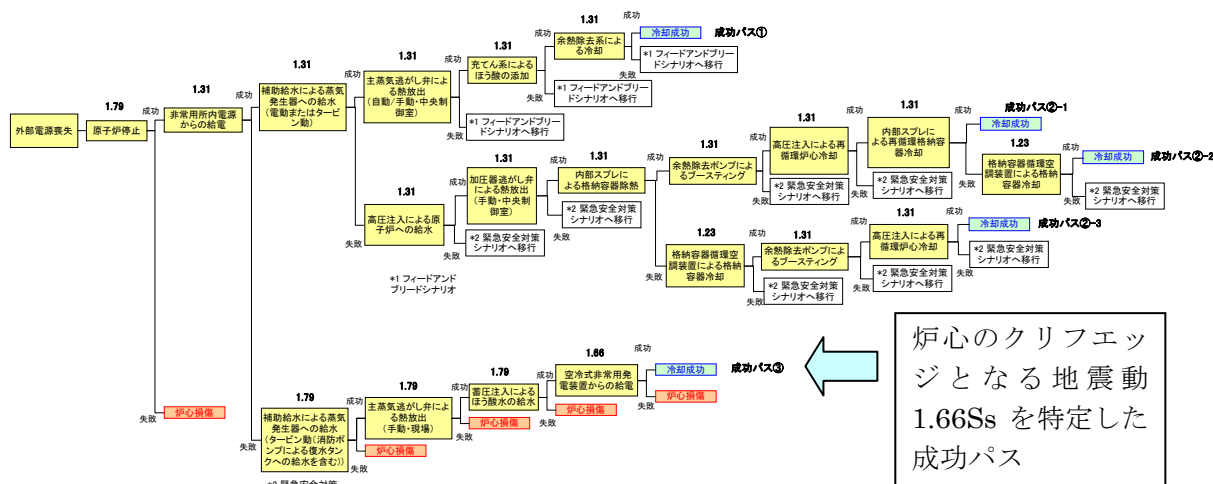
図5-(6)-1 地震時においてクリフエッジを特定したイベントツリー (炉心)
