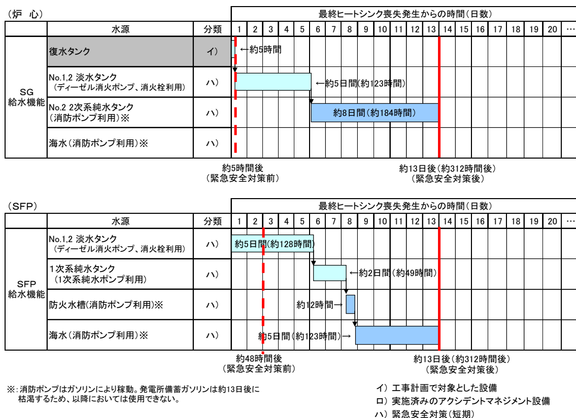
図 5-(5)-7 運転時における事象の過程の進展を防止する措置の効果の評価結果
