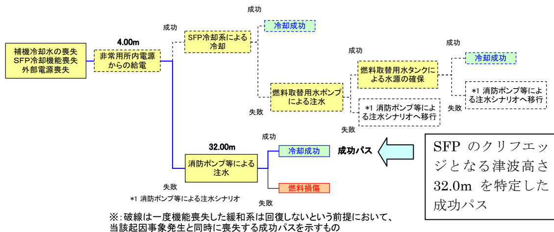
図5-(6)-5 津波時においてクリフエッジを特定したイベントツリー (SFP)
