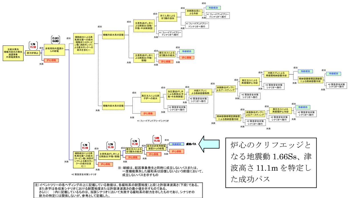
図5-(6)-3 地震・津波の重畳時においてクリフエッジを特定したイベントツリー (炉心)
