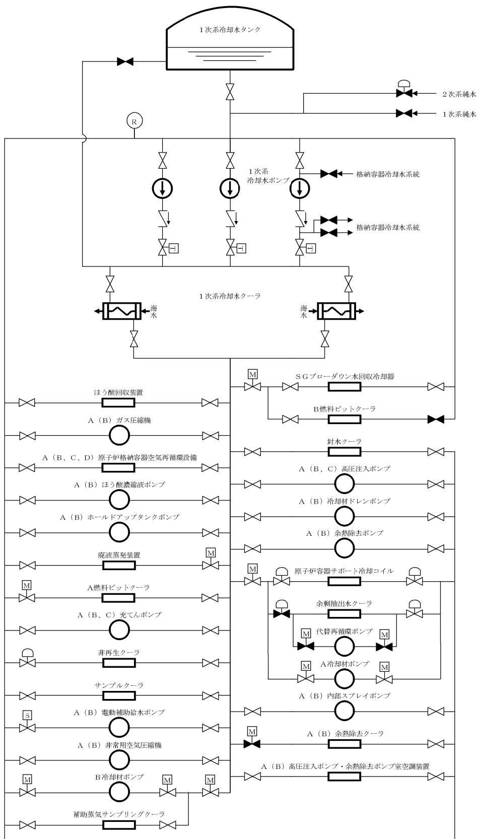
美浜発電所 1 号機の系統構成 (1 次系冷却水系)
