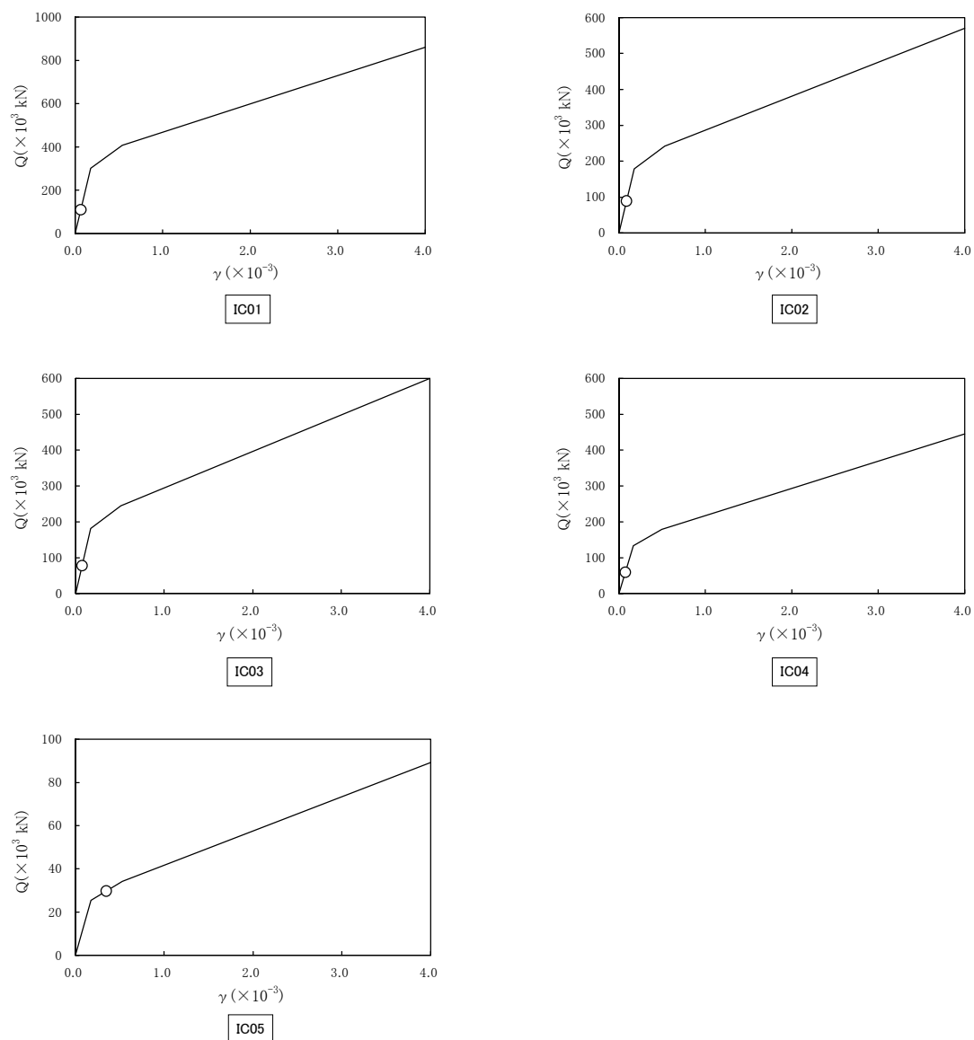
図 2-7-4 Q- \gamma 関係と最大応答値 (原子炉建屋 I/C S 8-1 NS 方向)
