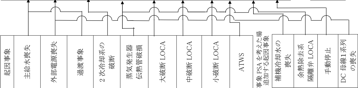
内的事象 PSA における起回事象 (美浜 1 号機 PSR 報告書より)
