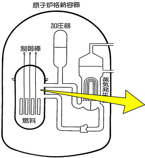
系統概要図
