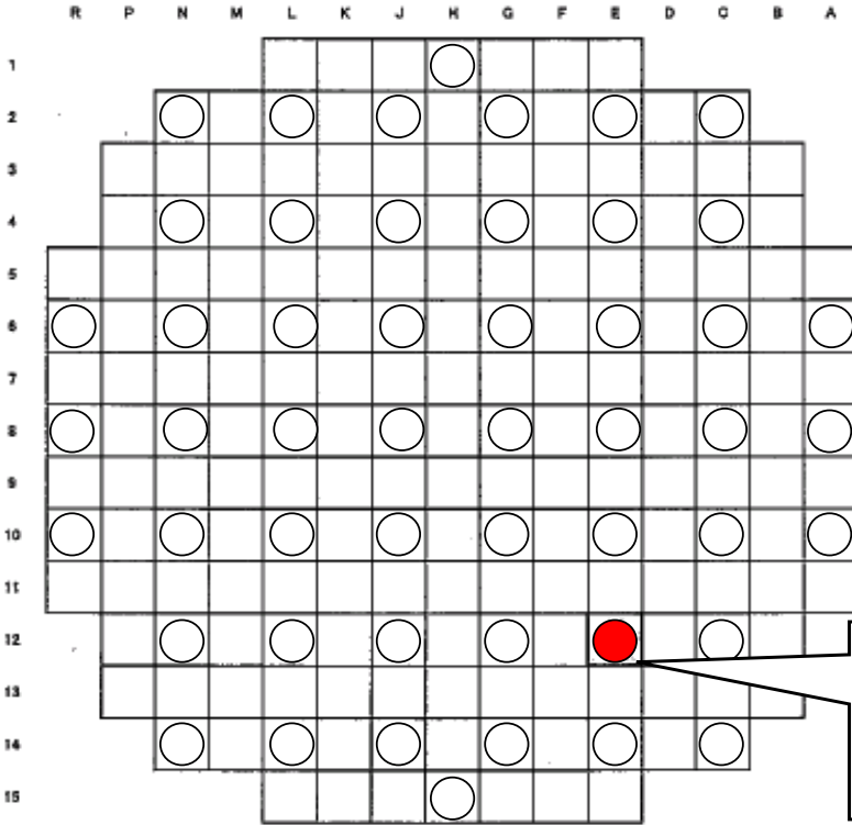
炉内計装配置図
