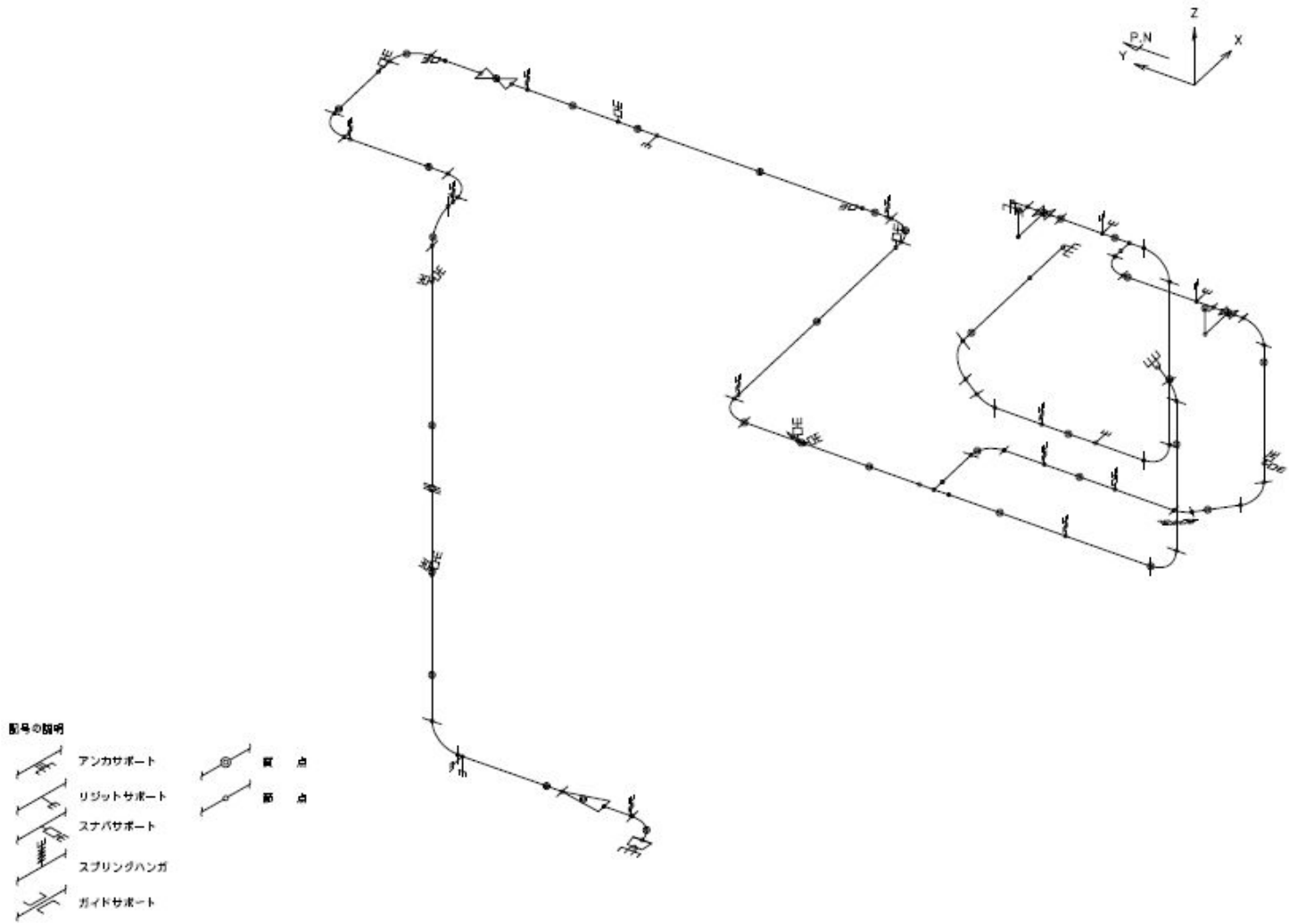
図 3 - 6 地震応答解析モデル（配管系の例）
