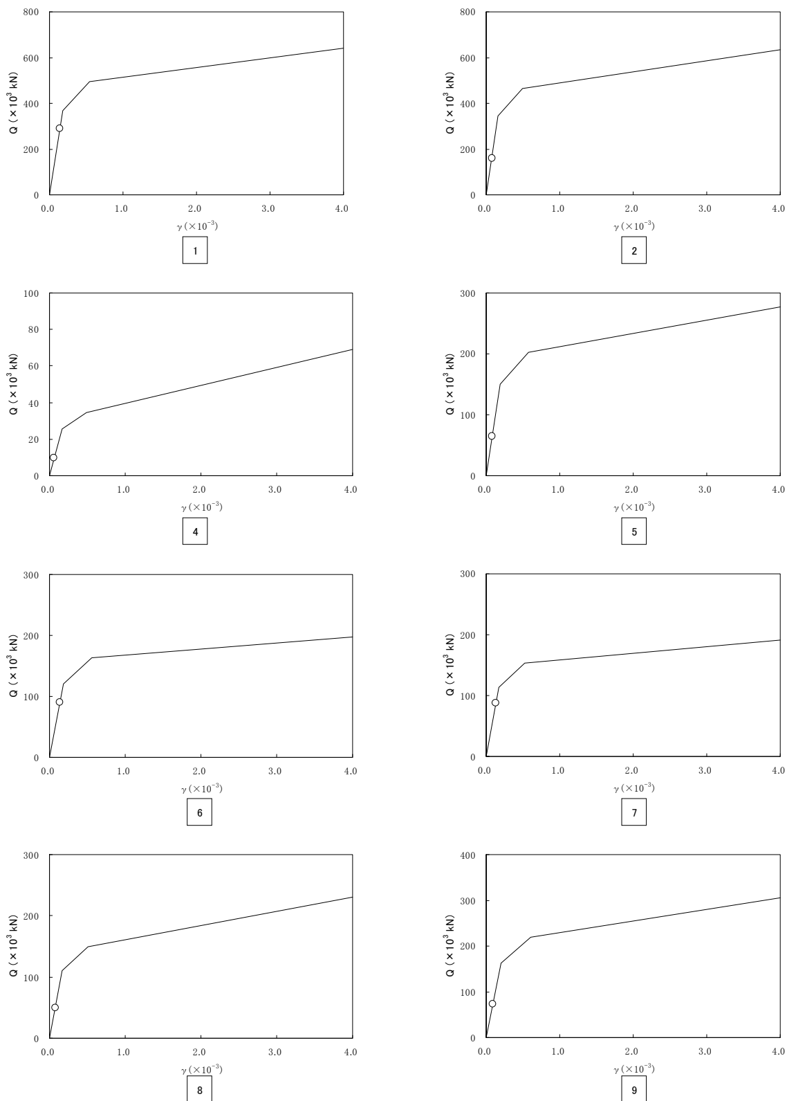
図 2 - 5 - 5 Q- \gamma 関係と最大応答値 (原子炉補助建屋 S_s EW 方向)
