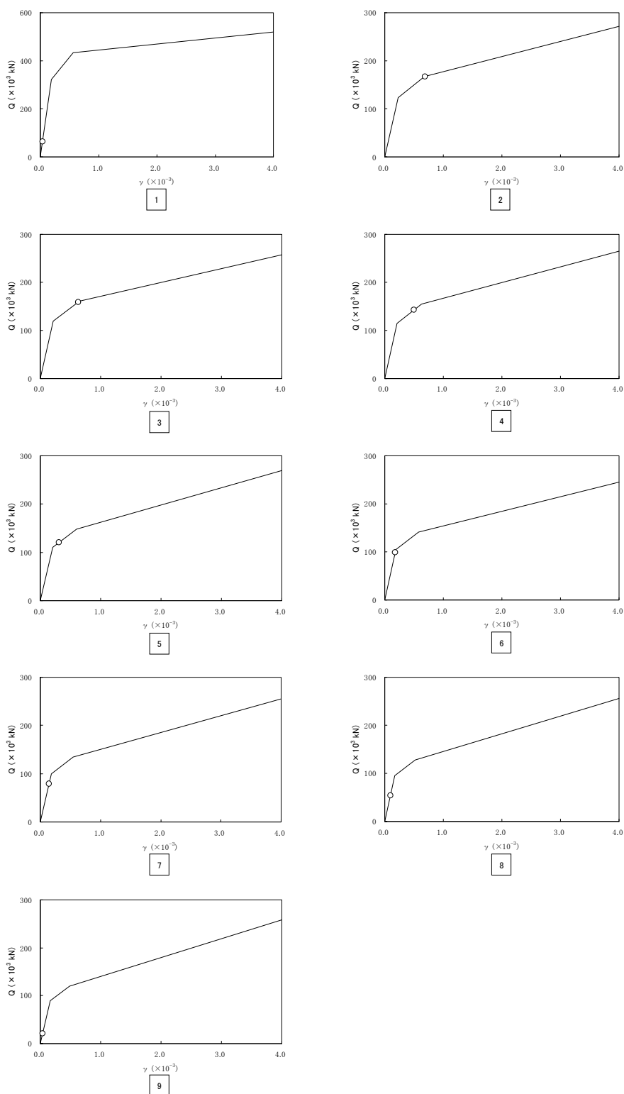
図 2-5-3 Q- \gamma 関係と最大応答値 (原子炉建屋 0/S S s NS 方向)
