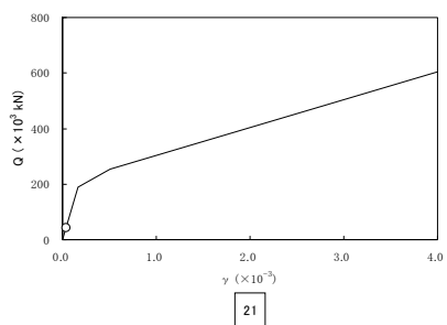
図 2-5-4 Q- \gamma 関係と最大応答値 (原子炉建屋 I/C S s NS 方向)
