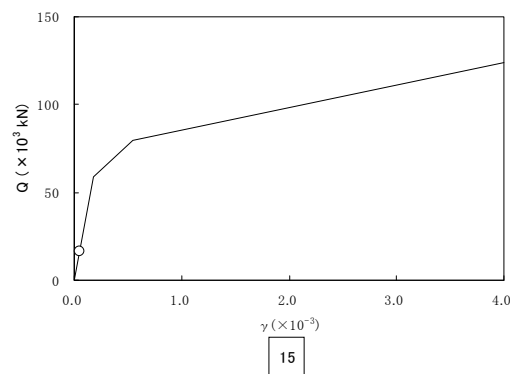
図 2 - 5 - 8 Q- \gamma 関係と最大応答値 (原子炉補助建屋 S_s NS 方向)
