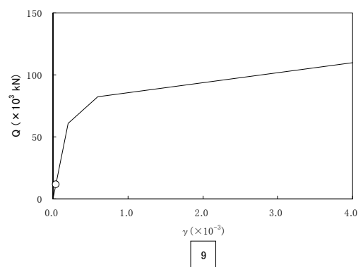
図 2 - 5 - 7 Q- \gamma 関係と最大応答値 (原子炉補助建屋 S s NS 方向)
