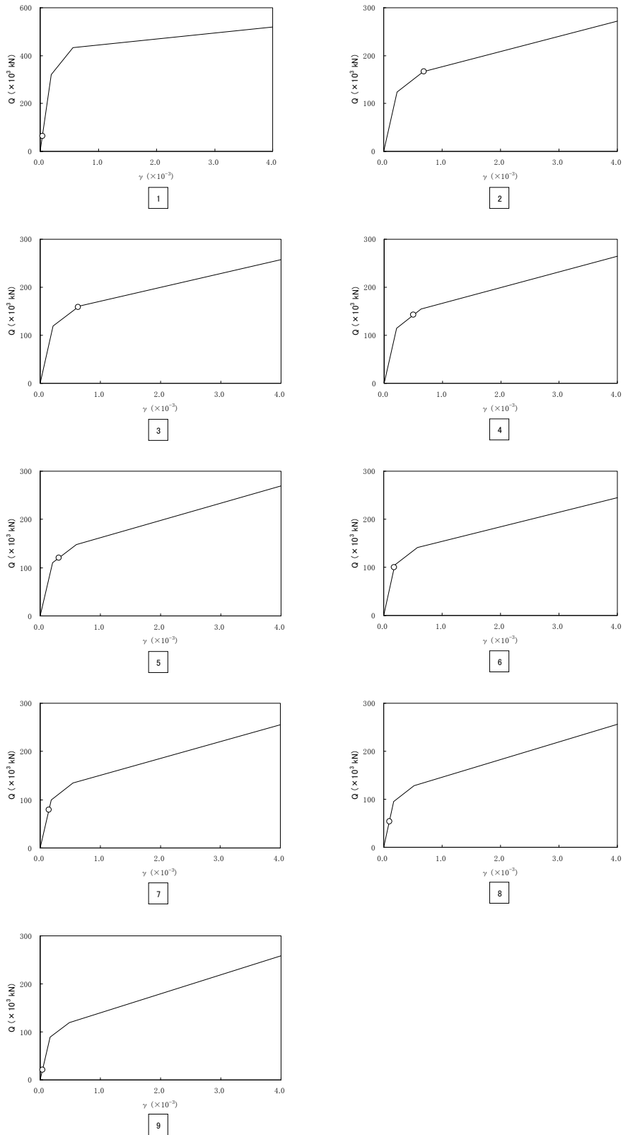
図 2 - 5 - 1 Q- \gamma 関係と最大応答値 (原子炉建屋 0/S S s EW 方向)
