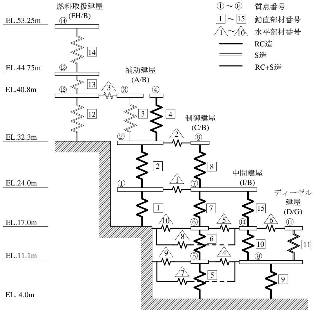
図 2 - 4 原子炉補助建屋の解析モデル(鉛直)
