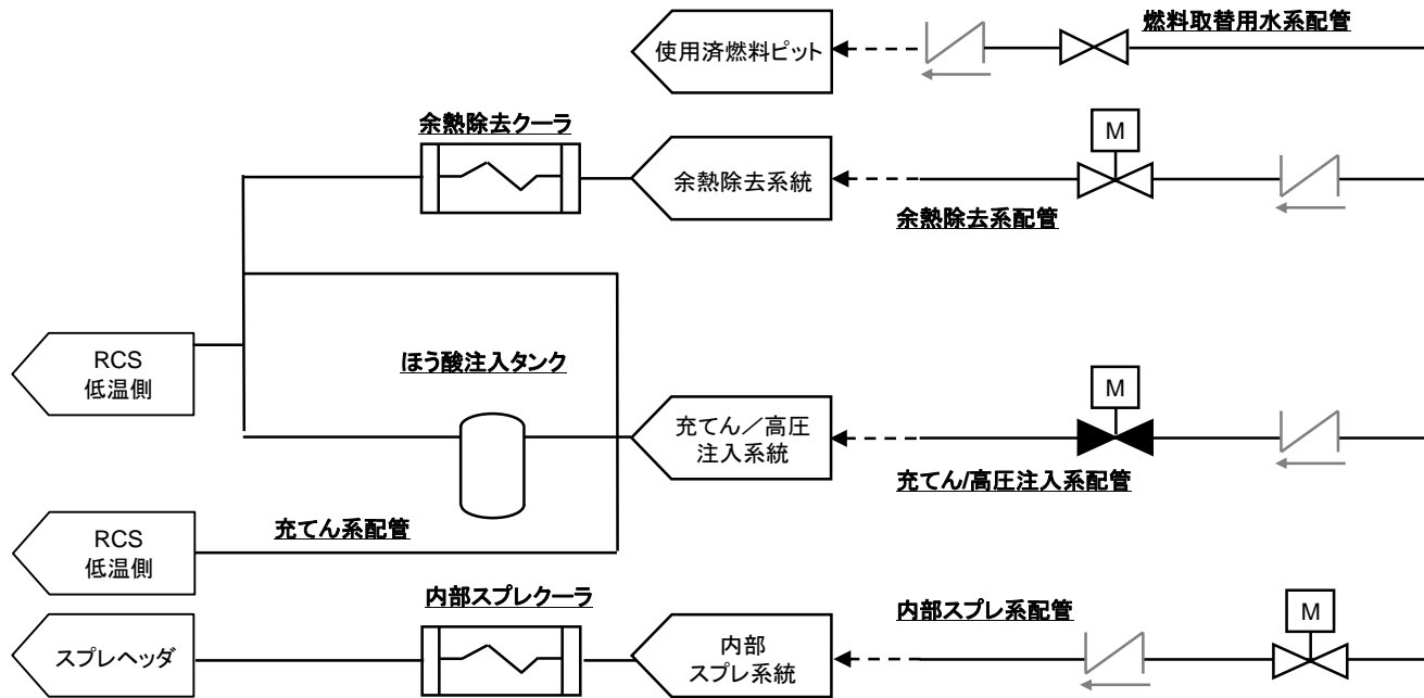
各影響緩和機能の系統図(地震: 炉心損傷)
