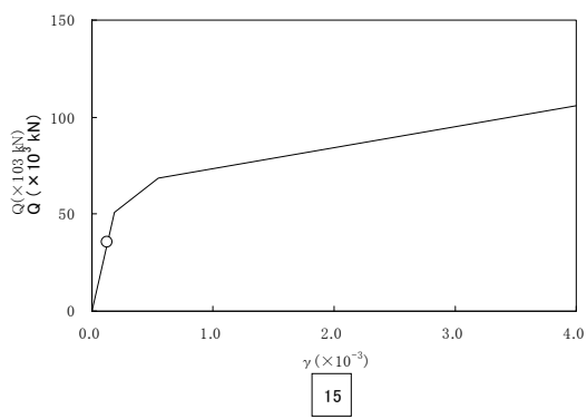
図 2 - 5 - 6 Q- \gamma 関係と最大応答値 (原子炉補助建屋 S_s EW 方向)
