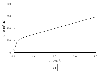
図 2-5-2 Q- \gamma 関係と最大応答値 (原子炉建屋 I/C S s EW 方向)
