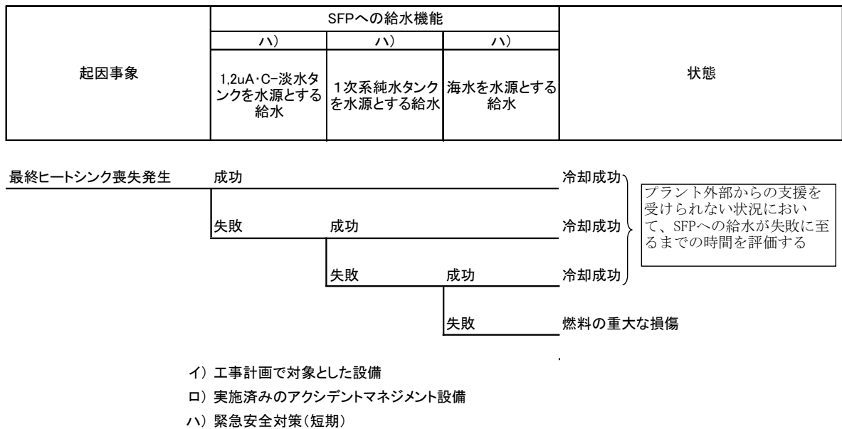
図 5-(5)-2 最終ヒートシンク喪失から燃料の重大な損傷に至る事象の過程 (SFP)
