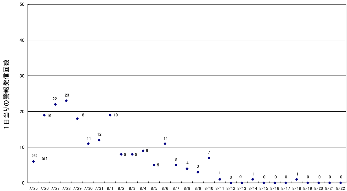
大飯4号機 「1次冷却材飽和温度注意」警報発信回数の推移
