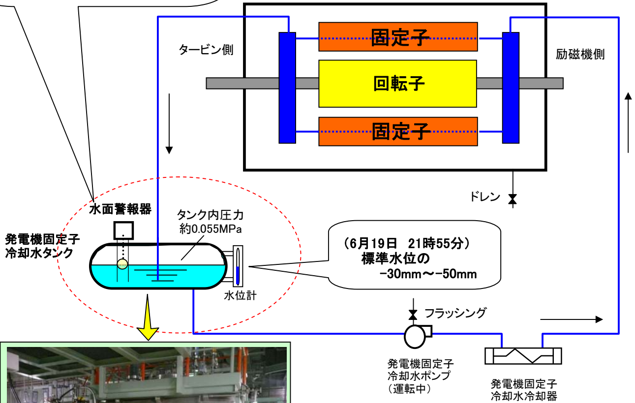
発電機固定子冷却水タンク 容量: 3.87m 3
