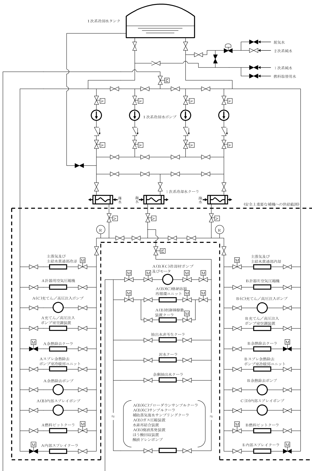
美浜発電所 3号機の系統構成 (1次系冷却水系)
