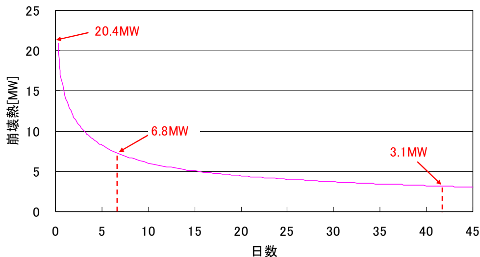
図 1 崩壊熱の変化
